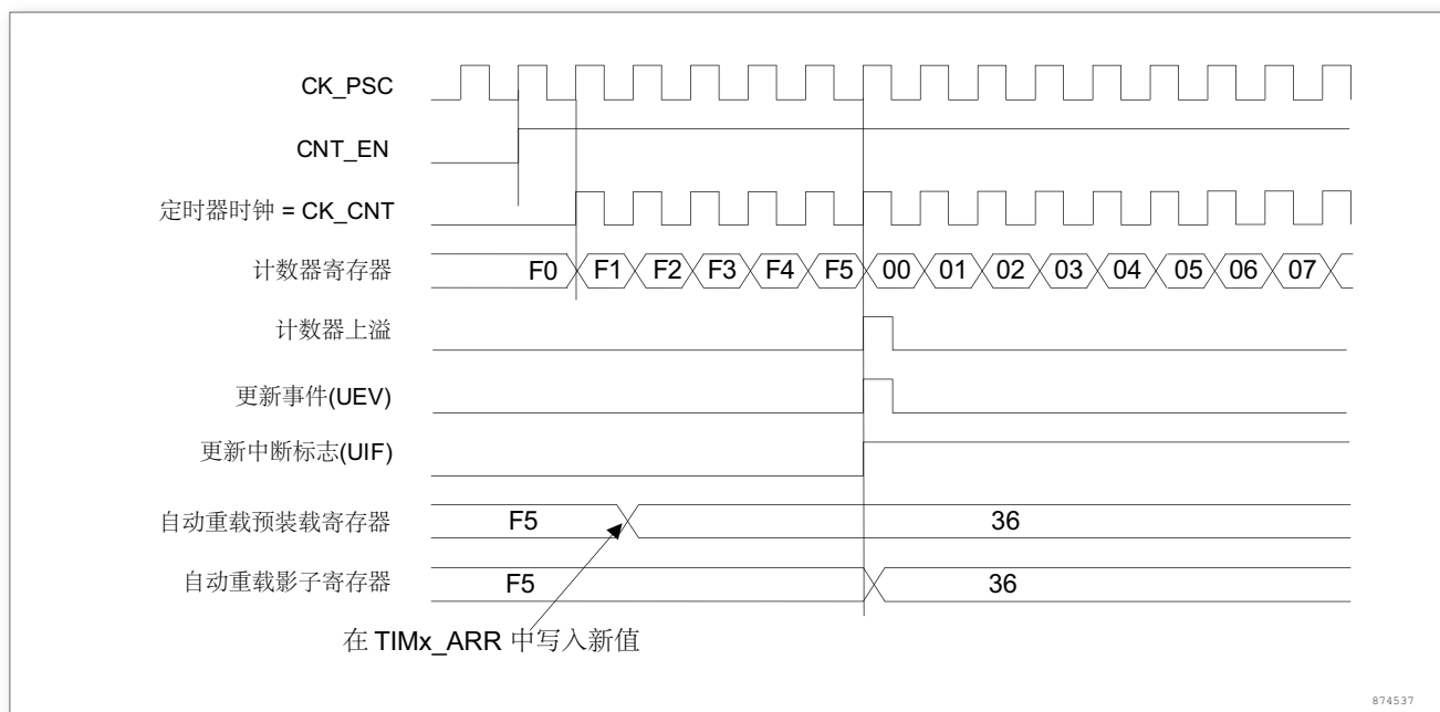
图 132. 计数器时序图，当 ARPE = 1 时的更新事件 (预装入了 TIMx_ARR)
