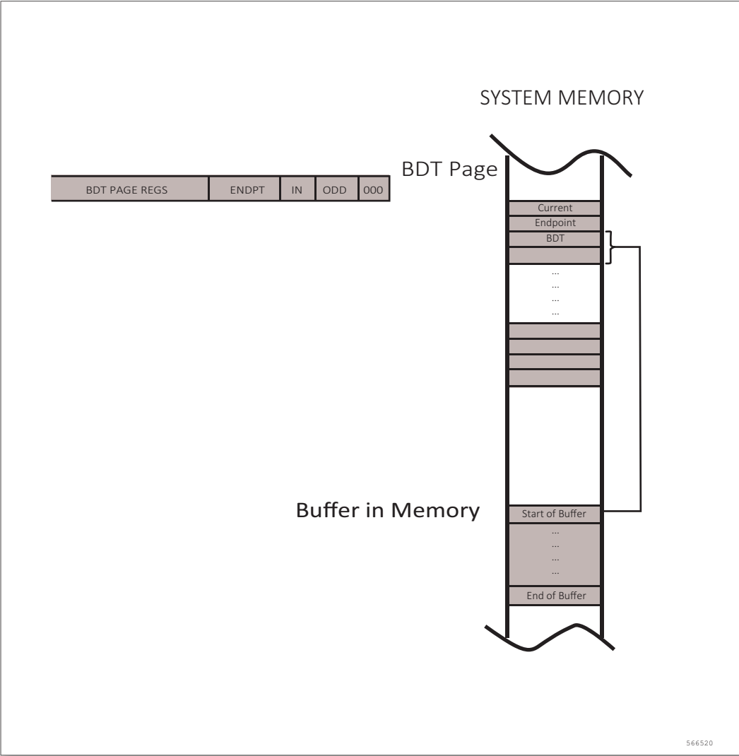
图 187. 缓冲区描述符表
