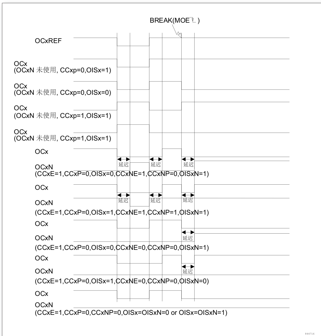
图 67. 响应刹车的输出
