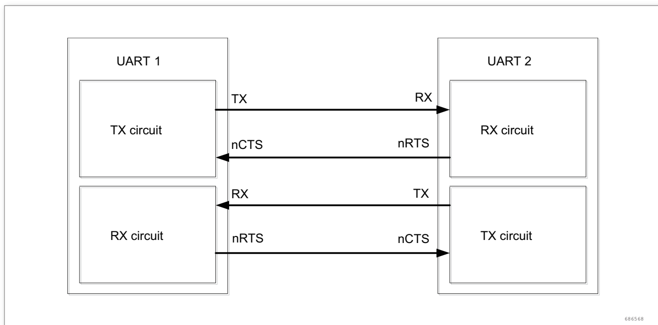
图 224. 两个 UART 间的硬件流控制
