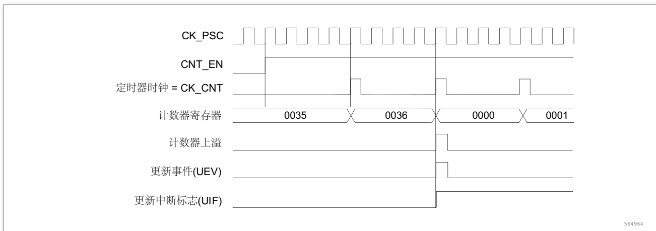
图 129. 计数器时序图，内部时钟分频因子为 4
