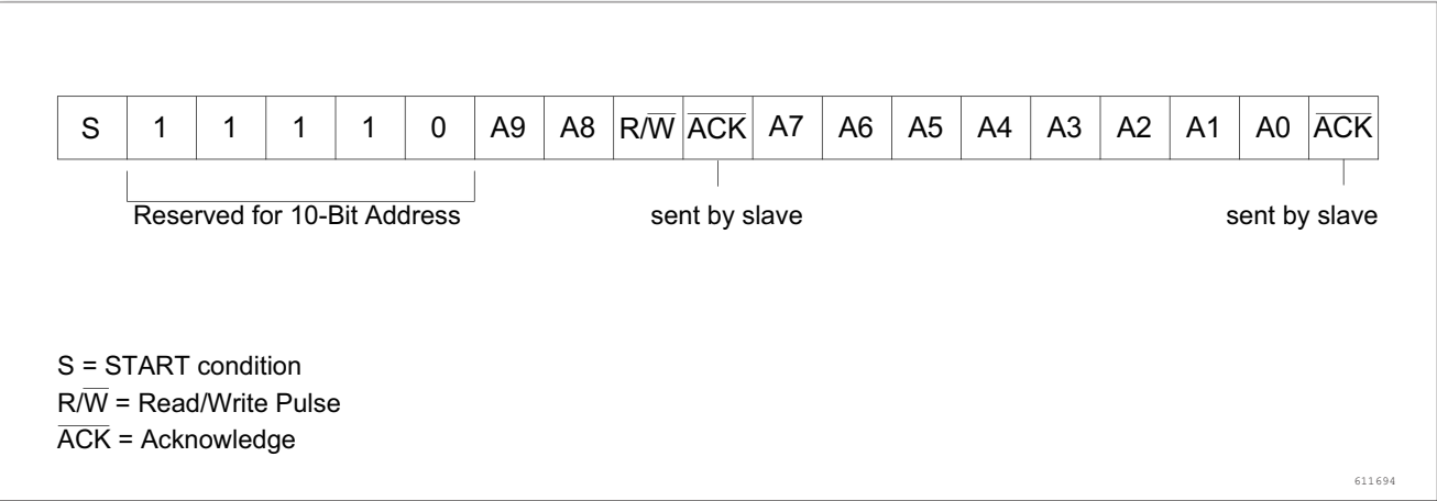
图 206. 10 位的地址格式
