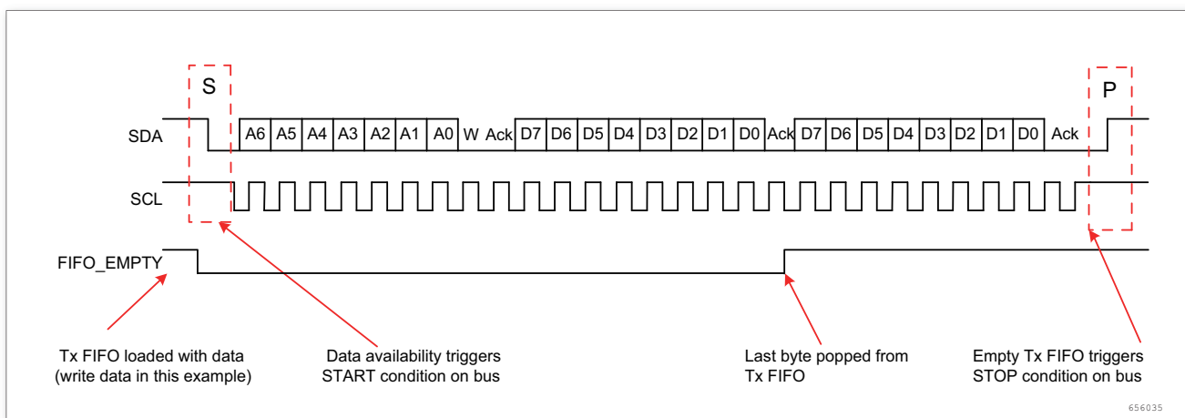
图 211. 主发送 - Tx FIFO 为空
