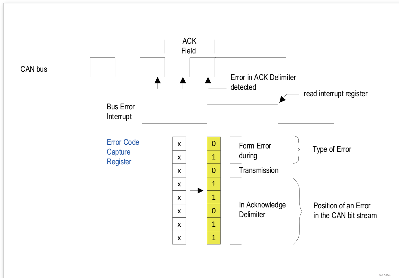
图 199. 错误码捕捉功能举例
