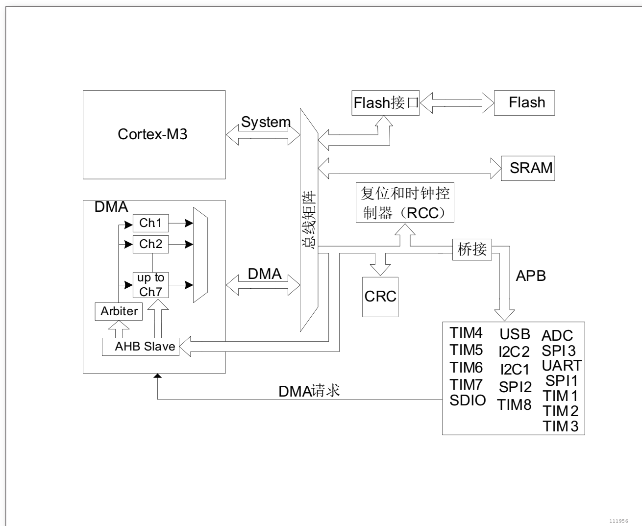
图 21. DMA 框图
