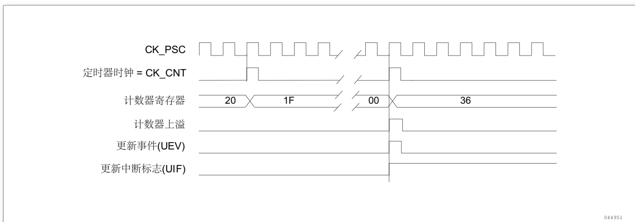
图 42. 计数器时序图，内部时钟分频因子为 N
