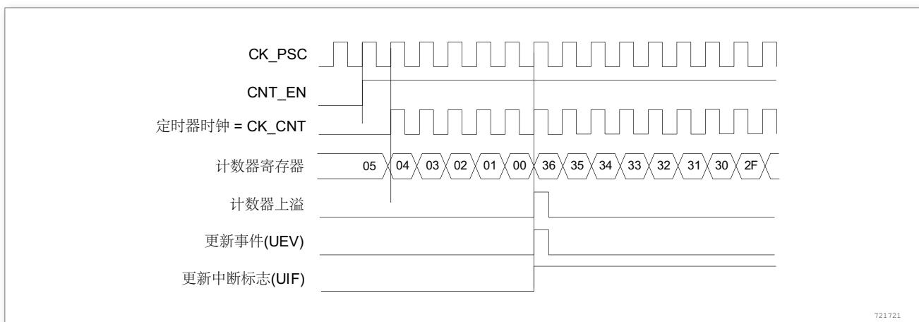
图 87. 计数器时序图，内部时钟分频因子为 1
