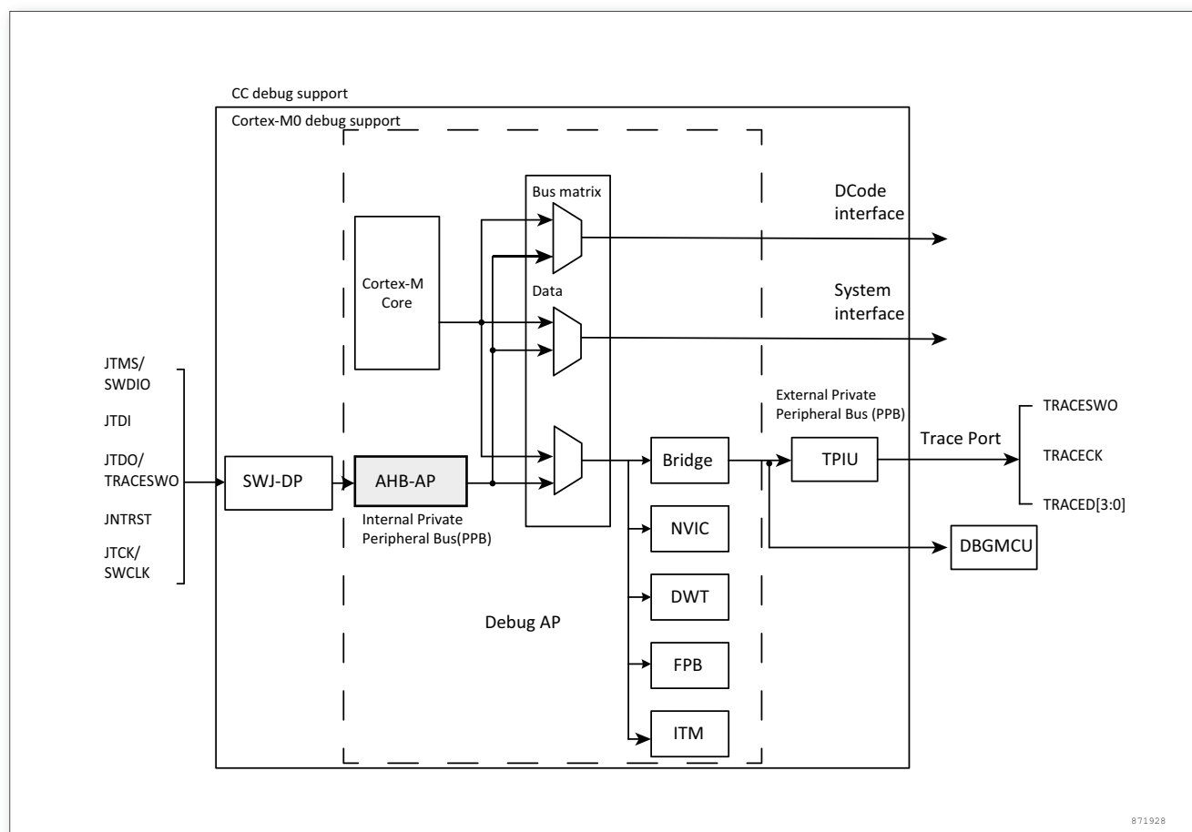
图 227. MM32 系列级别和 CPU 级别的调试框
