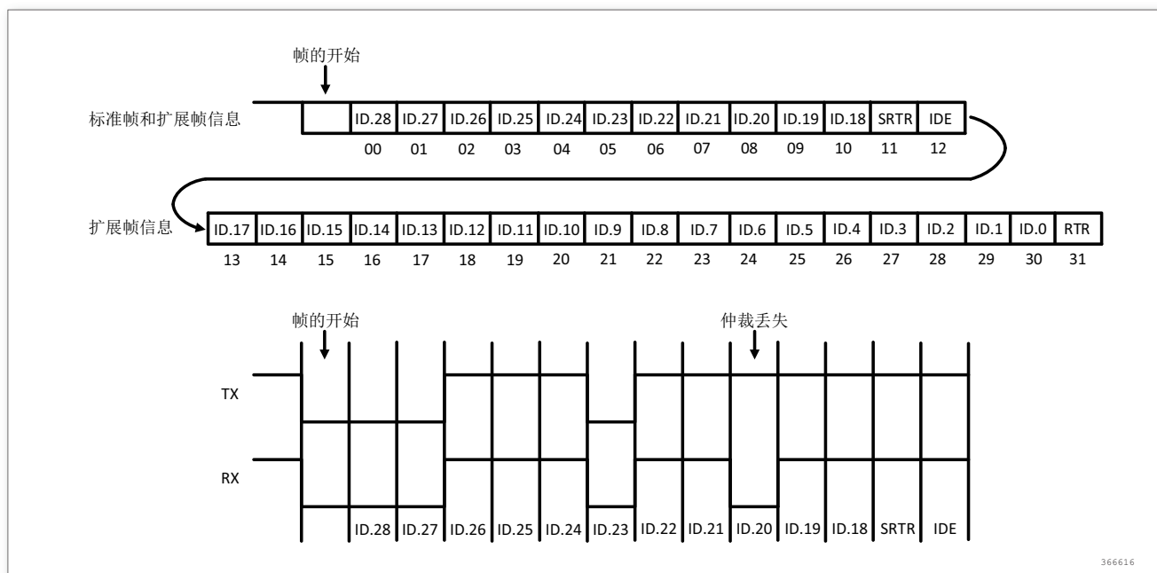
图 200. 仲裁丢失解释举例
