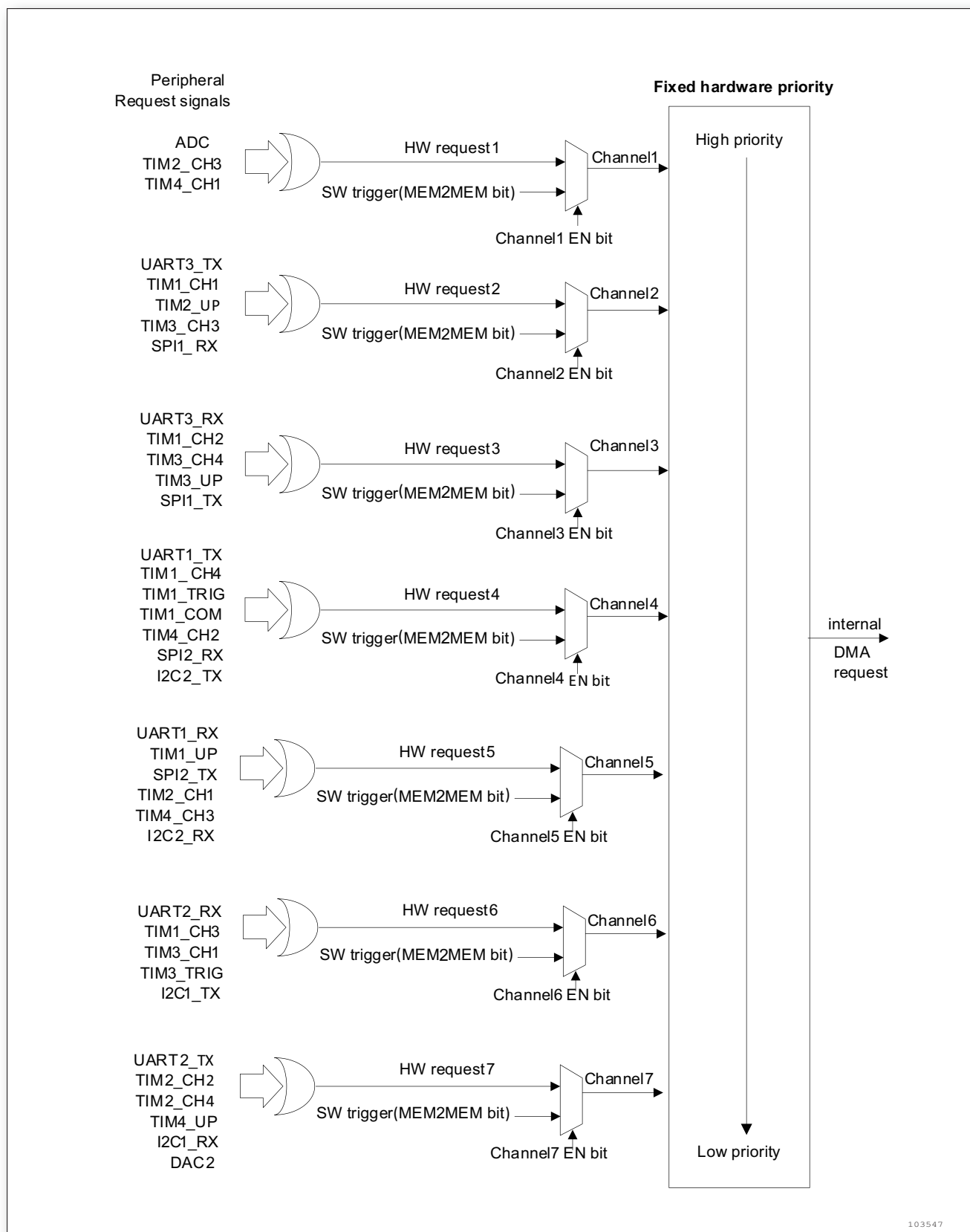
图 22. 外设 DMA1 请求映射
