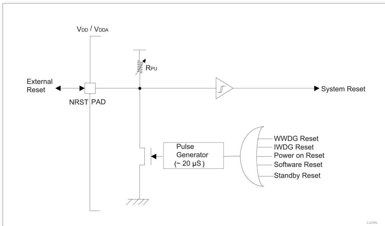
图 11. 复位电路
