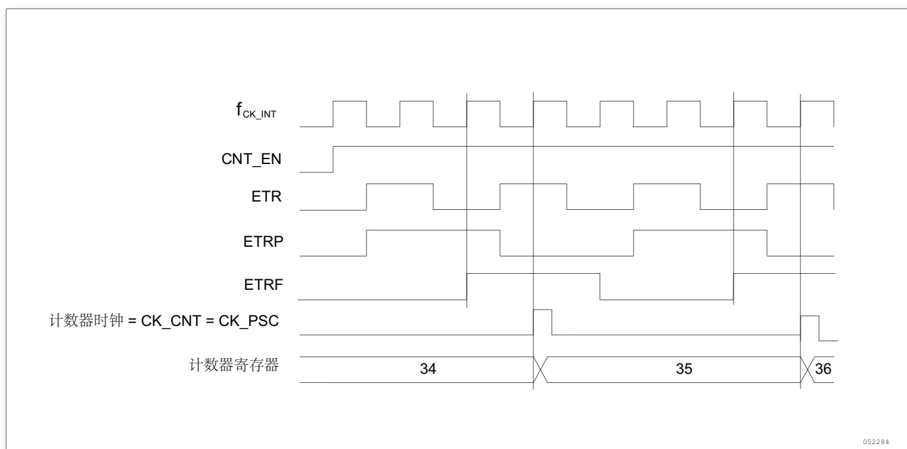
图 148. 外部时钟模式 2 下的控制电路
