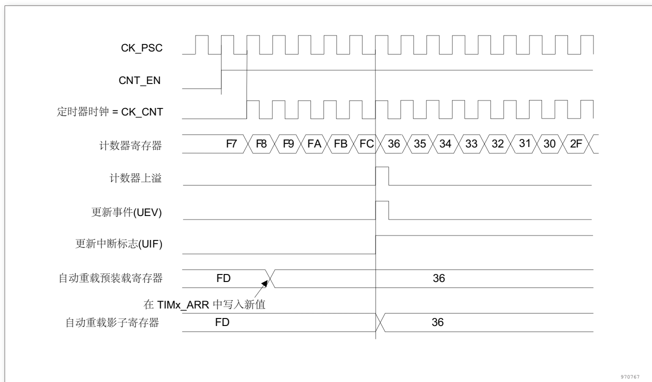
图 143. 计数器时序图, ARPE = 1 时的更新事件 (计数器溢出)
