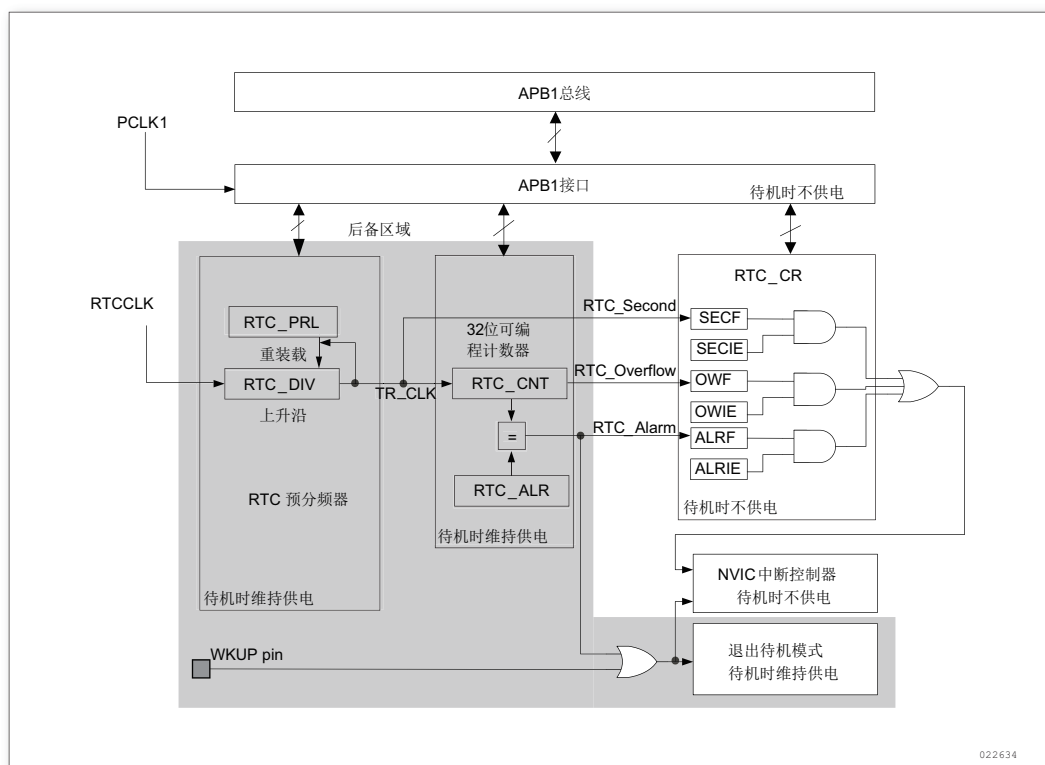
图 180. 实时时钟方框图
