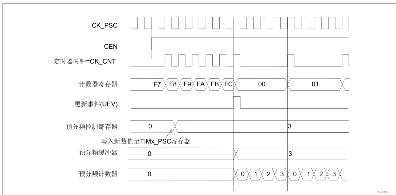
图 126. 当预分频器的参数从 1 变到 4 时，计数器的时序图
