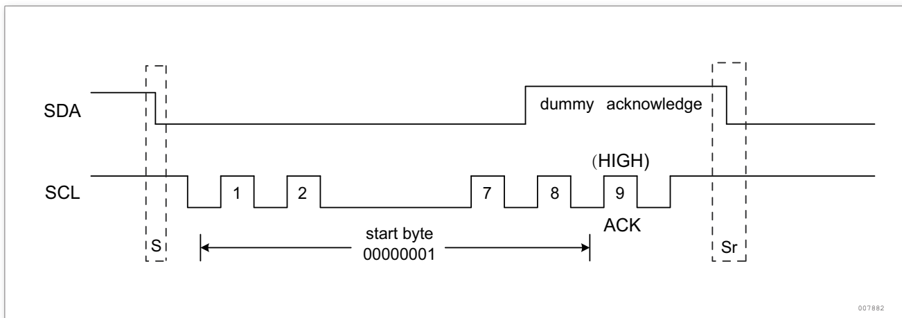
图 209. 起始字节传输
