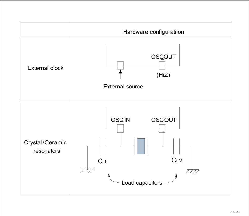
图 13. 时钟源
