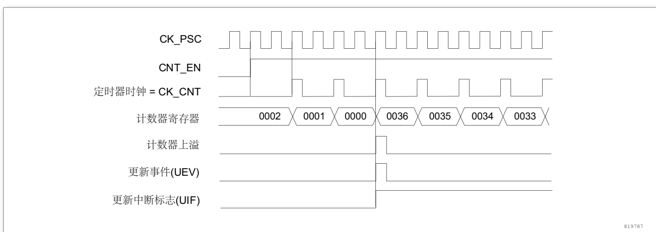
图 88. 计数器时序图，内部时钟分频因子为 2
