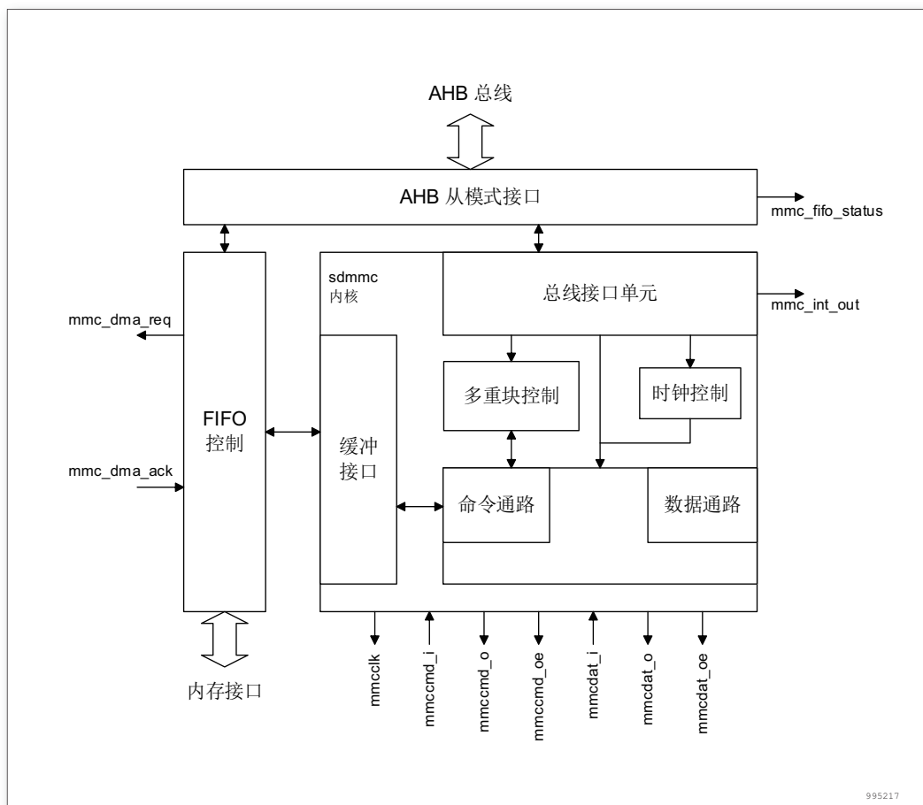
图 233. SDIO 框图
