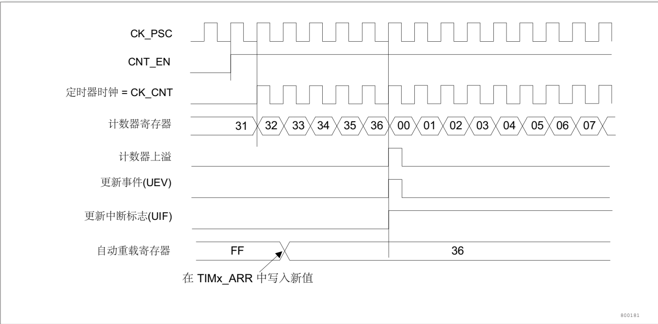
图 37. 计数器时序图，当 ARPE = 0 时的更新事件 (TIMx_ARR 没有预装入)
