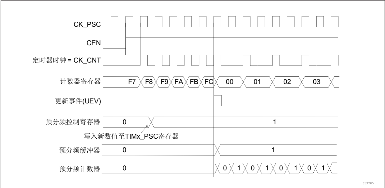
图 125. 当预分频器的参数从 1 变到 2 时，计数器的时序图
