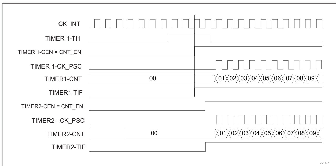
图 169. 使用定时器 1 的 TI1 输入触发定时器 1 和定时器 2
