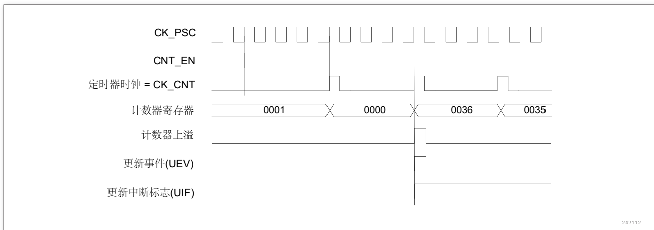
图 41. 计数器时序图，内部时钟分频因子为 4
