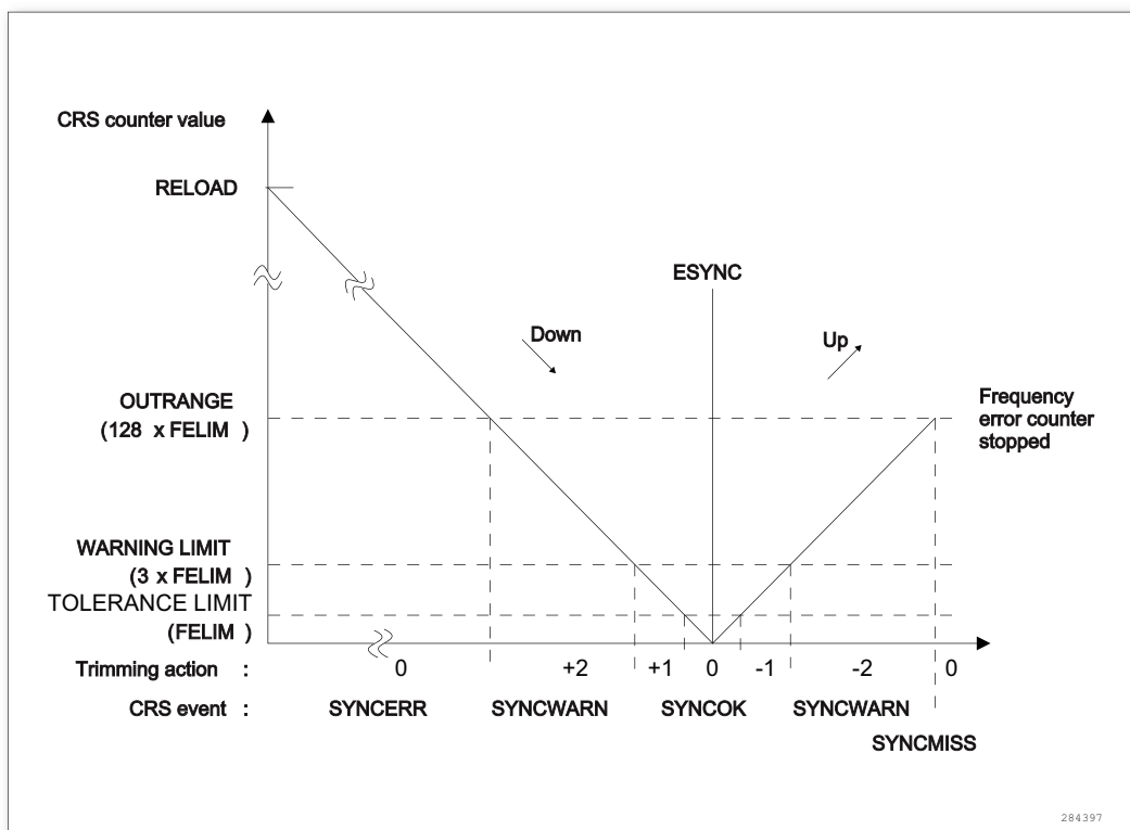
图 231. CRS 计数器状态图
