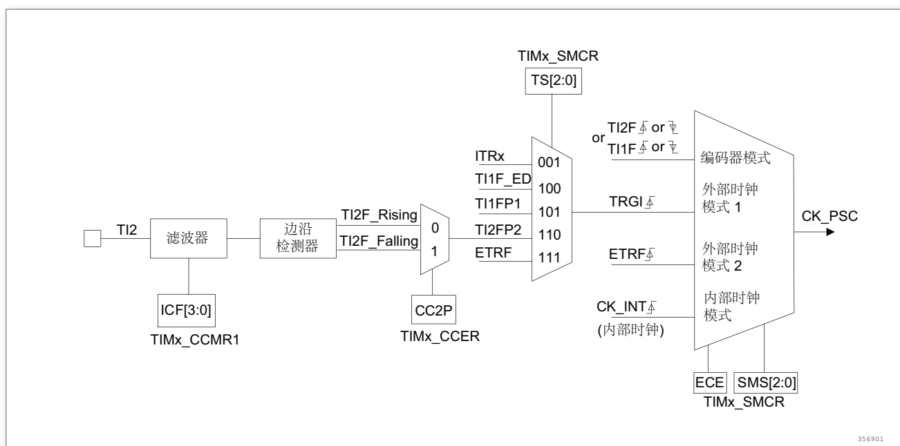
图 145. TI2 外部时钟连接例子
