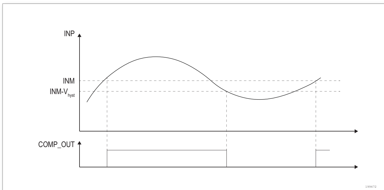
图 29. 比较器的迟滞现象
