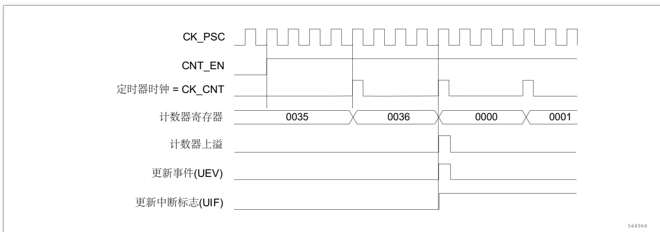
图 83. 计数器时序图，内部时钟分频因子为 4
