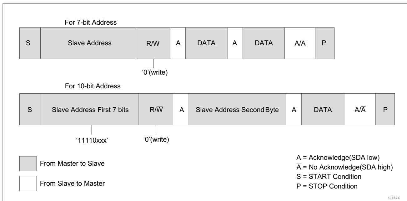
图 207. 主发送协议
