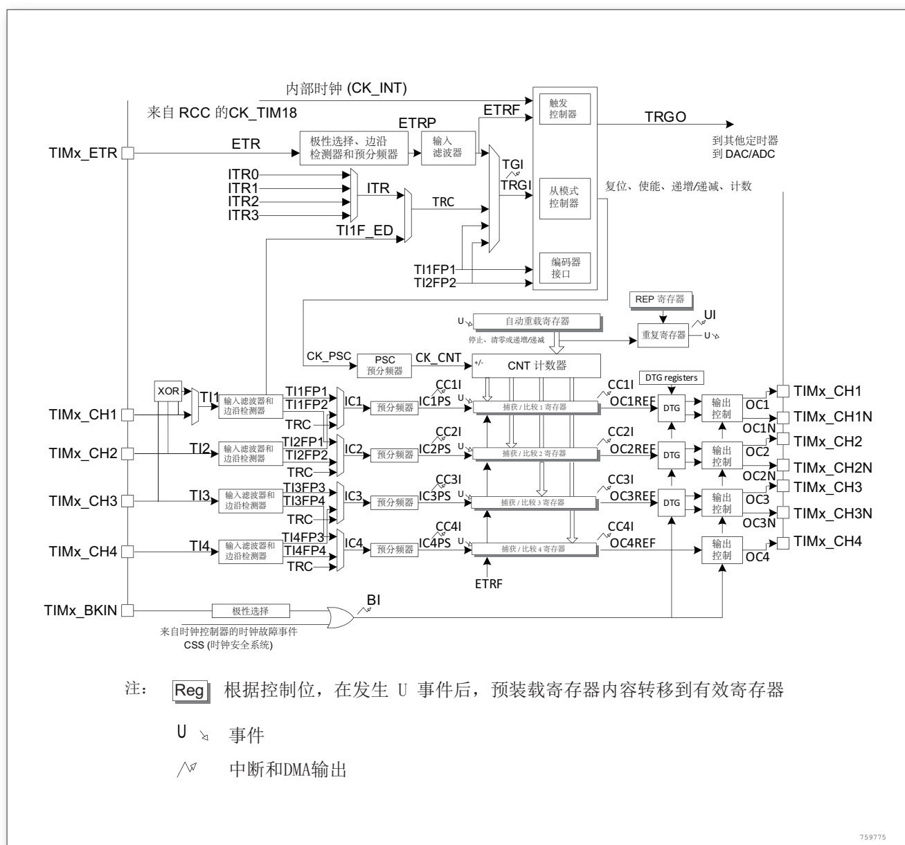
图 30. 高级控制定时器框图
