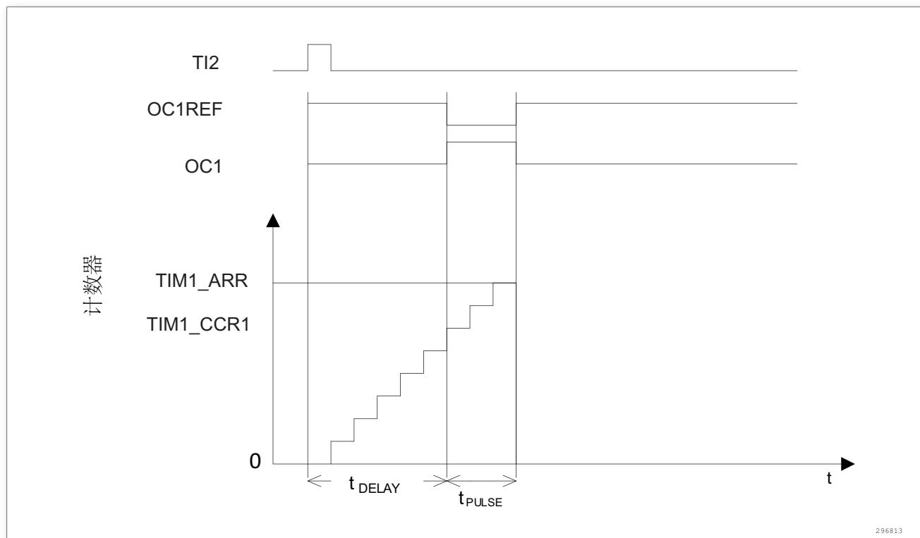
图 156. 单脉冲模式的例子
