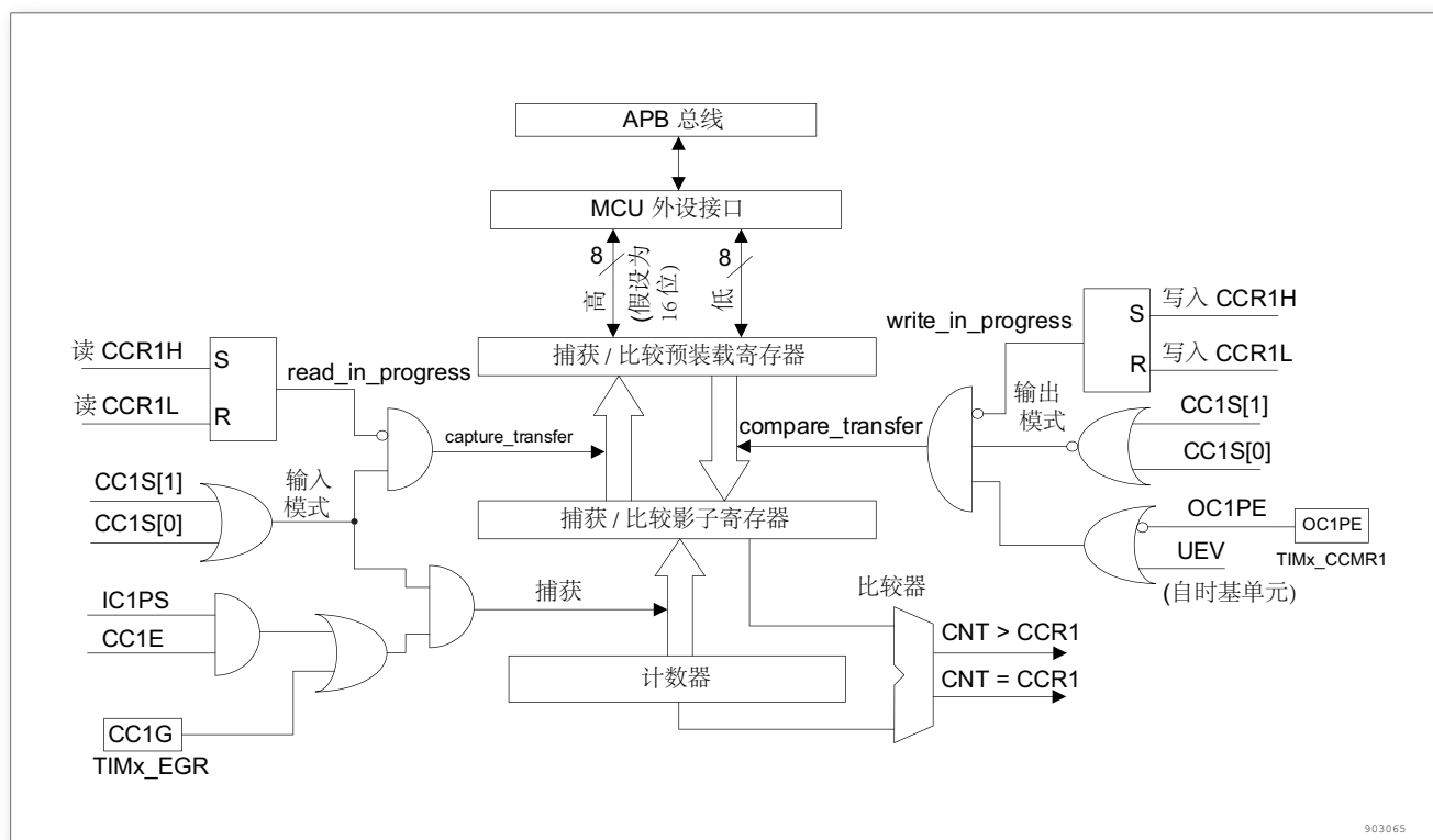
图 104. 捕获/比较通道 1 的主电路
