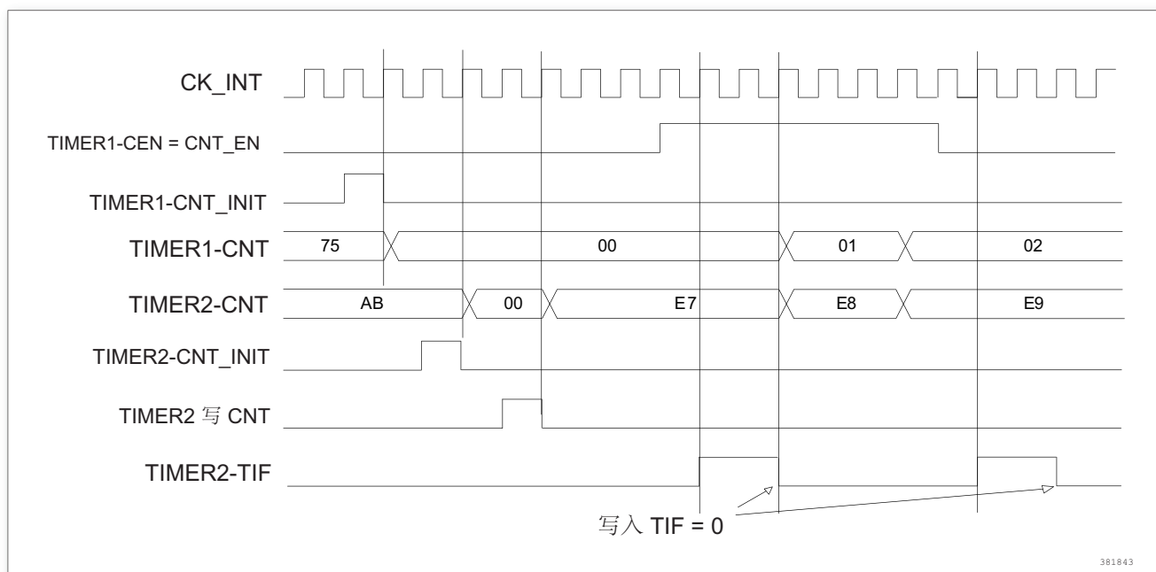
图 166. 通过使能定时器 1 可以控制定时器 2
