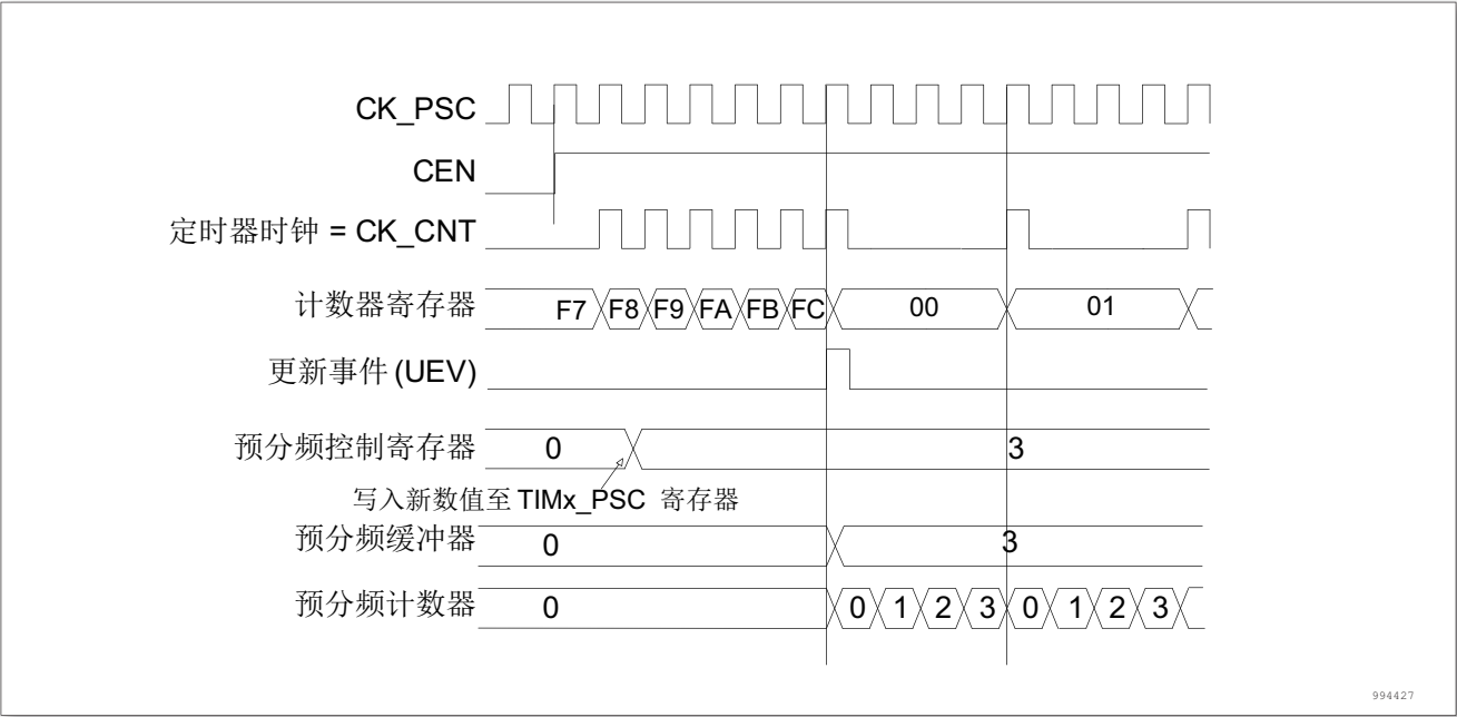
图 172. 当预分频器的参数从 1 变到 4 时，计数器的时序图
