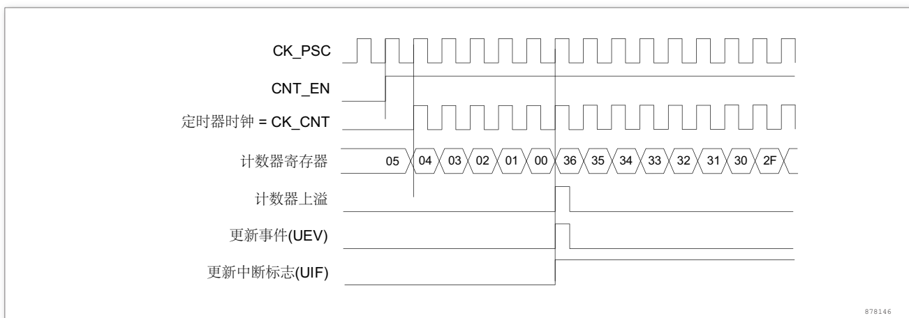
图 39. 计数器时序图，内部时钟分频因子为 1
