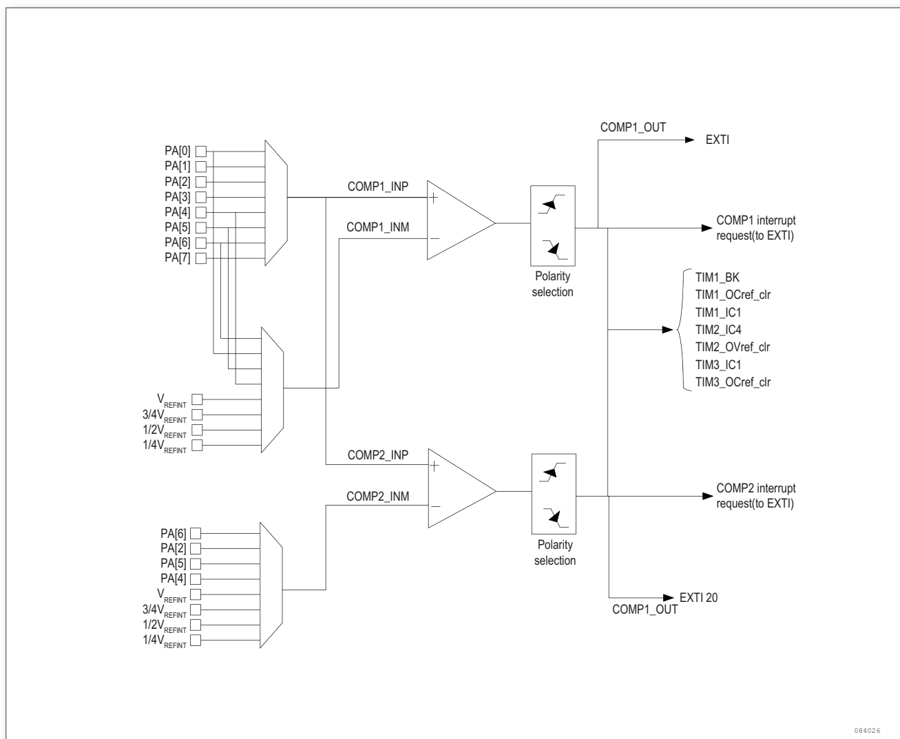
图 28. 比较器框图
