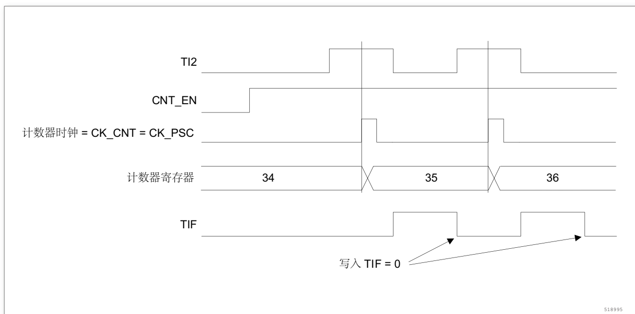
图 146. 外部时钟模式 1 下的控制电路
