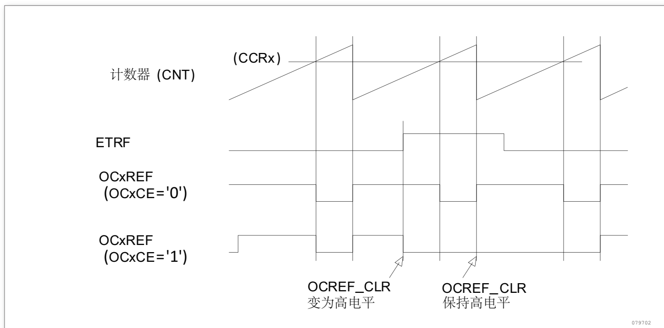
图 157. 清除 TIMx 的 OCxREF
