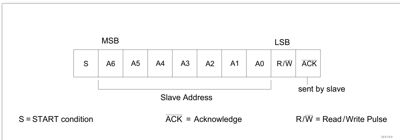
图 205. 7 位的地址格式
