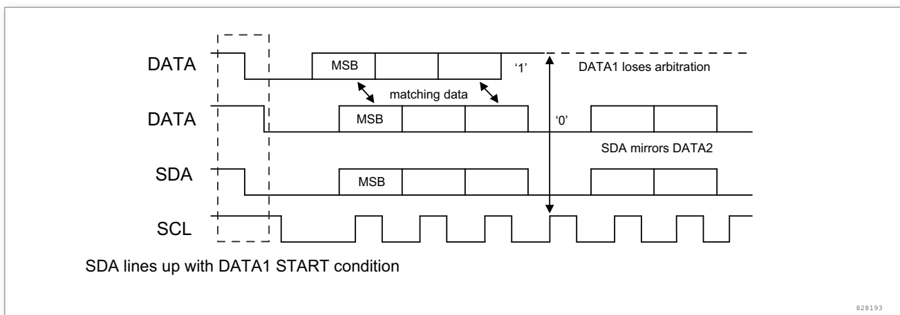
图 213. 多个主机仲裁
