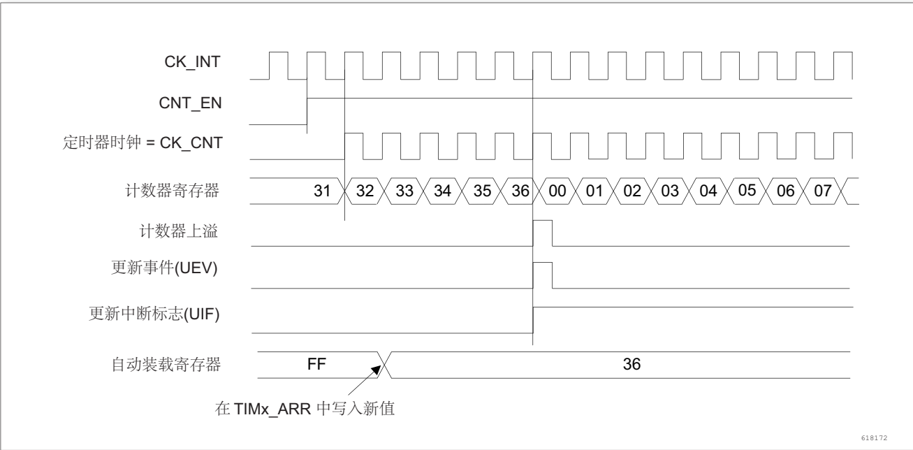
图 177. 计数器时序图，当 ARPE = 0 时的更新事件 (TIMx_ARR 没有预装载)
