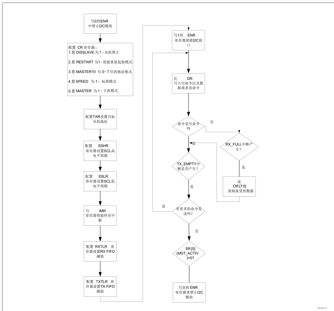
图 216. I2C 接口主机流程图
