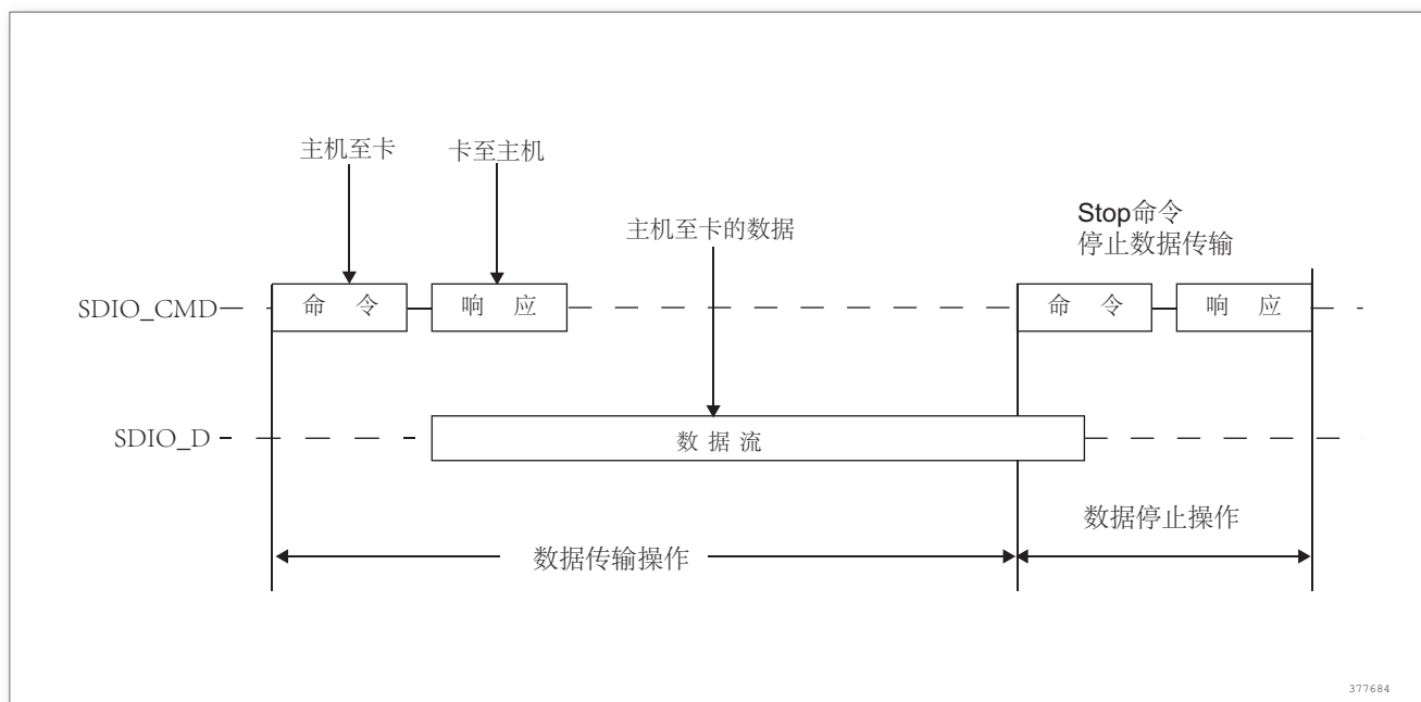
图 238. SDIO 连续写操作
