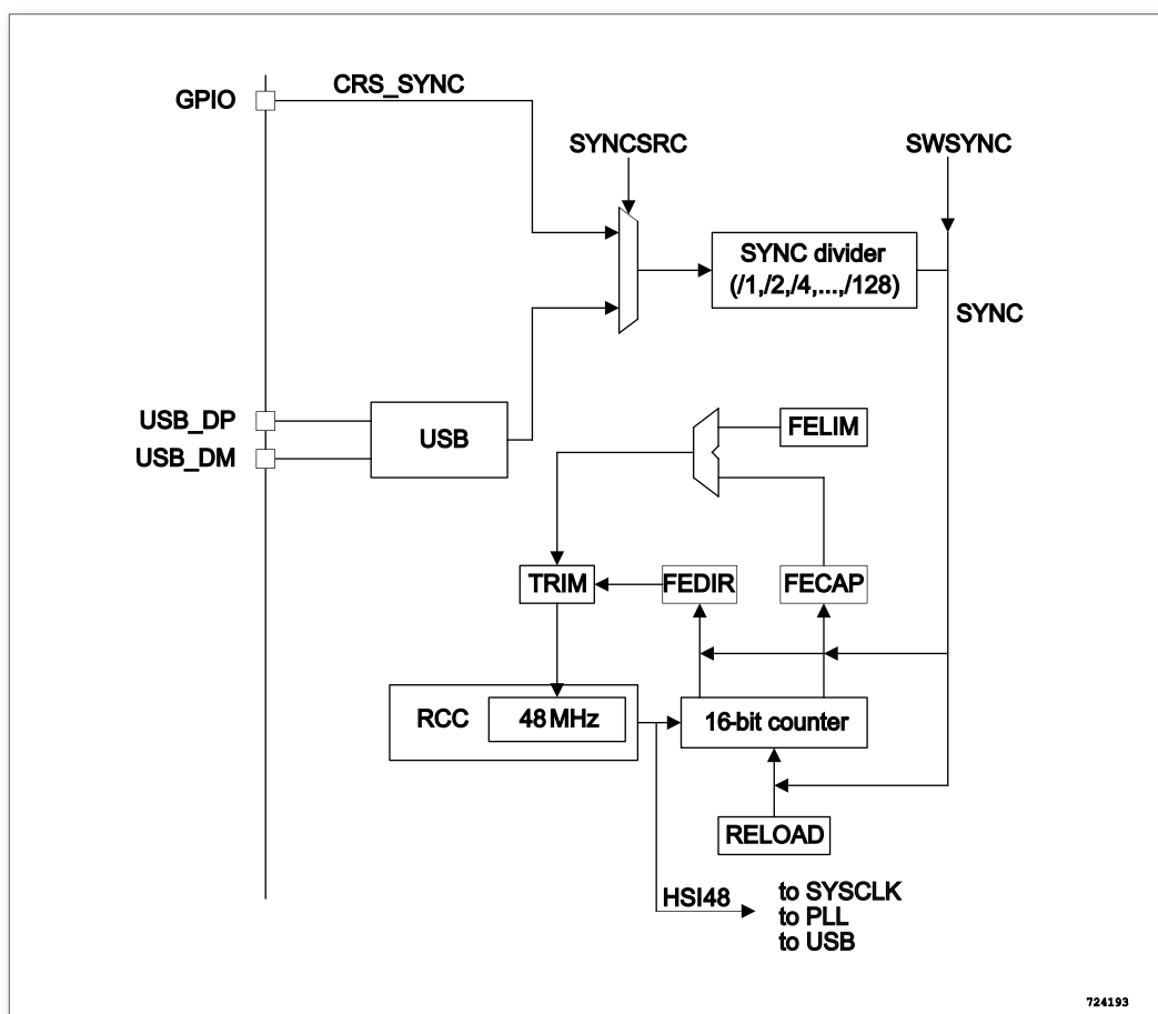
图 230. CRS 框图架构
