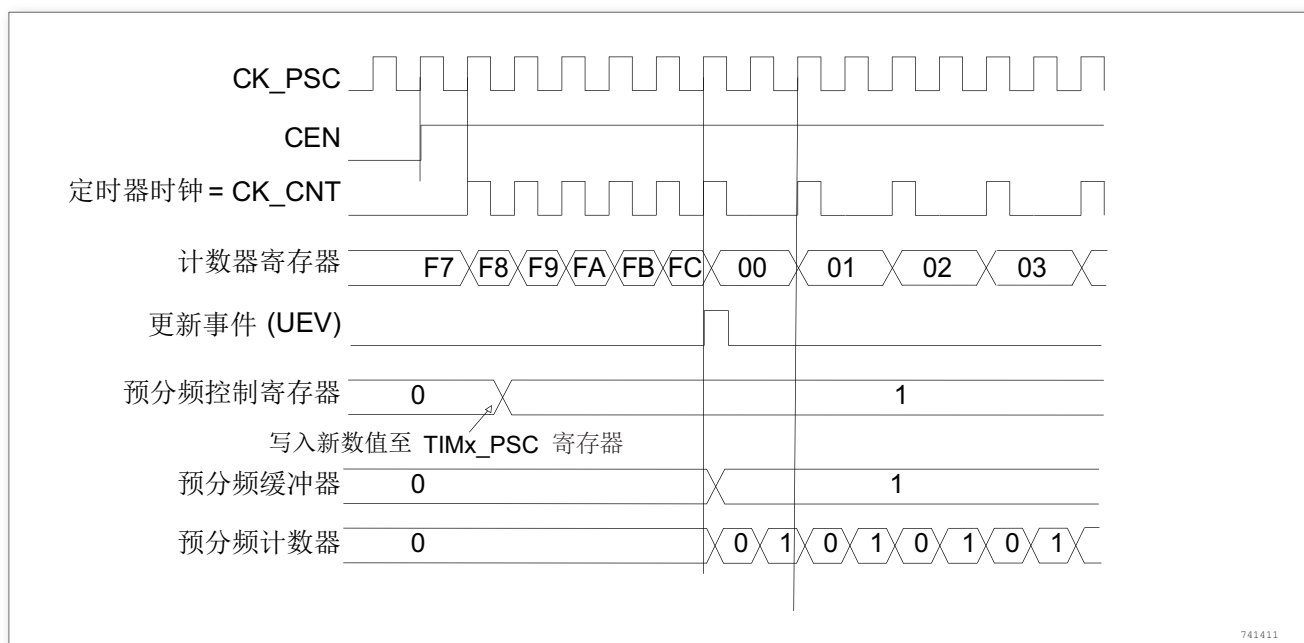
图 171. 当预分频器的参数从 1 变到 2 时，计数器的时序图
