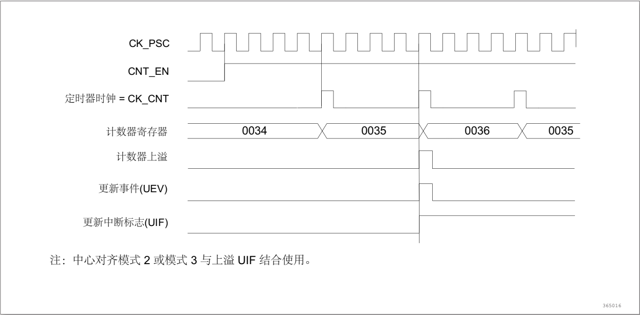
图 46. 计数器时序图，内部时钟分频因子为 4，TIMx_ARR = 0x36
