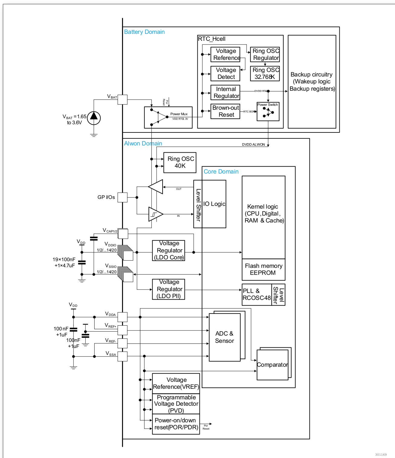
图 8. 电源框图
