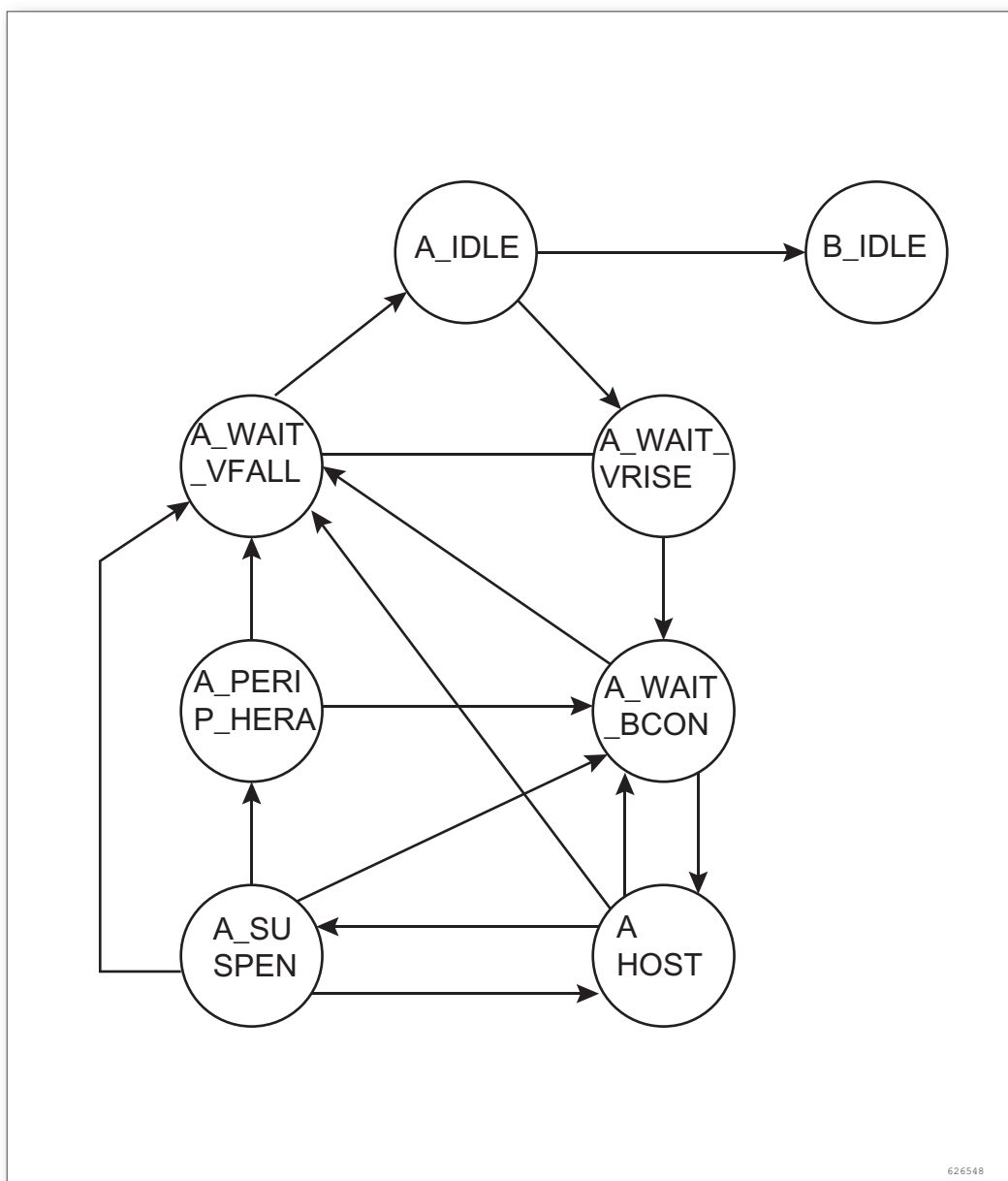
图 189. OTG 双角色 A 设备操作方式
