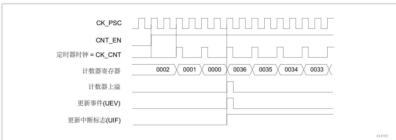
图 134. 计数器时序图，内部时钟分频因子为 2
