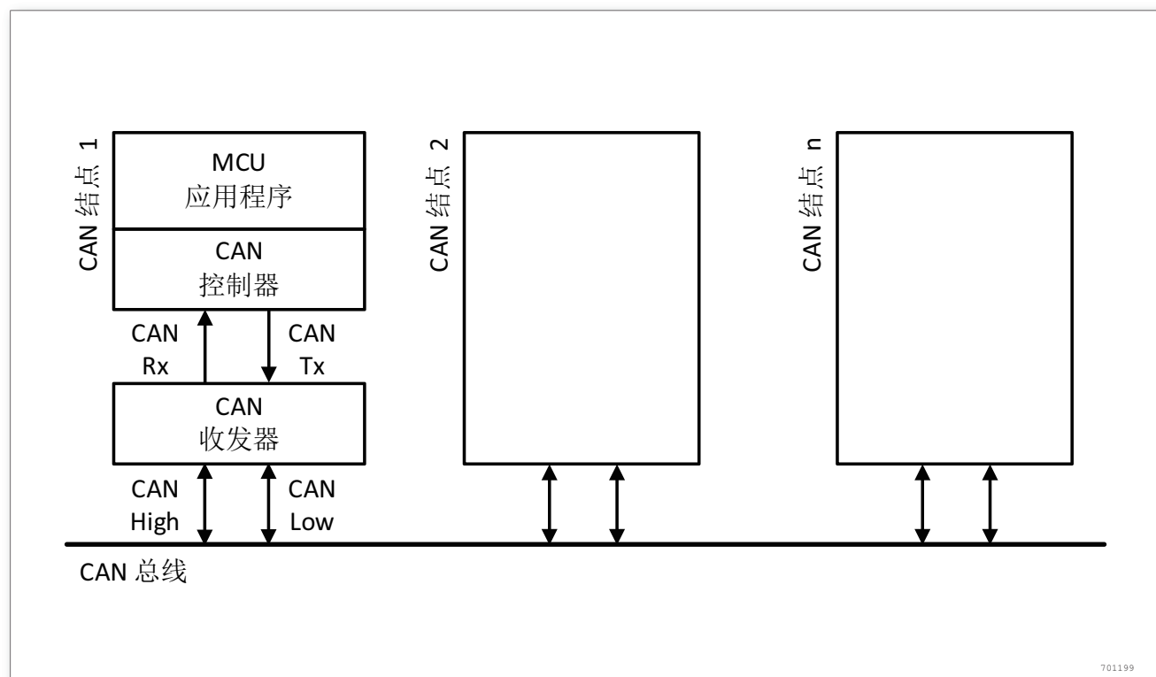
图 190. CAN 网络拓扑结构
