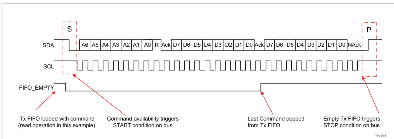
图 212. 主接收 - Tx FIFO 为空
