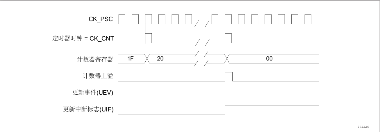
图 84. 计数器时序图，内部时钟分频因子为 N
