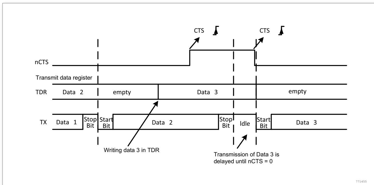
图 226. CTS 流控制
