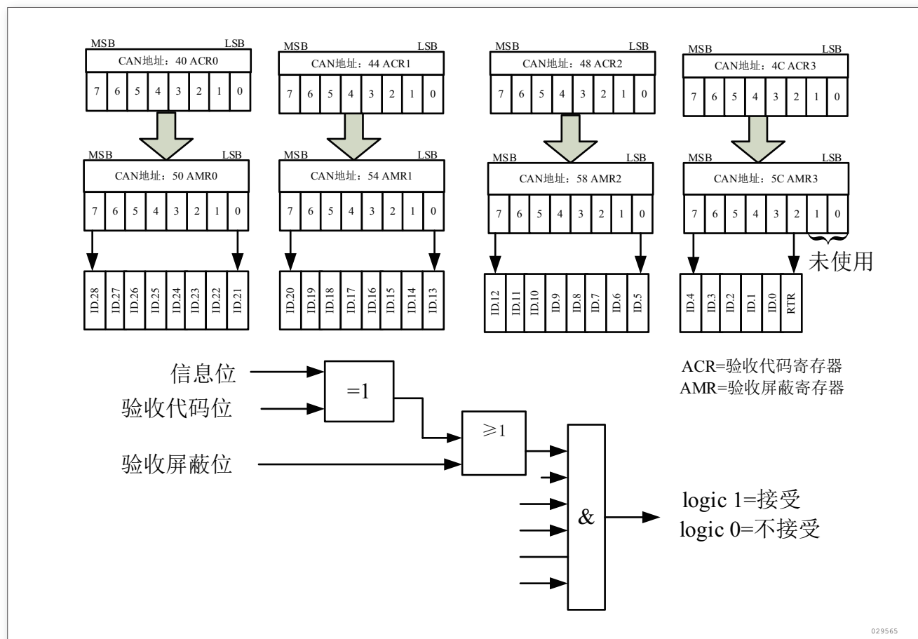
图 194. 单滤波器配置，接收扩展帧信息
