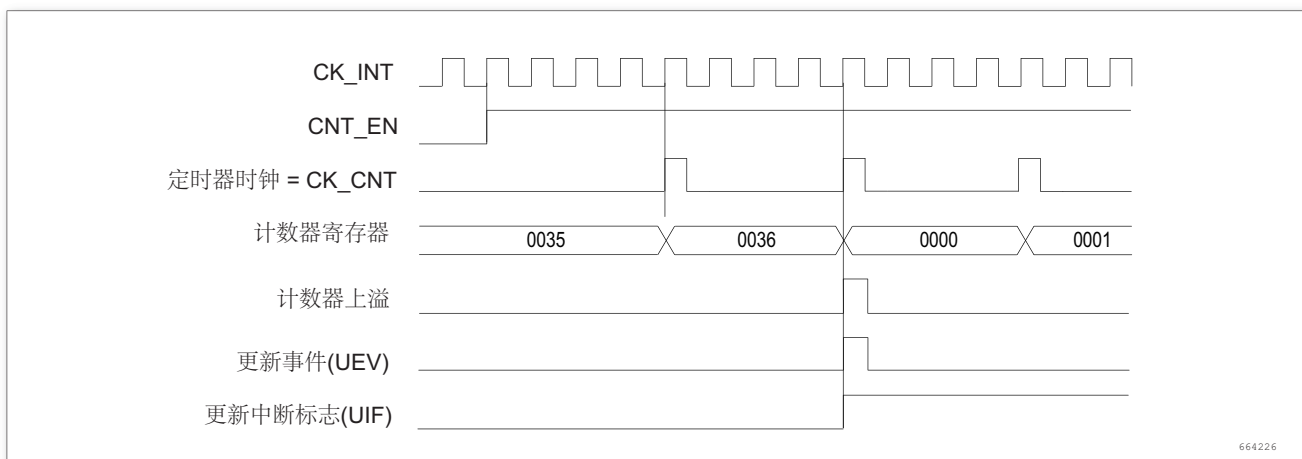
图 175. 计数器时序图，内部时钟分频因子为 4
