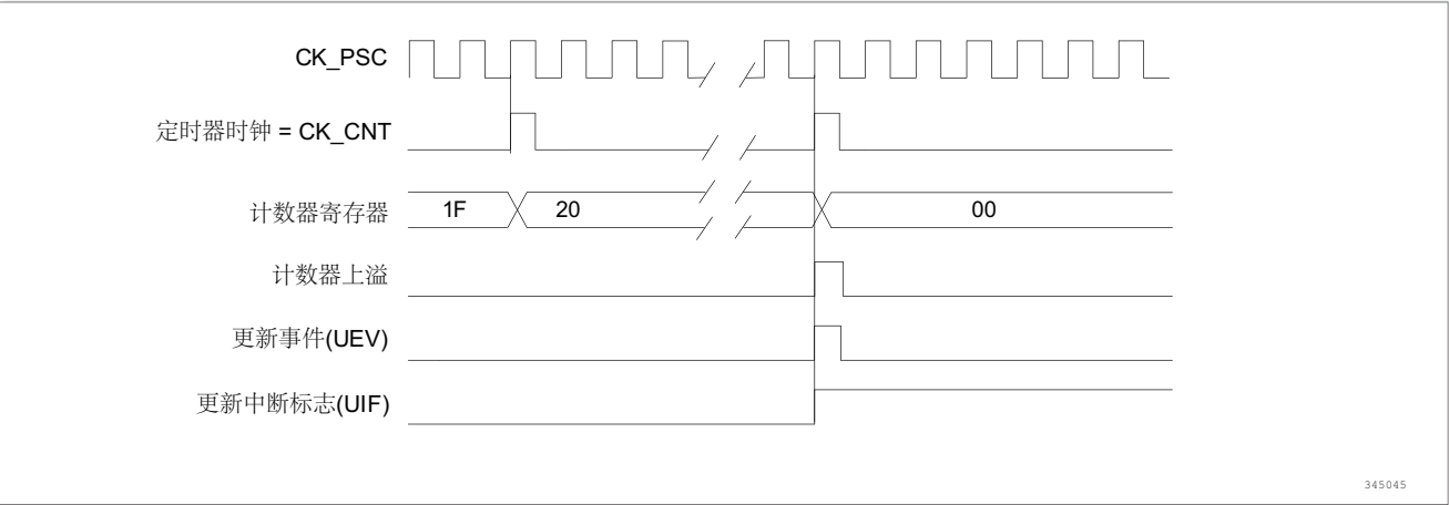
图 36. 计数器时序图，内部时钟分频因子为 N
