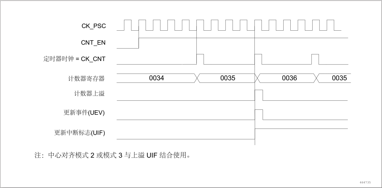
图 94. 计数器时序图，内部时钟分频因子为 4，TIMx_ARR = 0x36
