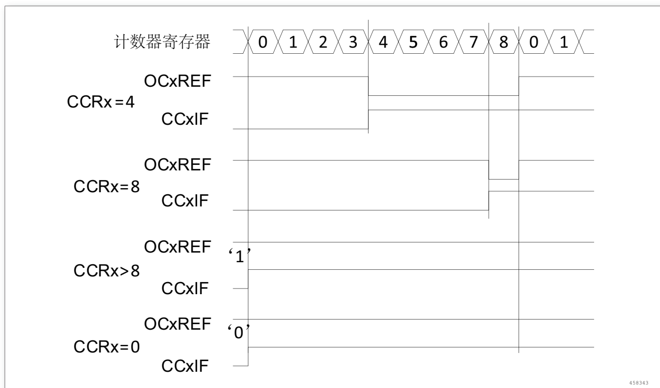
图 154. 边沿对齐的 PWM 波形 (ARR = 8)
