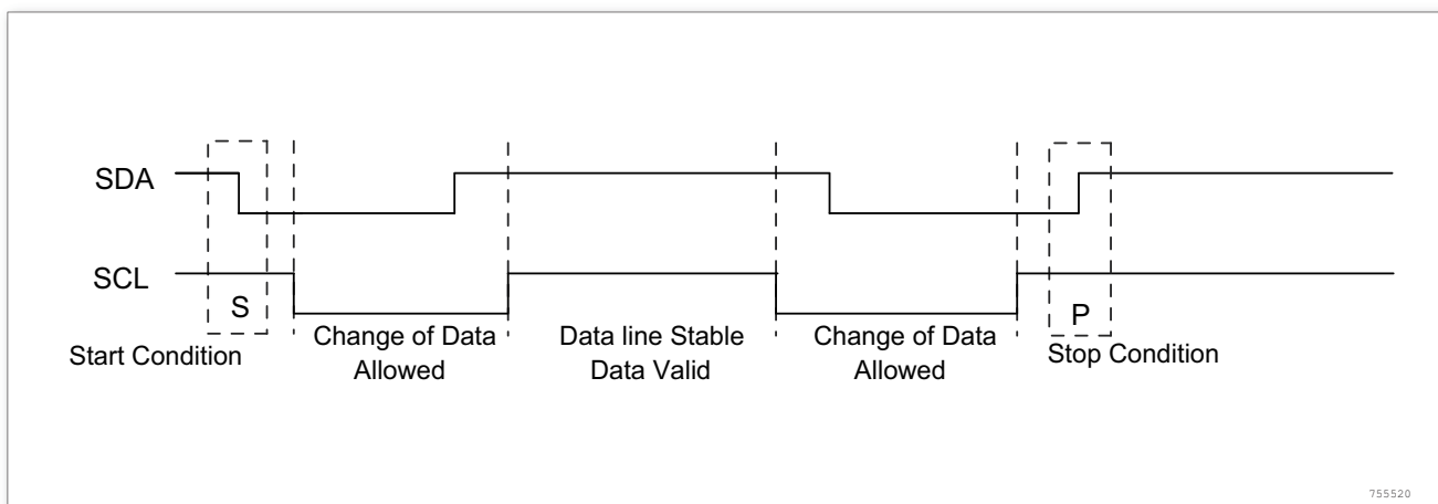
图 204. 起始和停止条件
