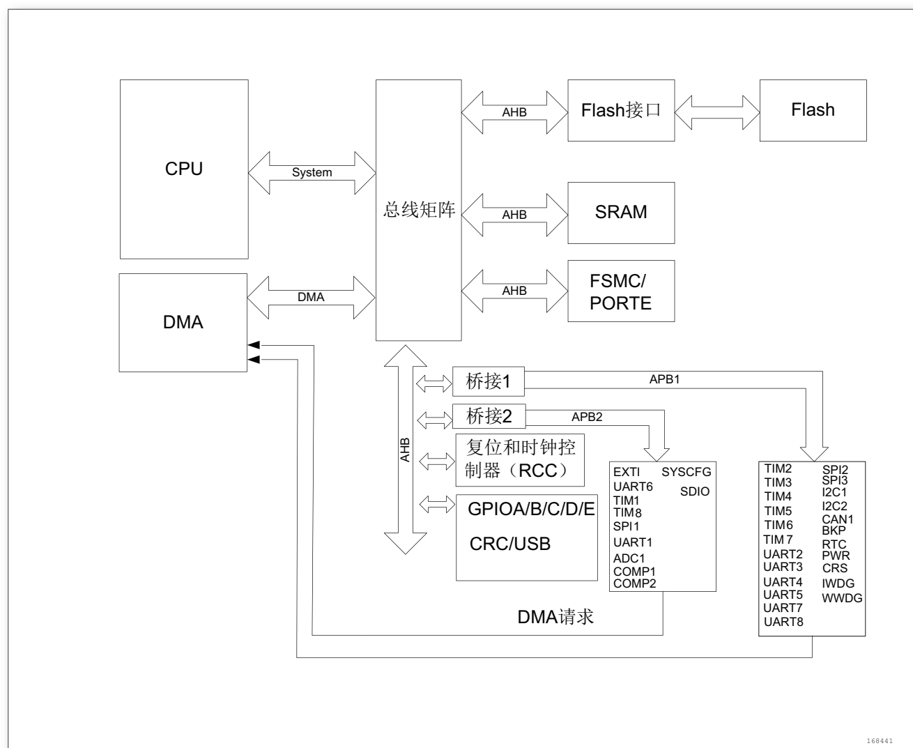
图 1. 系统架构
