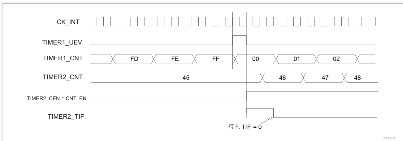
图 167. 使用定时器 1 的更新触发定时器 2
