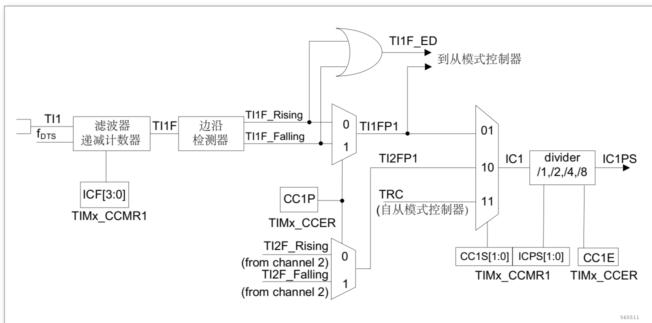
图 103. 捕获/比较通道 (如: 通道 1 输入部分)
