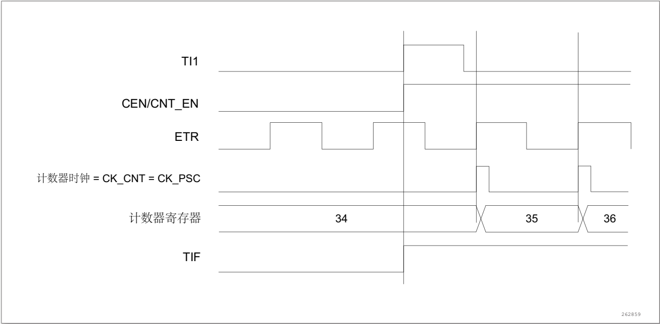
图 163. 外部时钟模式 2 + 触发模式下的控制电路
