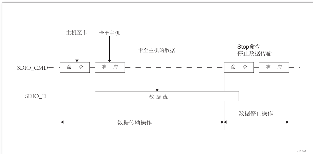
图 237. SDIO 连续读操作
