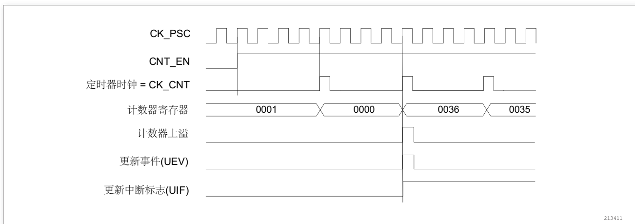
图 89. 计数器时序图，内部时钟分频因子为 4
