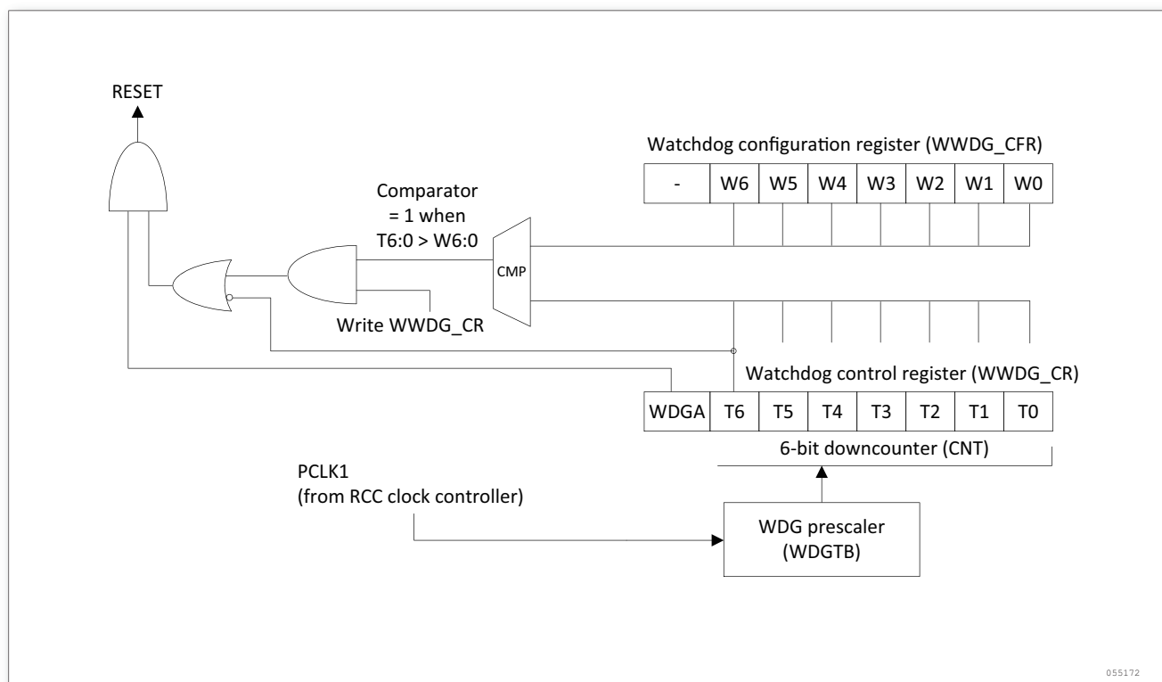
图 184. 看门狗框图
