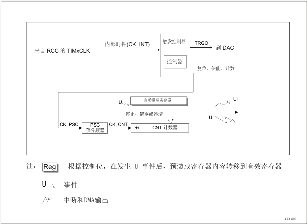
图 170. 基本定时器 TIM6 和 TIM7 框图
