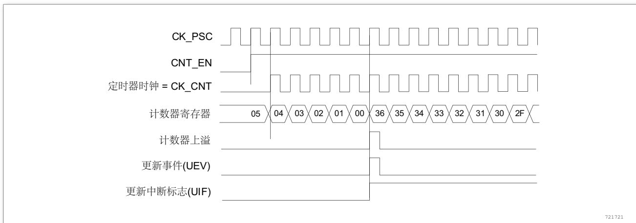
图 133. 计数器时序图，内部时钟分频因子为 1
