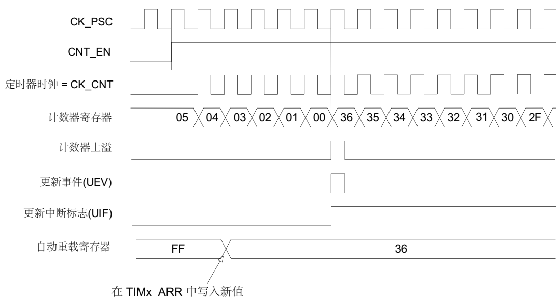
图 137. 计数器时序图，当没有使用重复计数器时的更新事件
