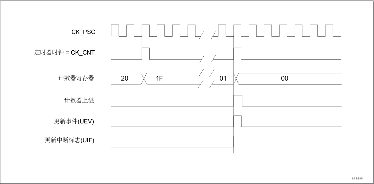
图 47. 计数器时序图，内部时钟分频因子为 N
