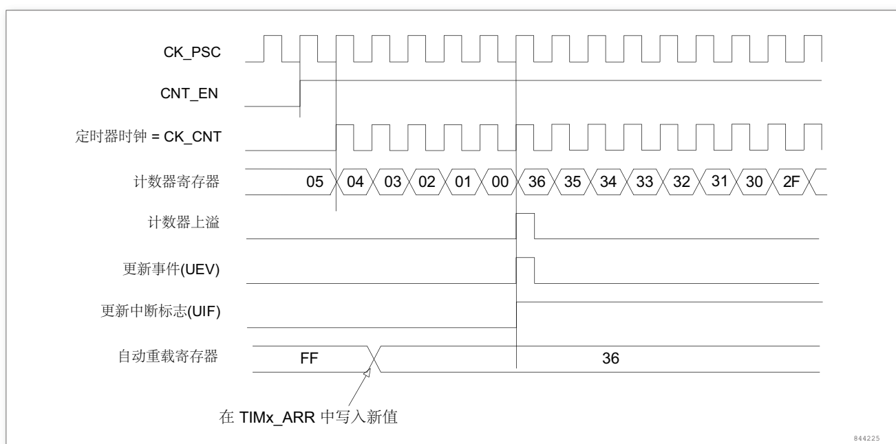
图 43. 计数器时序图，当没有使用重复计数器时的更新事件
