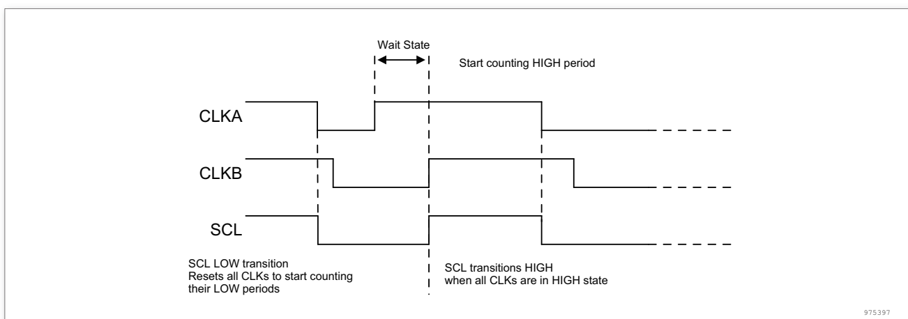
图 214. 多个主机时钟同步
