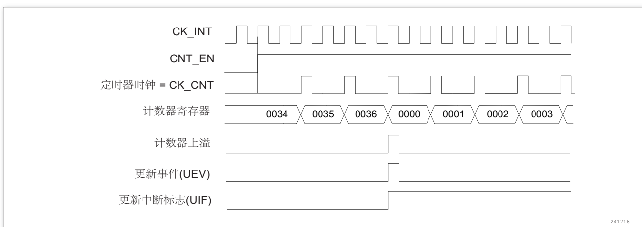
图 174. 计数器时序图，内部时钟分频因子为 2
