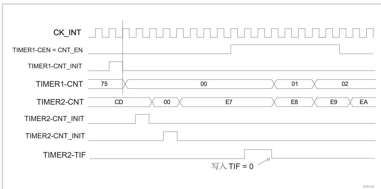
图 168. 利用定时器 1 的使能触发定时器 2
