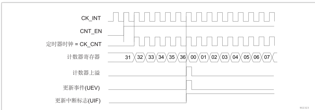
图 173. 计数器时序图，内部时钟分频因子为 1
