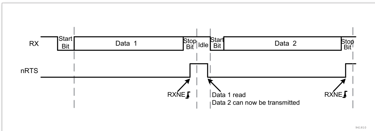
图 225. RTS 流控制
