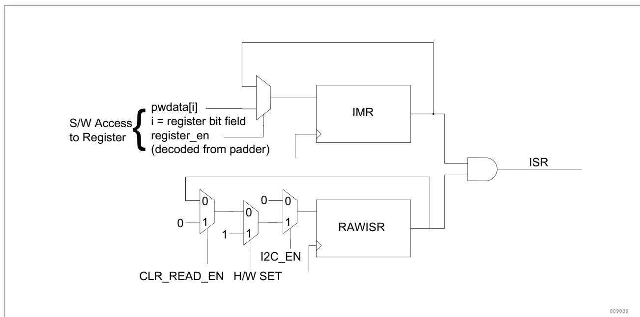
图 217. 中断机制
