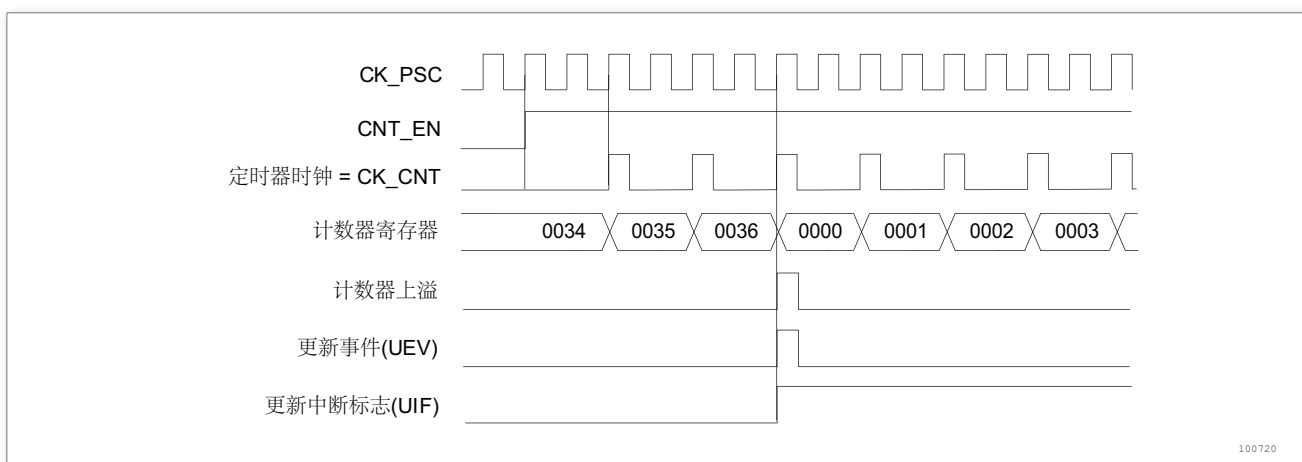
图 128. 计数器时序图，内部时钟分频因子为 2
