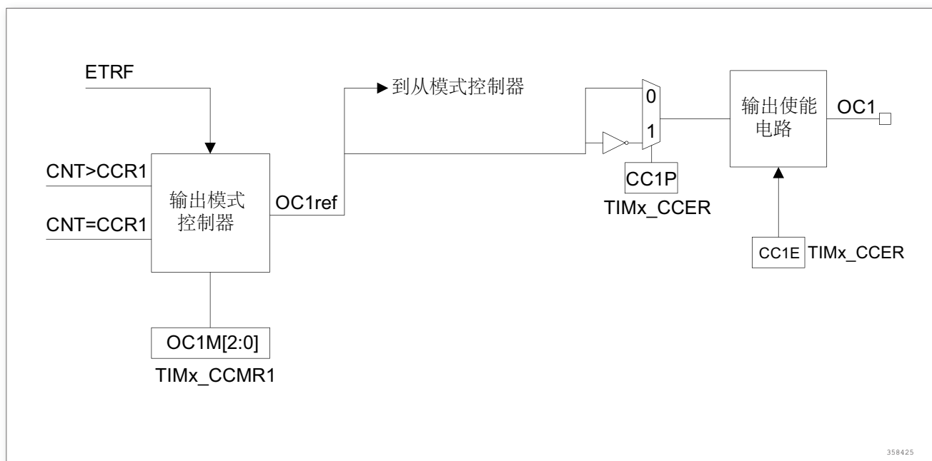
图 151. 捕获/比较通道的输出部分 (通道 1)
