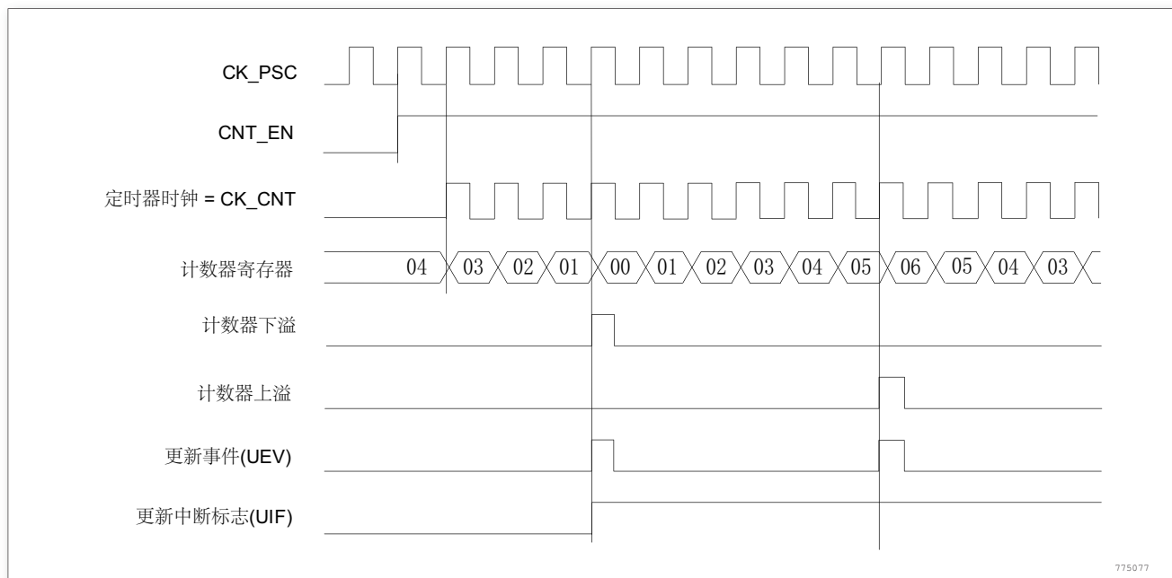
图 138. 计数器时序图，内部时钟分频因子为 1，TIMx_ARR = 0x6
