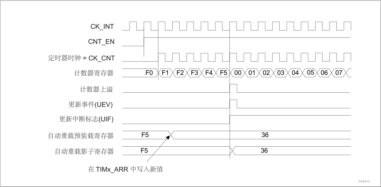
图 178. 计数器时序图，当 ARPE = 1 时的更新事件 (TIMx_ARR 预装载)
