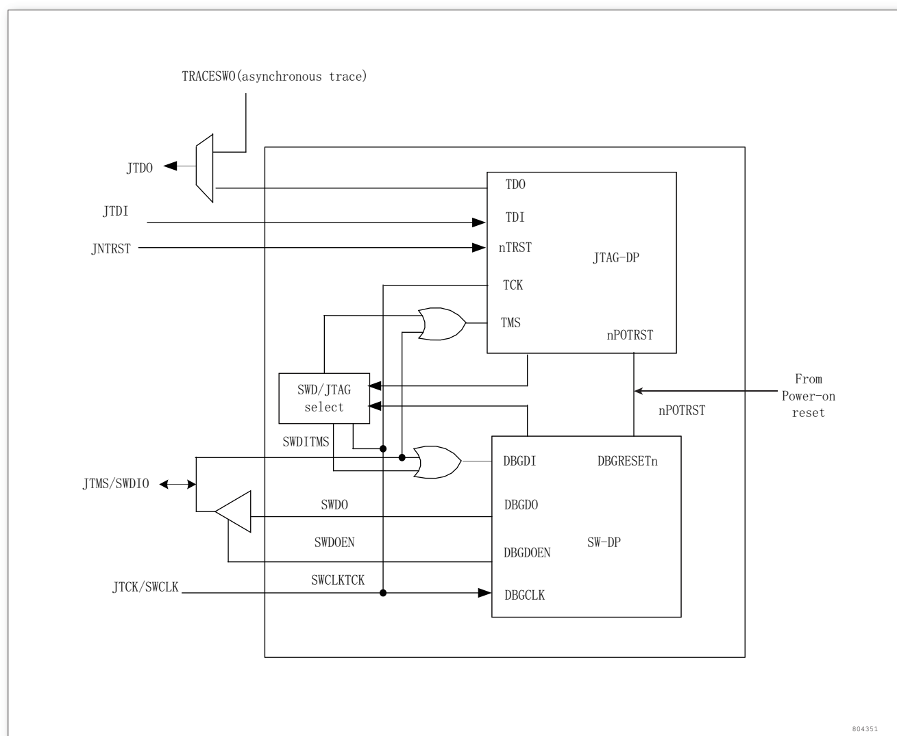
图 228. SWJ 调试端口
