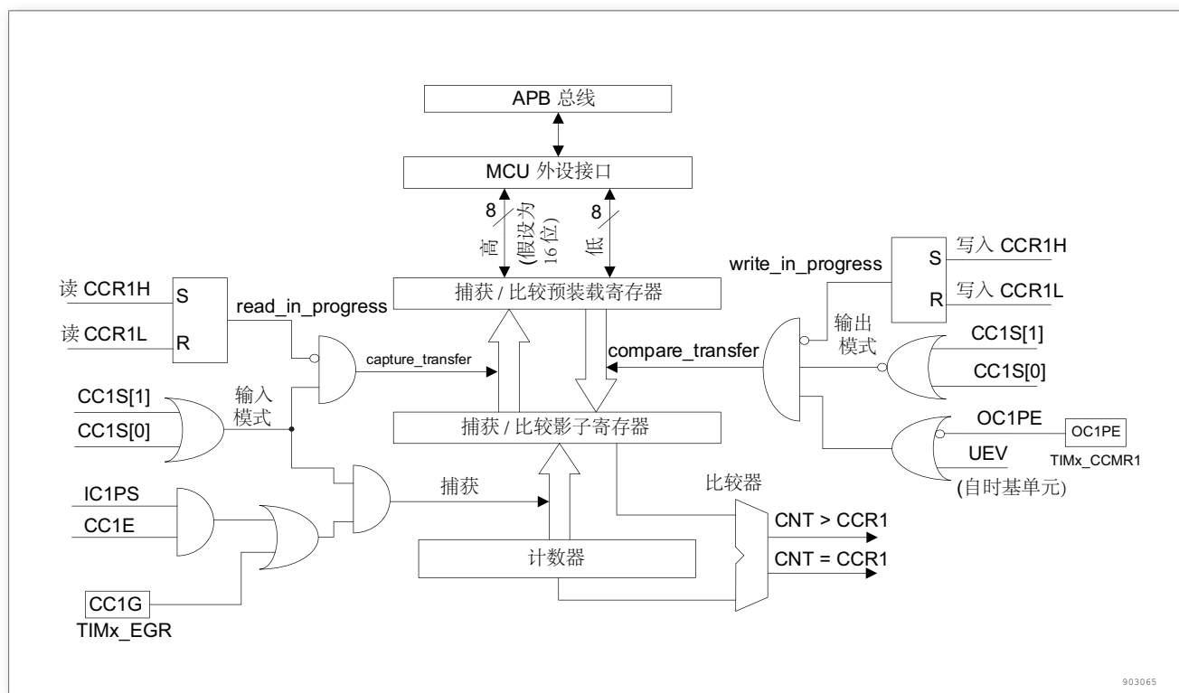
图 150. 捕获/比较通道 1 的主电路
