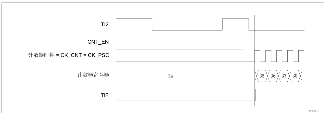
图 162. 触发器模式下的控制电路
