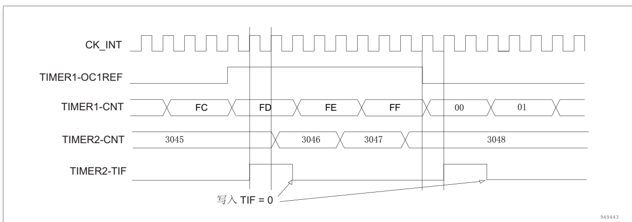
图 165. 定时器 1 的 OC1REF 控制定时器 2
