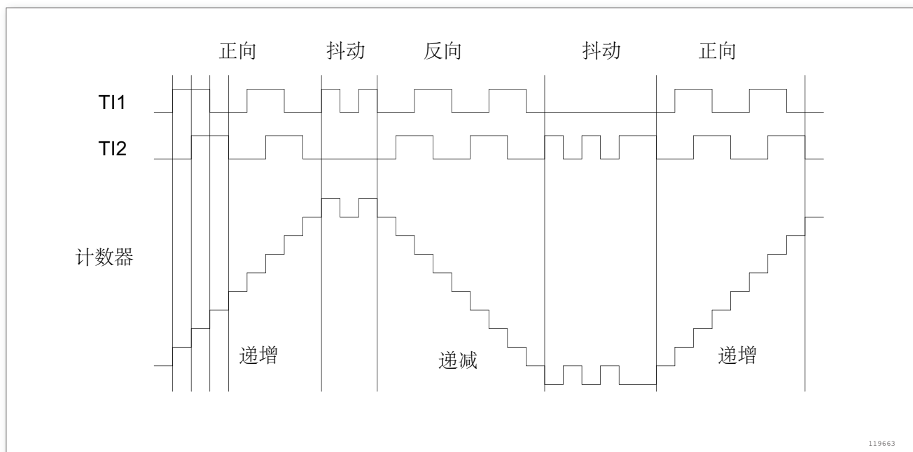
图 158. 编码器模式下的计数器操作实例
