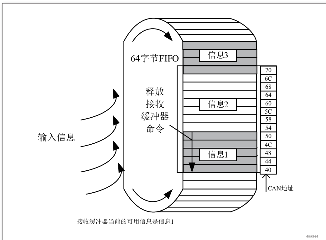
图 198. 标准帧和扩展帧格式配置在发送缓冲器的列表
