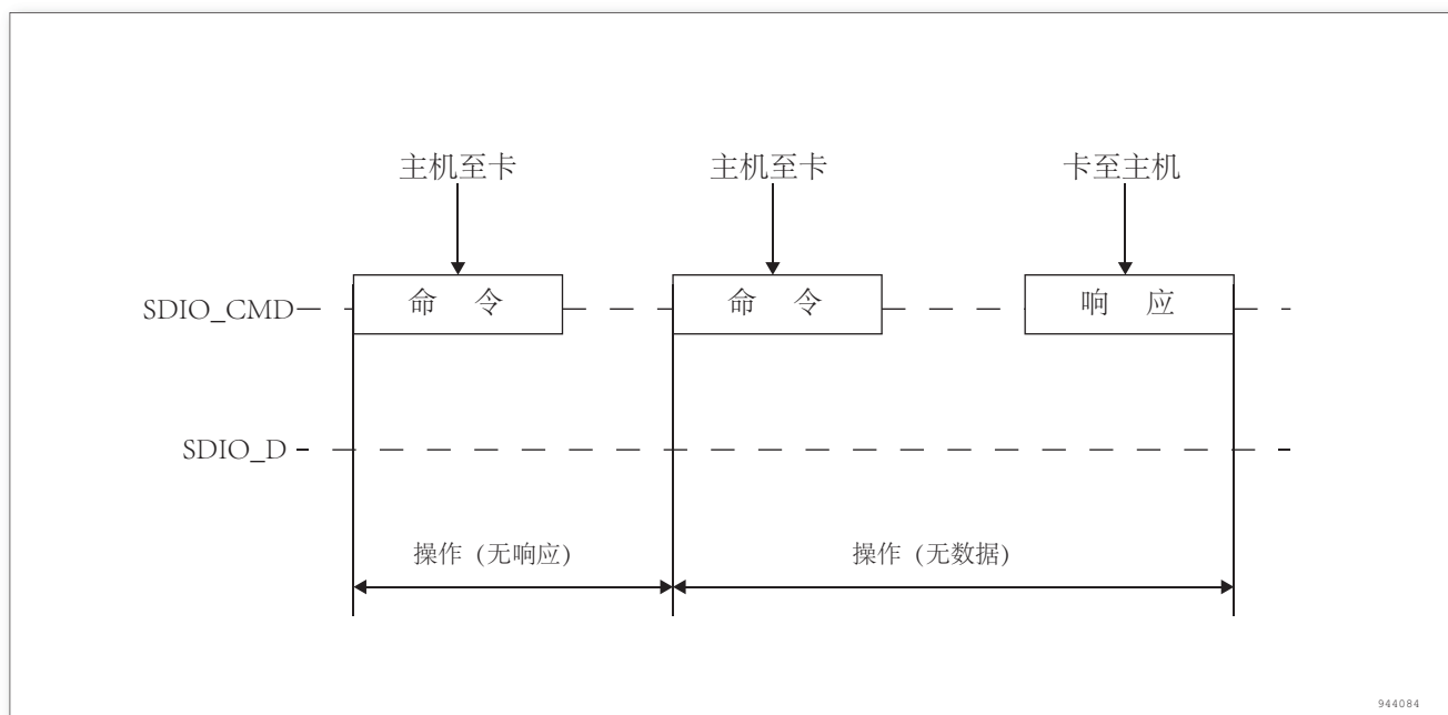
图 234. SDIO “无响应”和“无数据”操作
