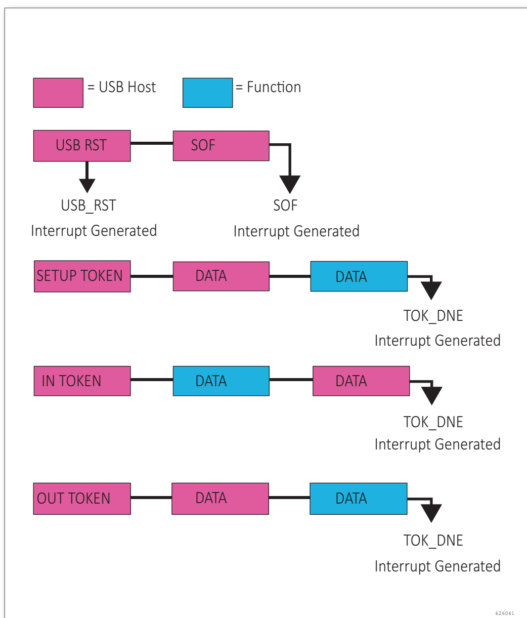
图 188. 令牌交易
