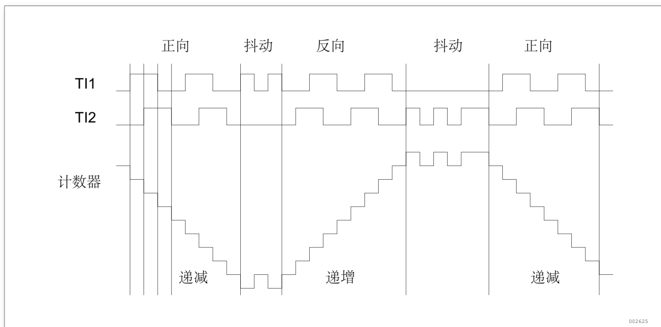
图 159. IC1FP1 反相的编码器接口模式实例
