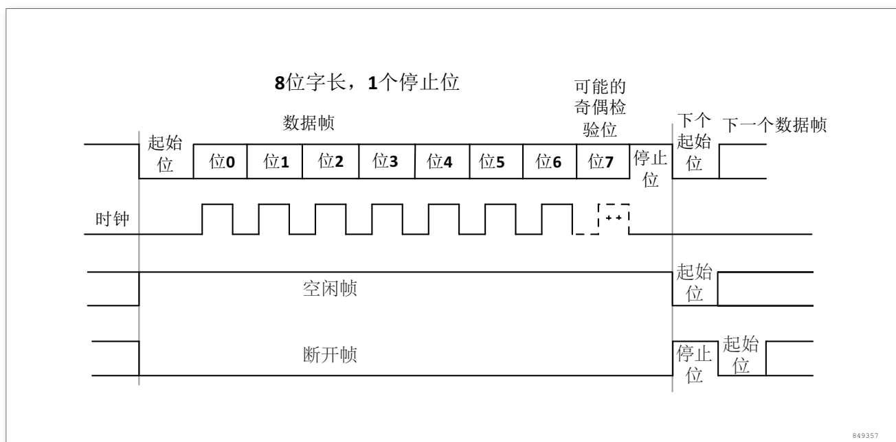
图 219. UART 时序
