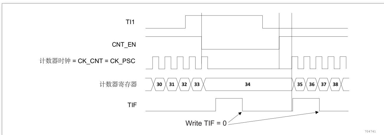
图 161. 门控模式下的控制电路
