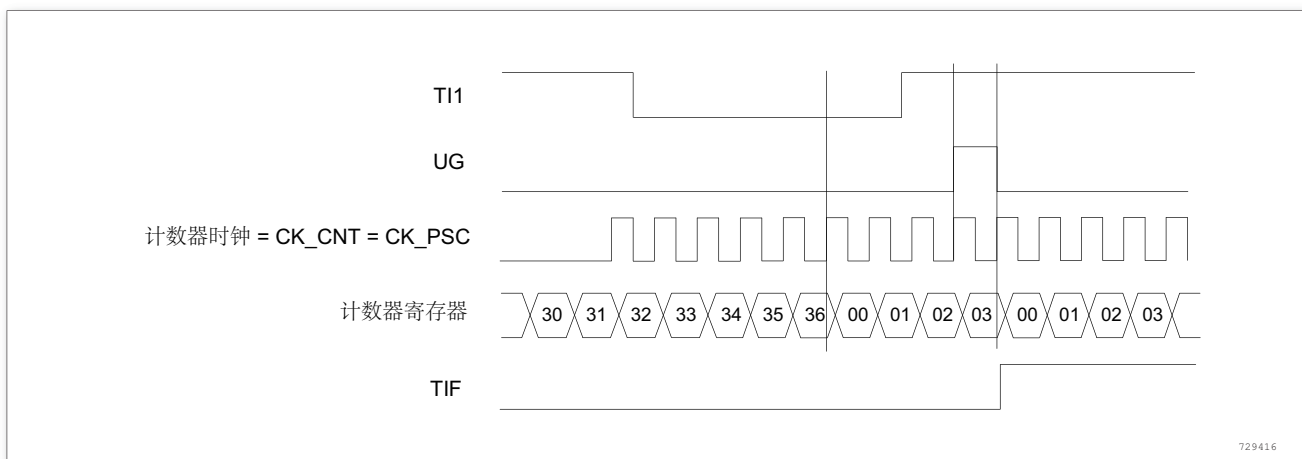
图 160. 复位模式下的控制电路
