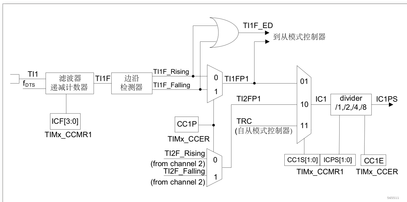
图 149. 捕获/比较通道 (如: 通道 1 输入部分)
