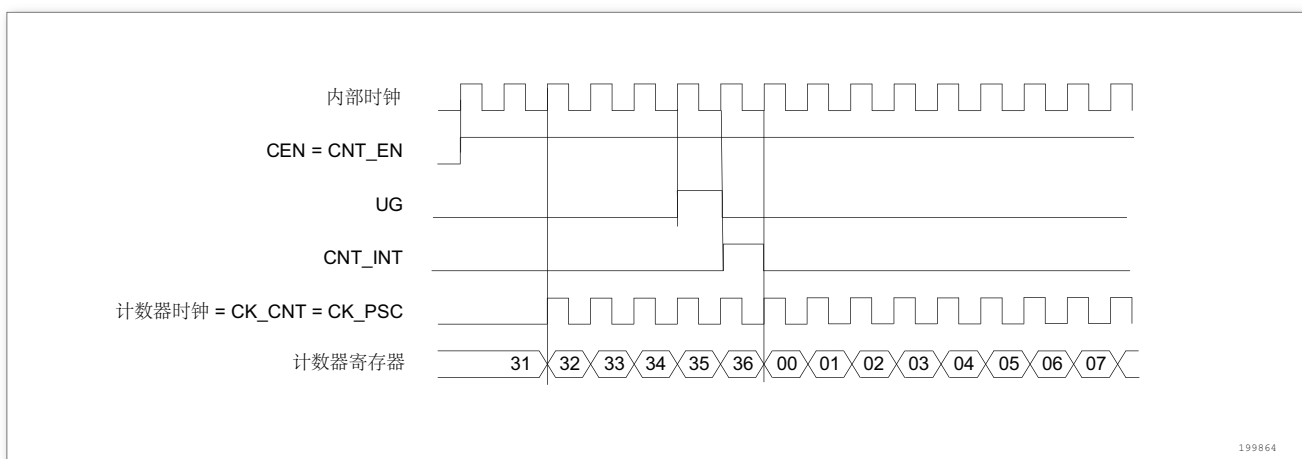
图 144. 一般模式下的控制电路, 内部时钟分频因子为 1
