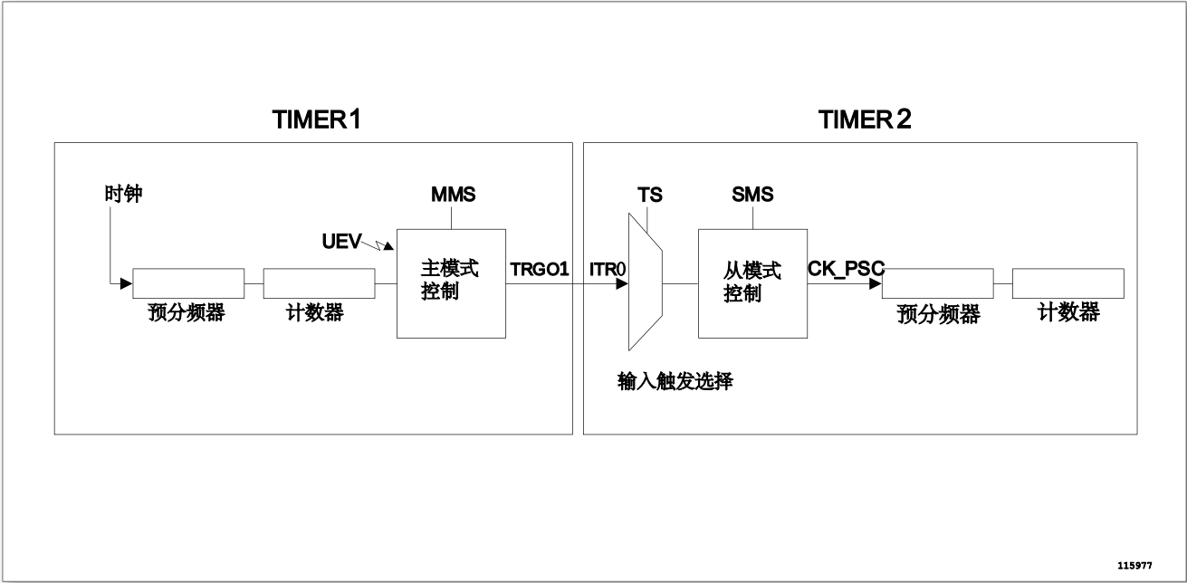
图 164. 主/从定时器的例子
