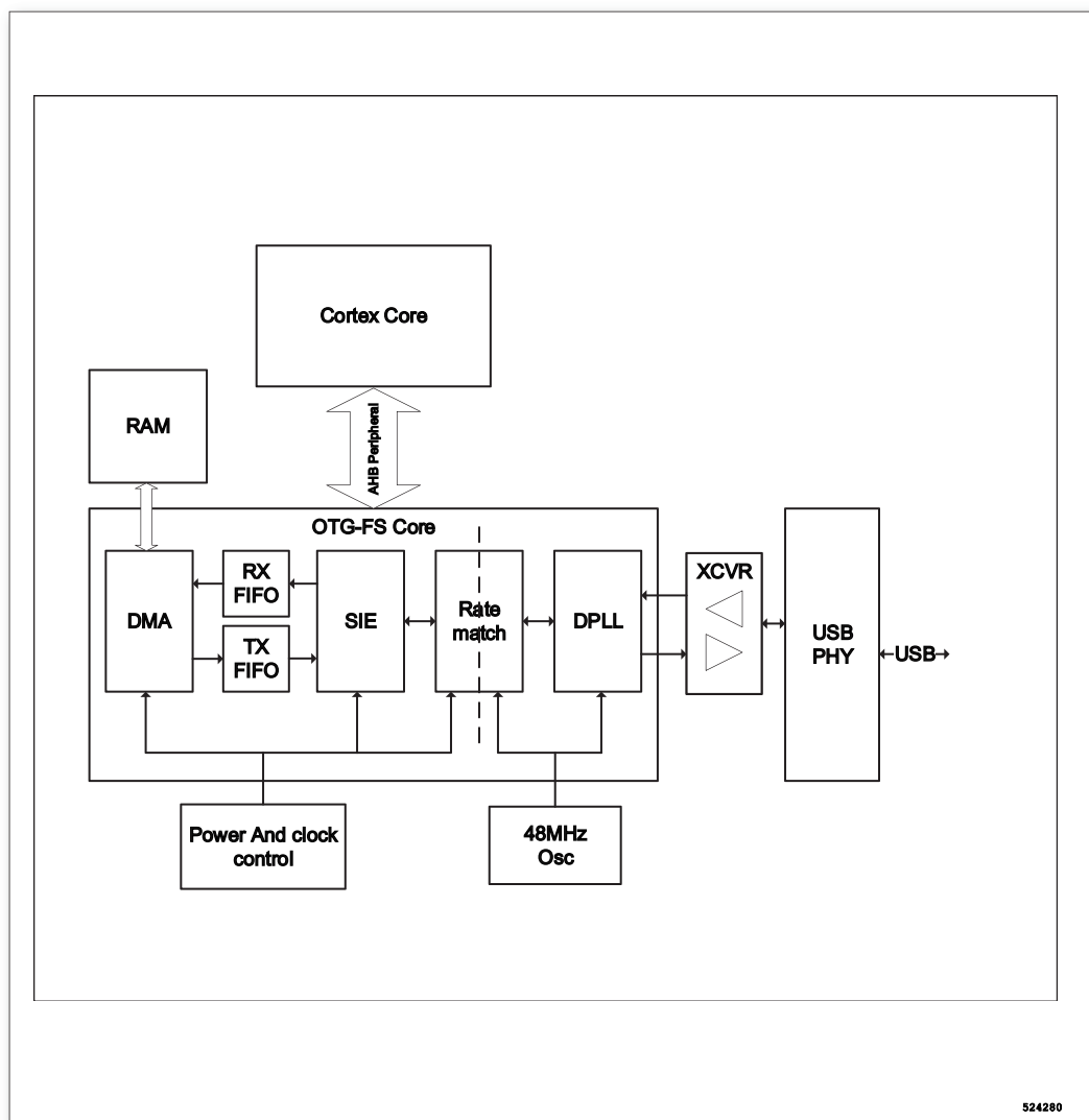
图 186. OTG-FS 功能框图
