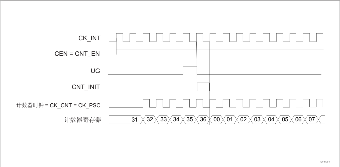
图 179. 一般模式下的控制电路，内部时钟分频因子为 1
