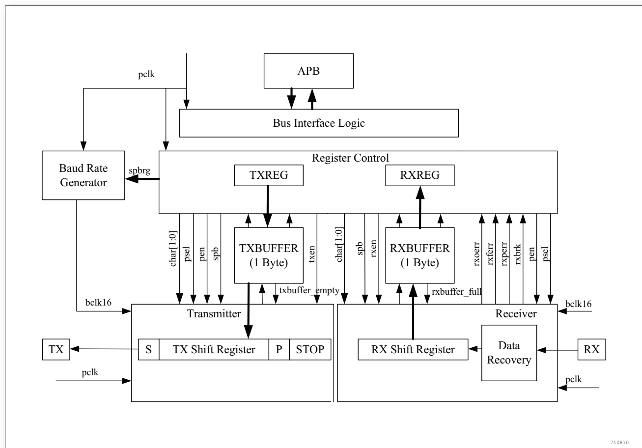
图 218. UART 方框图
