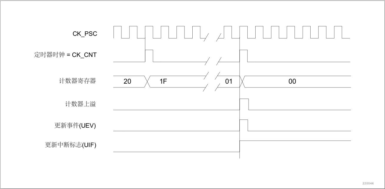
图 95. 计数器时序图，内部时钟分频因子为 N
