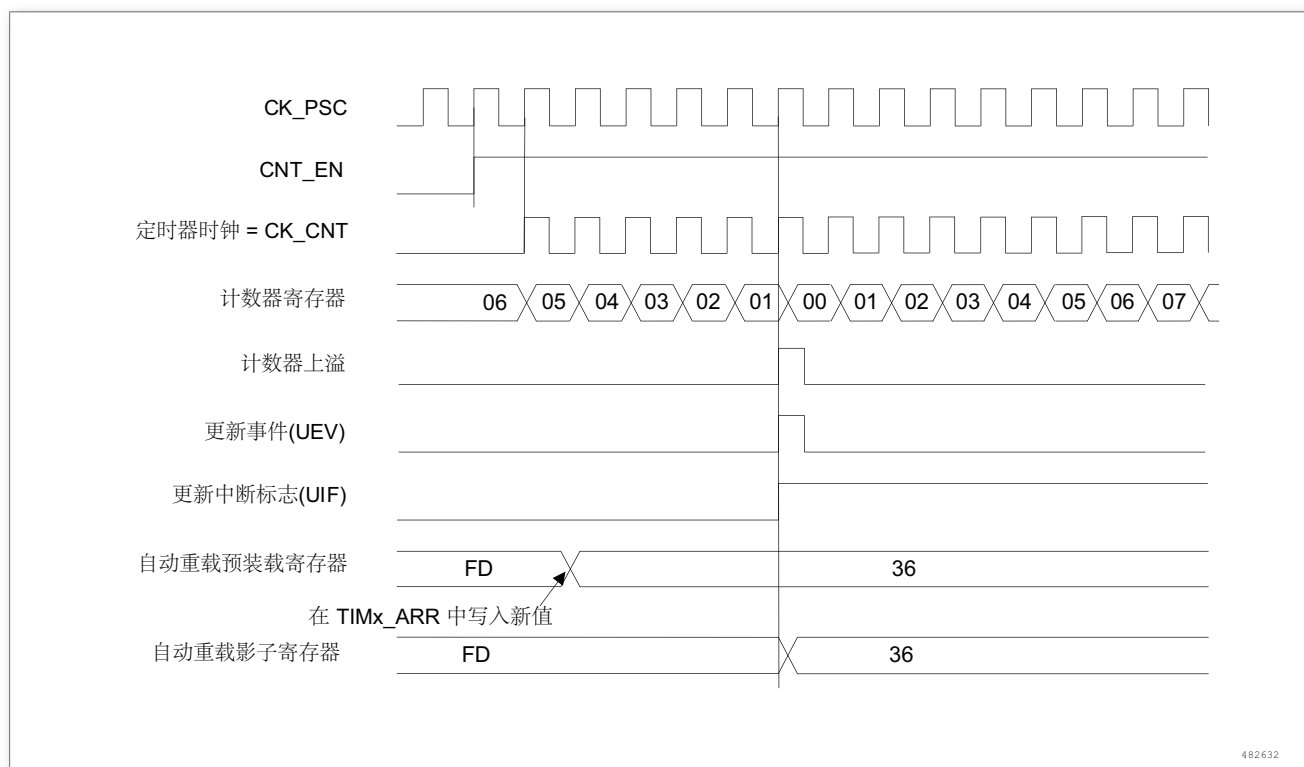
图 142. 计数器时序图, ARPE = 1 时的更新事件 (计数器下溢)
