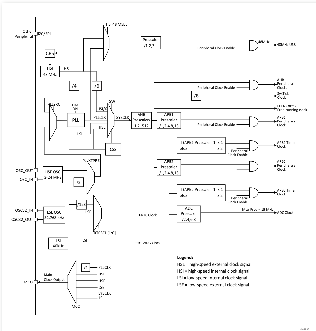
图 12. 时钟树
