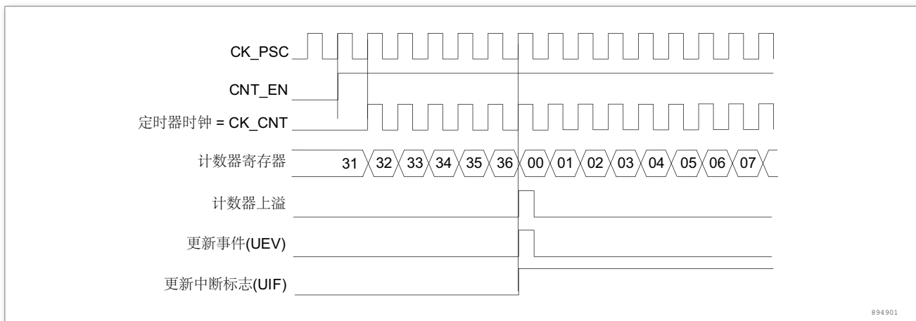
图 127. 计数器时序图，内部时钟分频因子为 1
