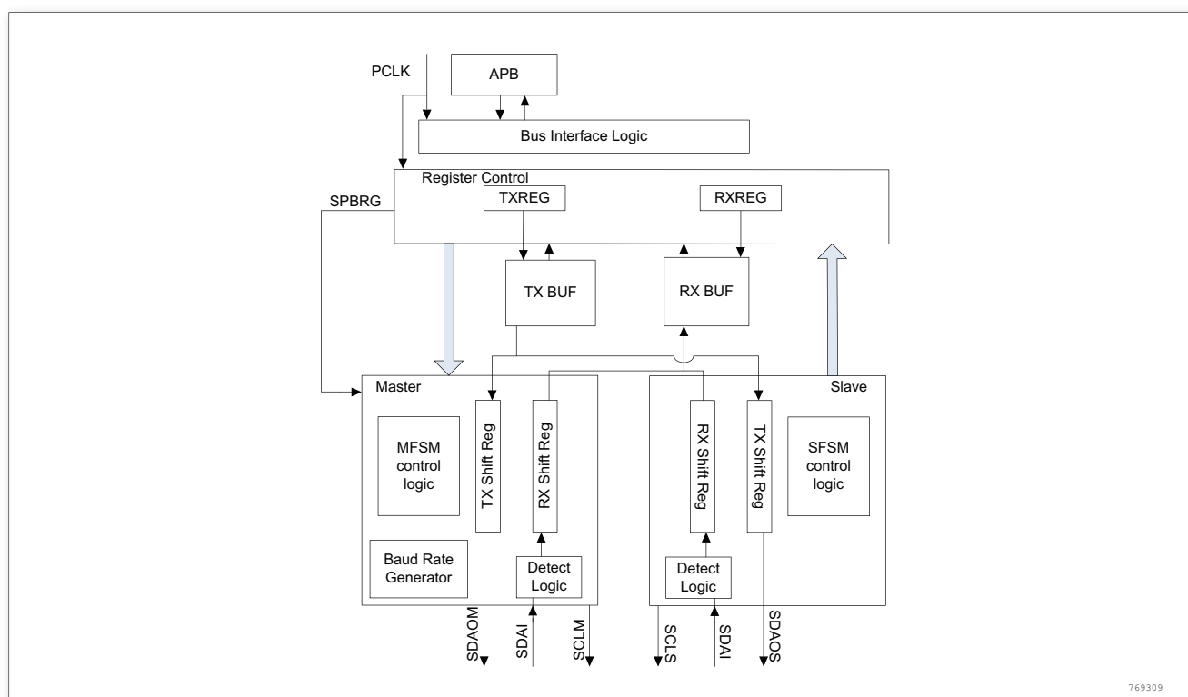
图 215. I2C 功能框图
