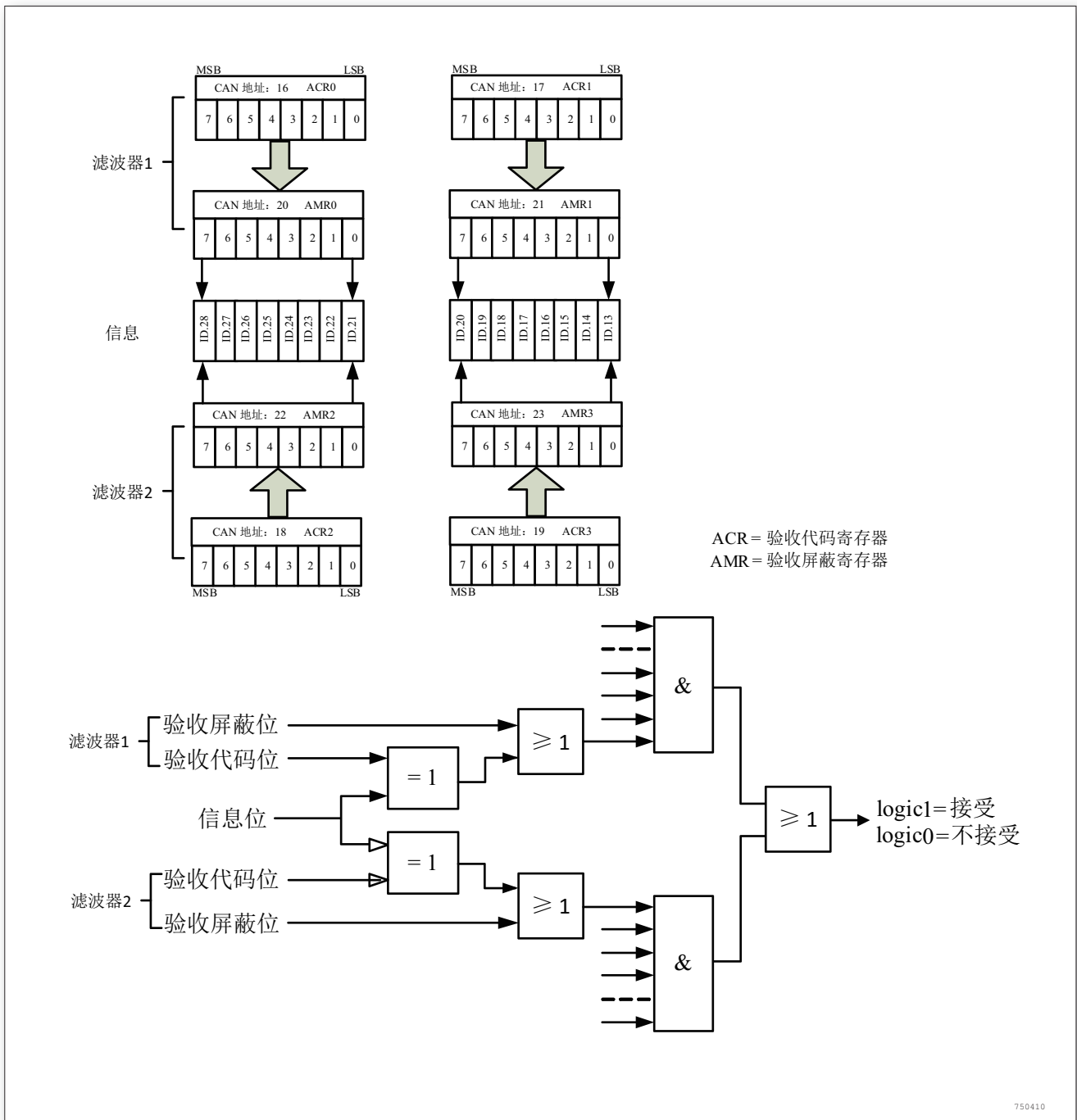
图 196. 双滤波器配置，接收扩展帧信息
