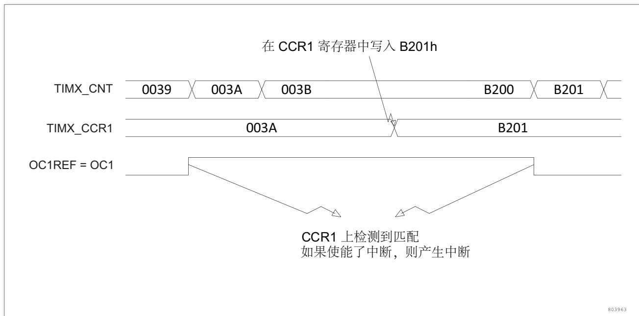
图 153. 输出比较模式，翻转 OC1
