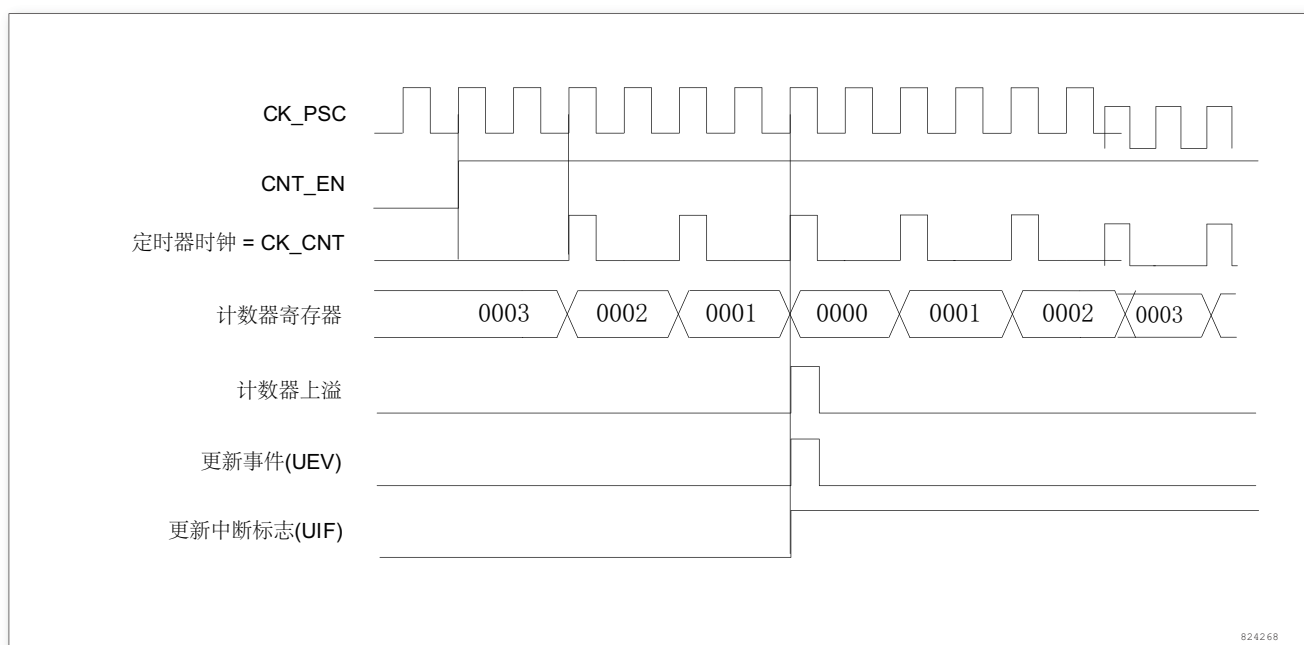
图 139. 计数器时序图，内部时钟分频因子为 2
