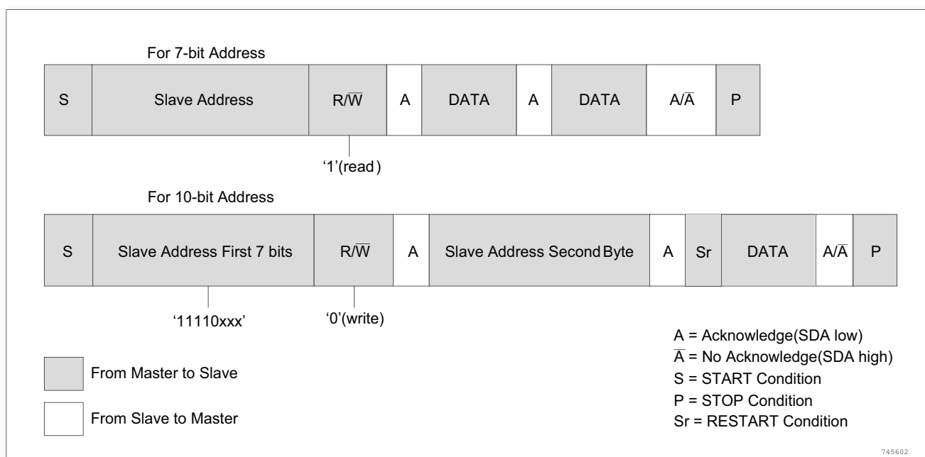
图 208. 主接收协议
