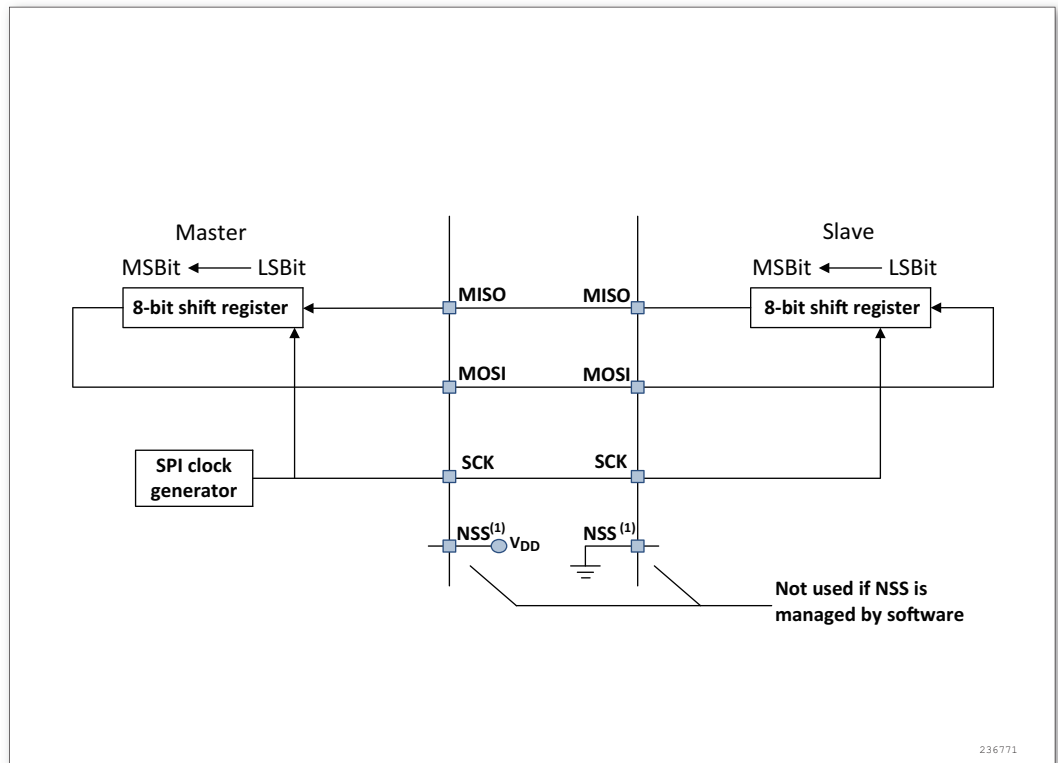
图 202. 单主和单从应用
