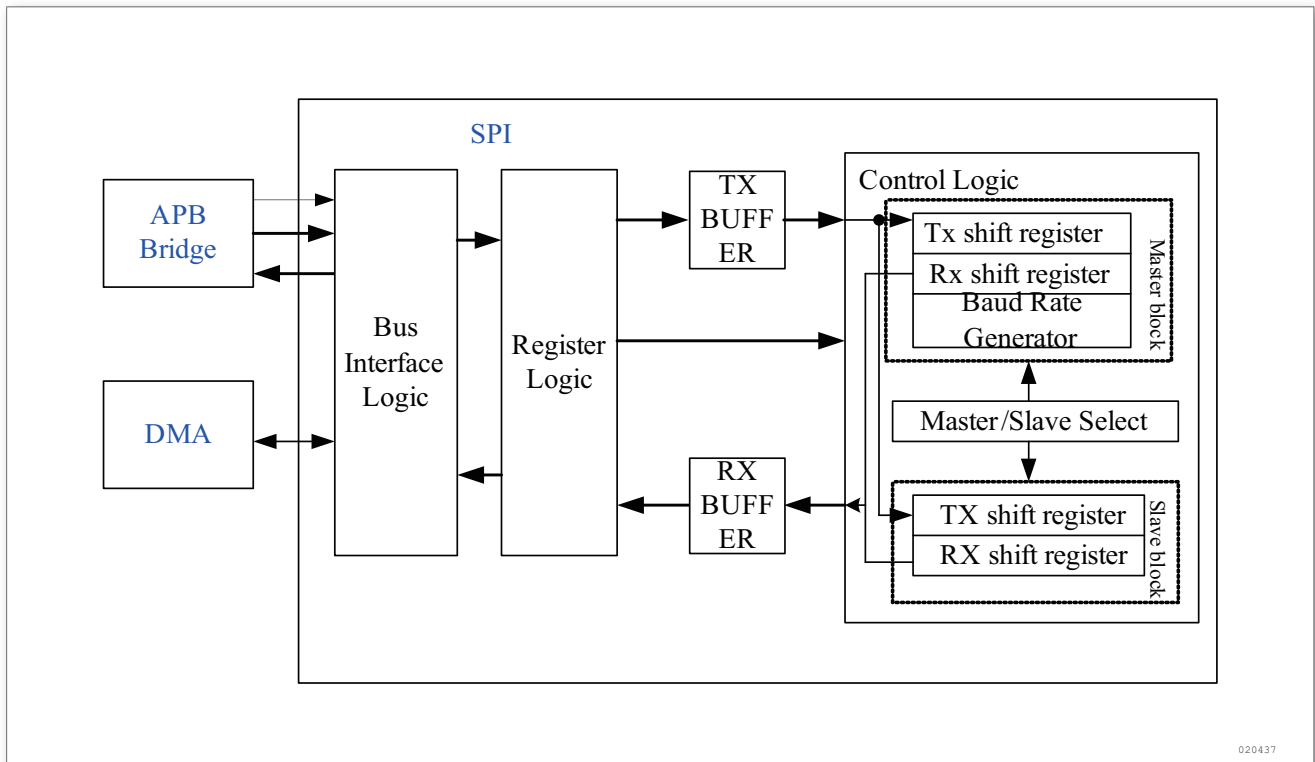
图 201. SPI 框图
