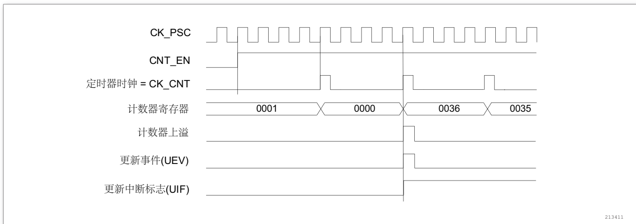
图 135. 计数器时序图，内部时钟分频因子为 4
