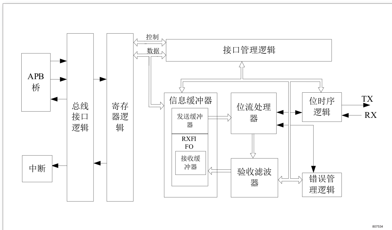
图 191. CAN 结构方框图
