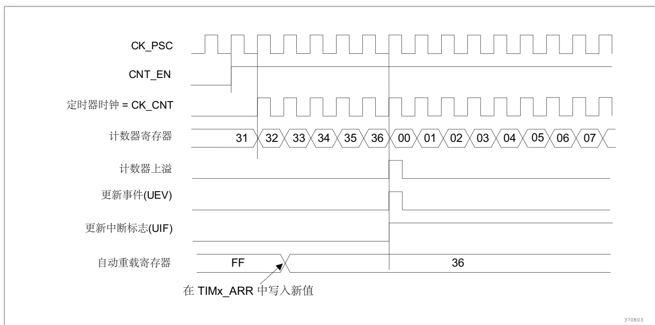
图 131. 计数器时序图，当 ARPE = 0 时的更新事件 (TIMx_ARR 没有预装入)
