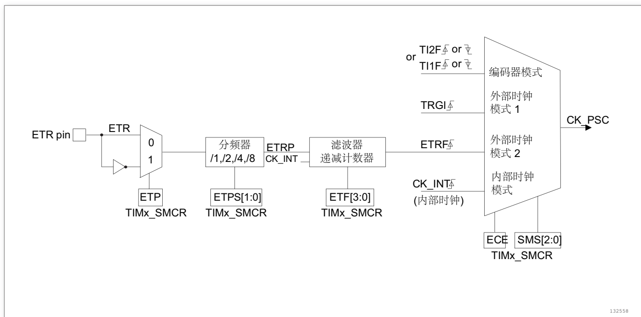
图 147. 外部触发输入框图
