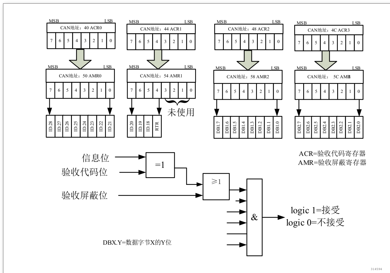
图 193. 接收标准结构信息时的单个滤波器配置
