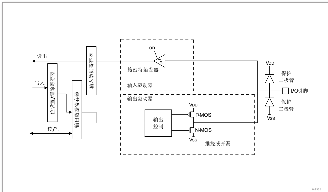
图 16. 输出配置
