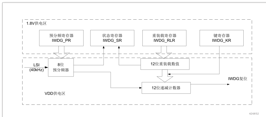
图 183. 独立看门狗框图
