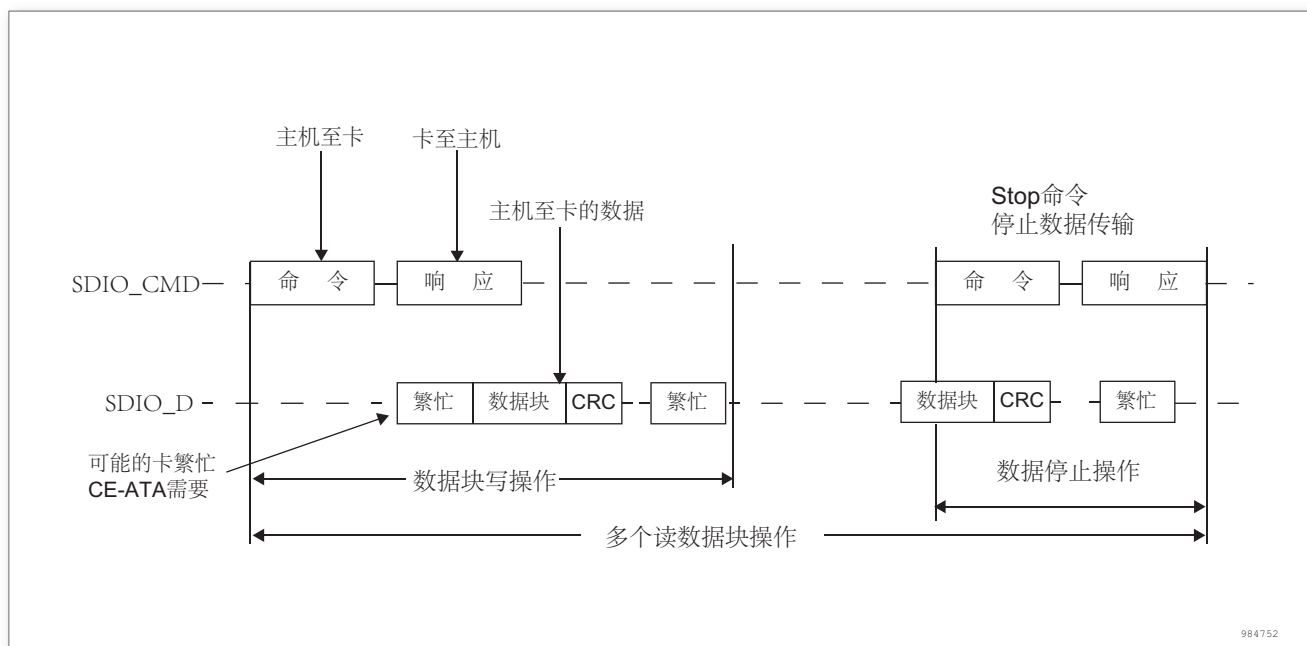
图 236. SDIO(多) 数据块写操作
