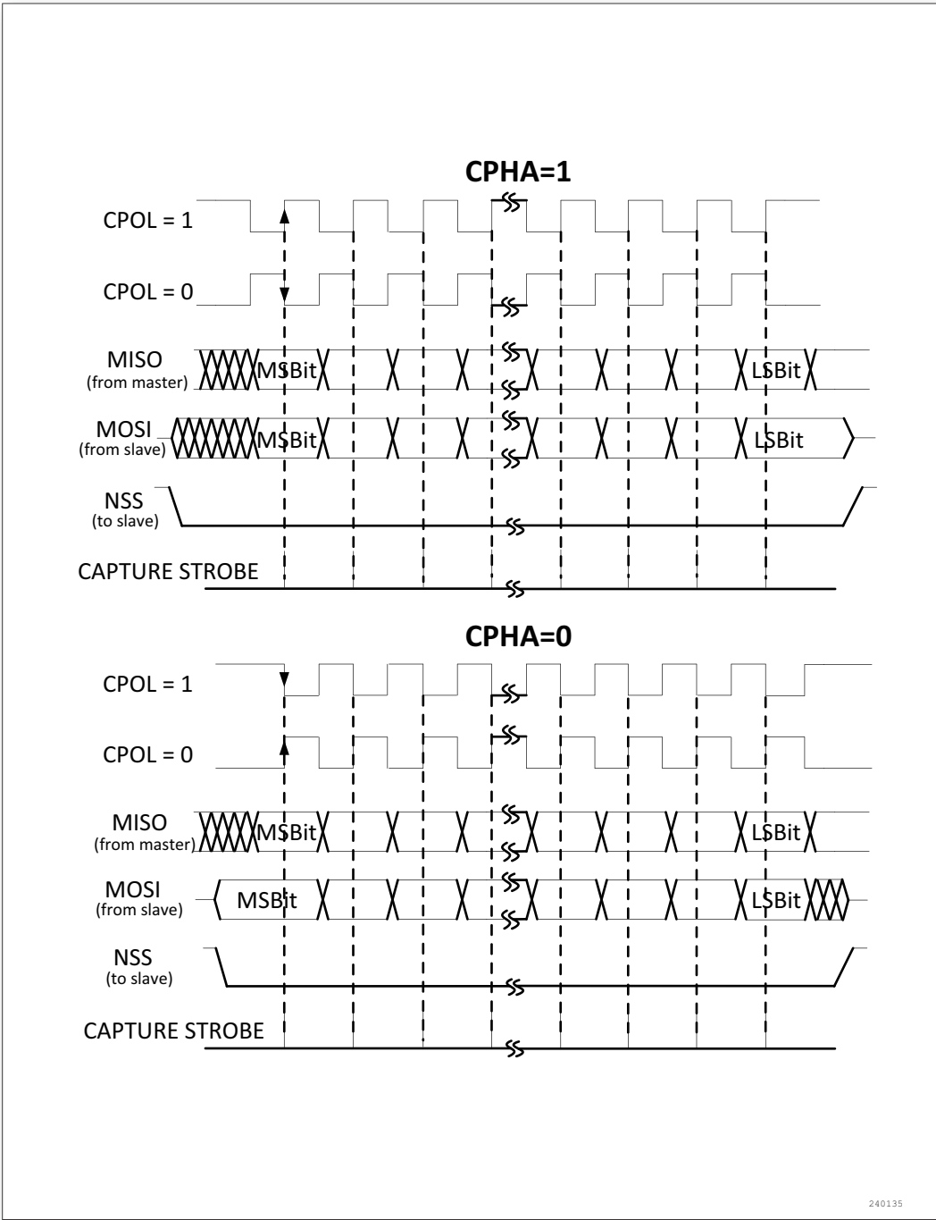
图 203. 数据时钟时序图
