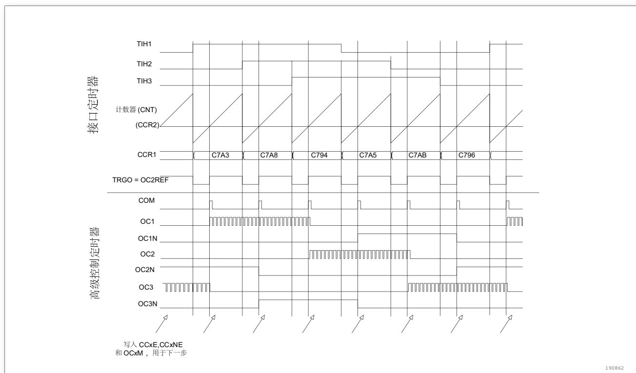
图 73. 霍尔传感器接口的实例
