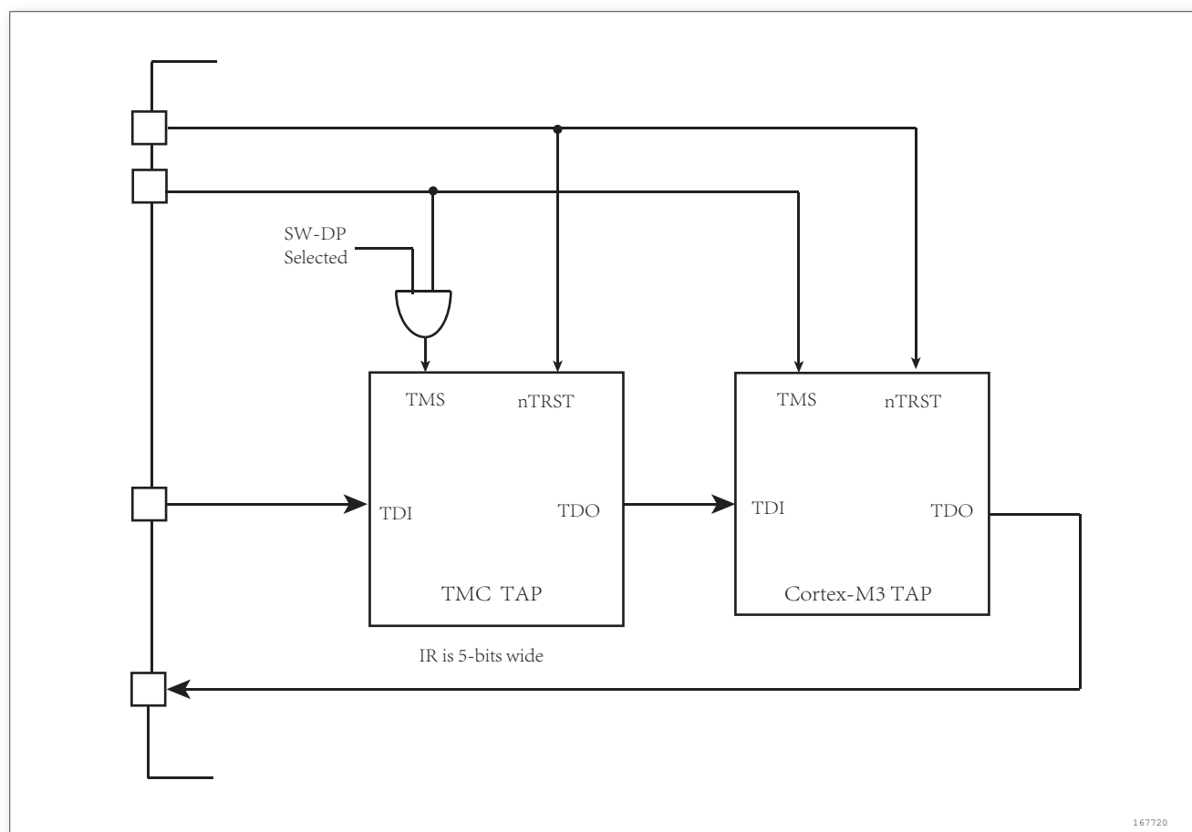
图 229. JTAG TAP 连接
