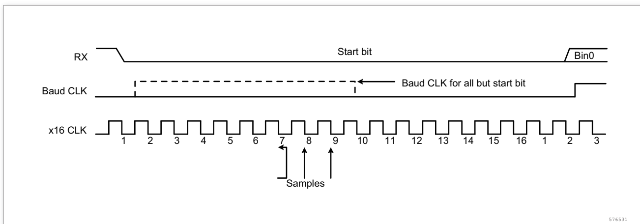
图 223. RX 引脚采样方案
