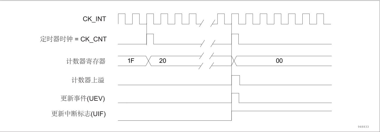
图 176. 计数器时序图，内部时钟分频因子为 N
