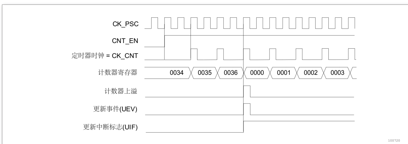
图 82. 计数器时序图，内部时钟分频因子为 2
