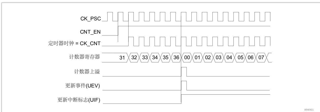
图 81. 计数器时序图，内部时钟分频因子为 1
