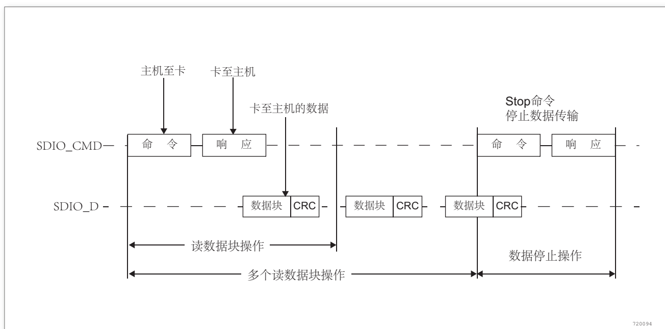
图 235. SDIO(多) 数据块读操作
