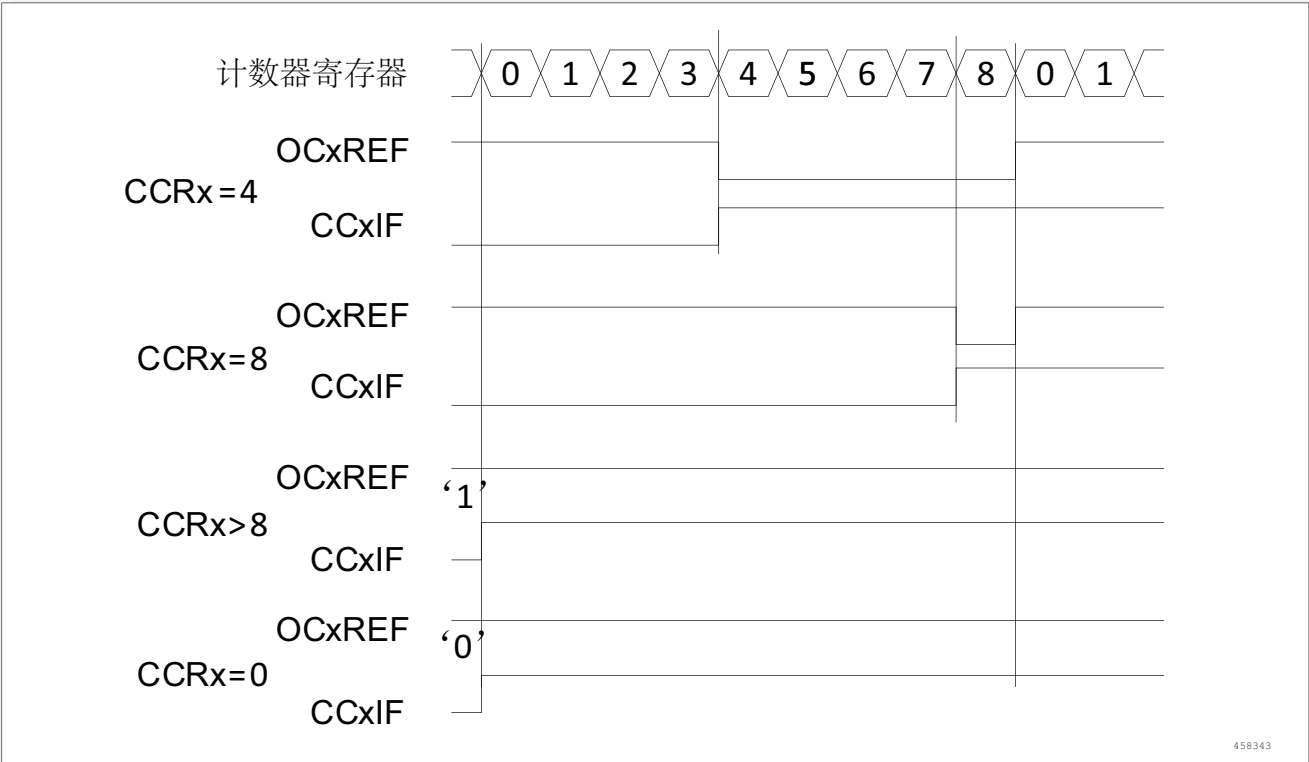
图 108. 边沿对齐的 PWM 波形 (ARR = 8)
