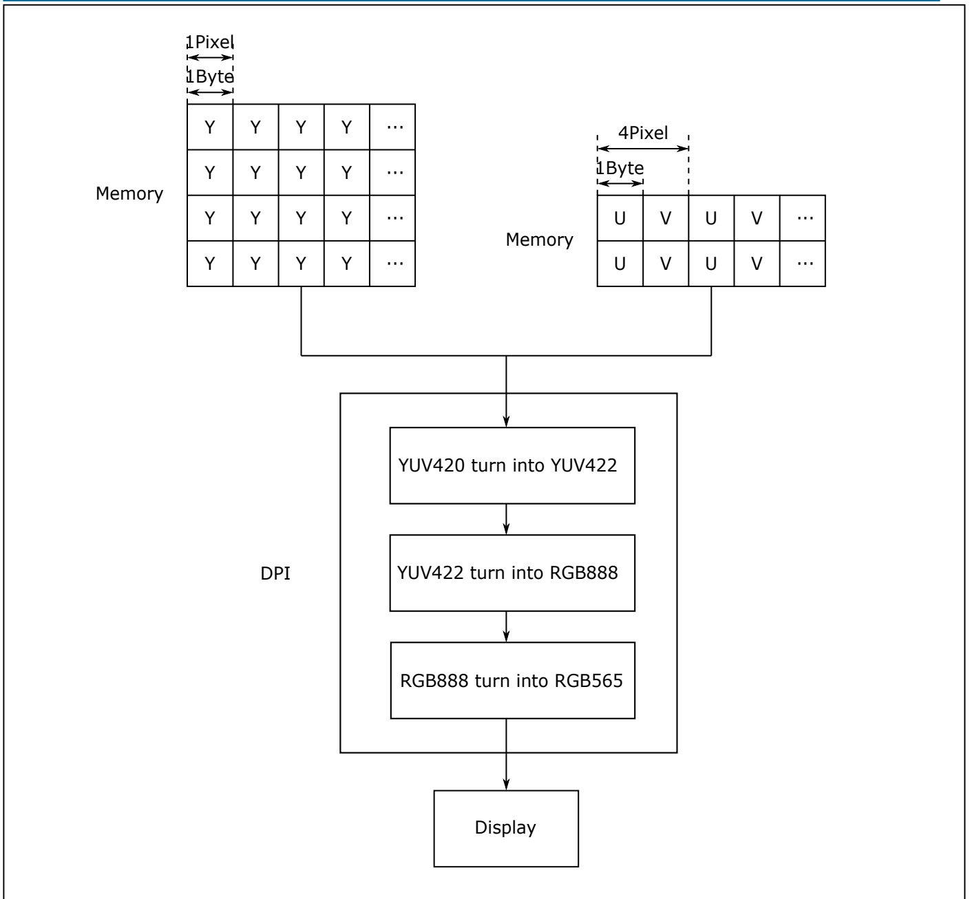
图 11.10: YUV420 处理过程
