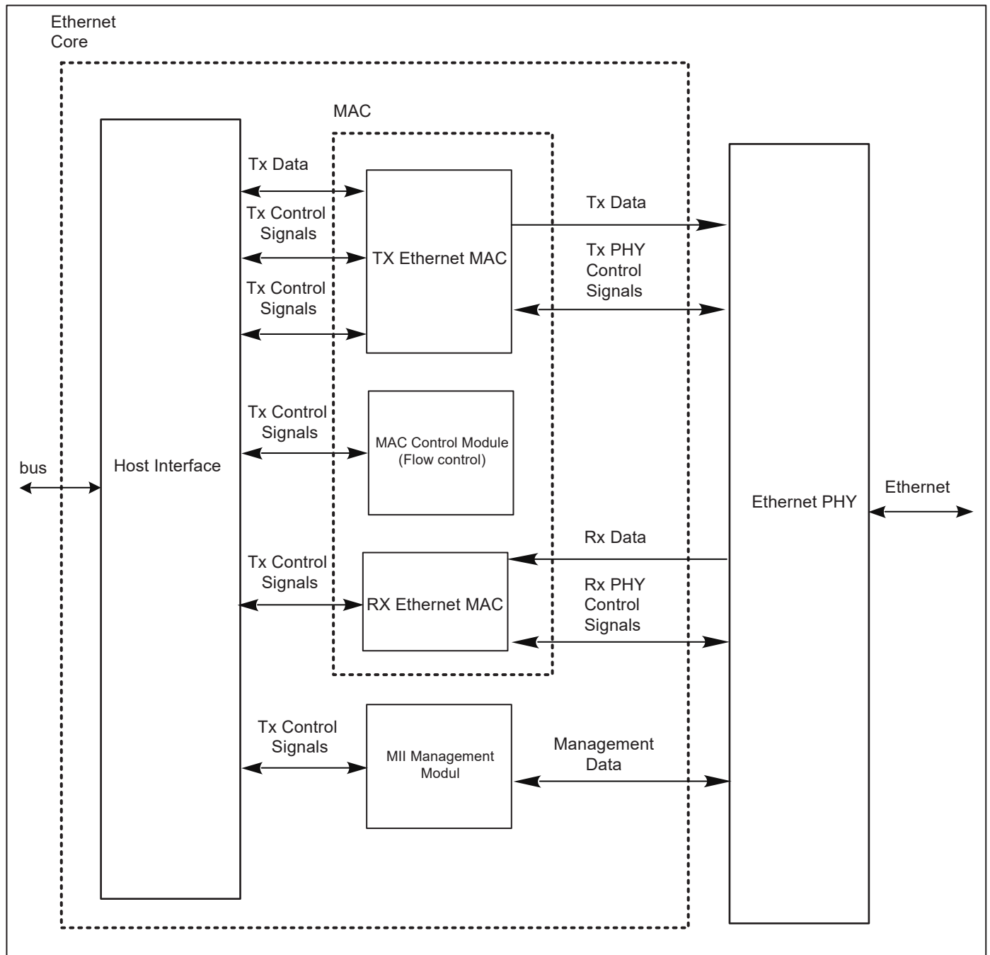
图 24.1: EMAC 框图
