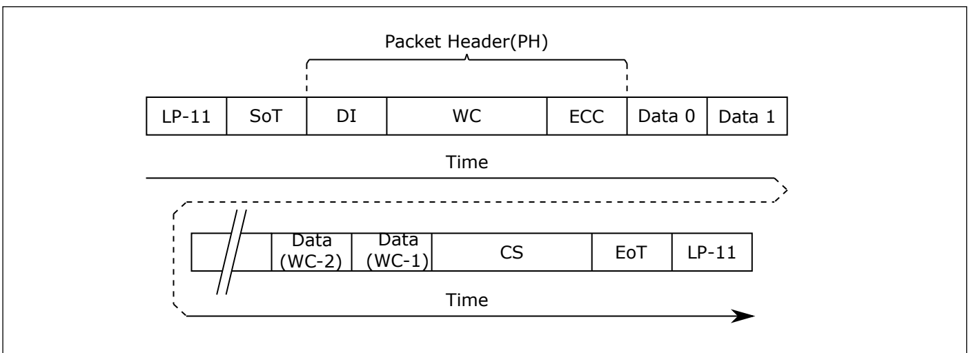
图 12.25: 长数据包结构图
