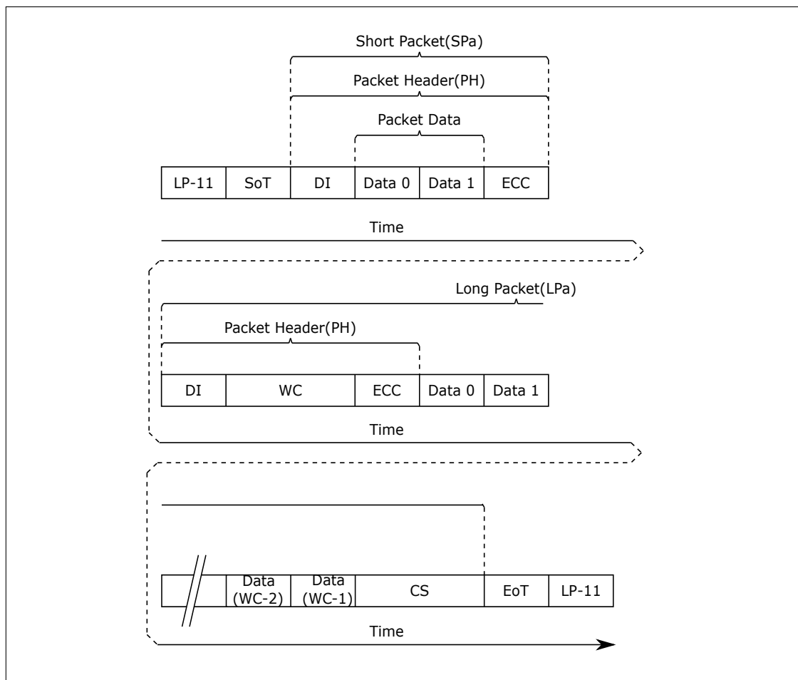
图 12.26: 一次传输多个数据包
