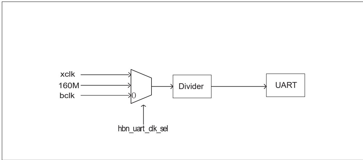
图 16.3: UART 时钟
