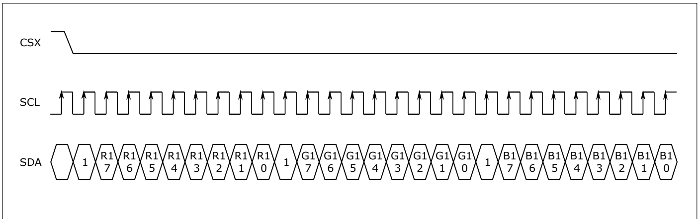
图 10.11: RGB888 输出
