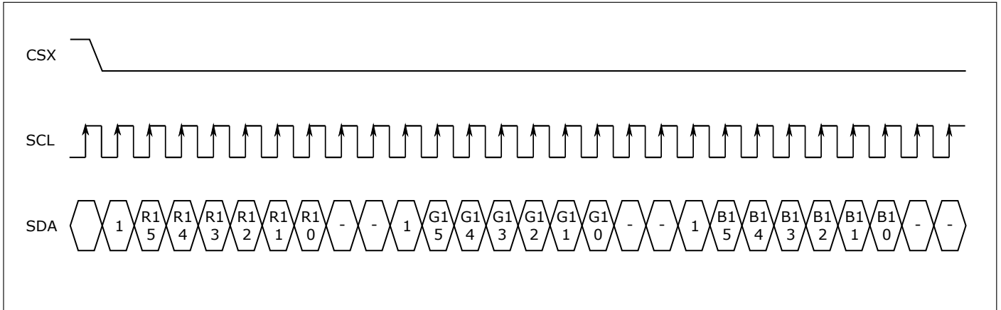
图 10.10: RGB666 输出
