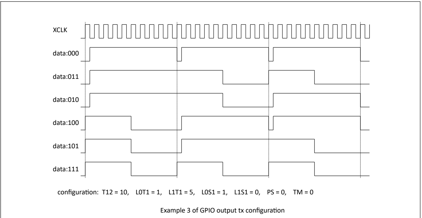
图 4.3: 默认电平为低电平，逻辑 0 电平翻转输出波形
