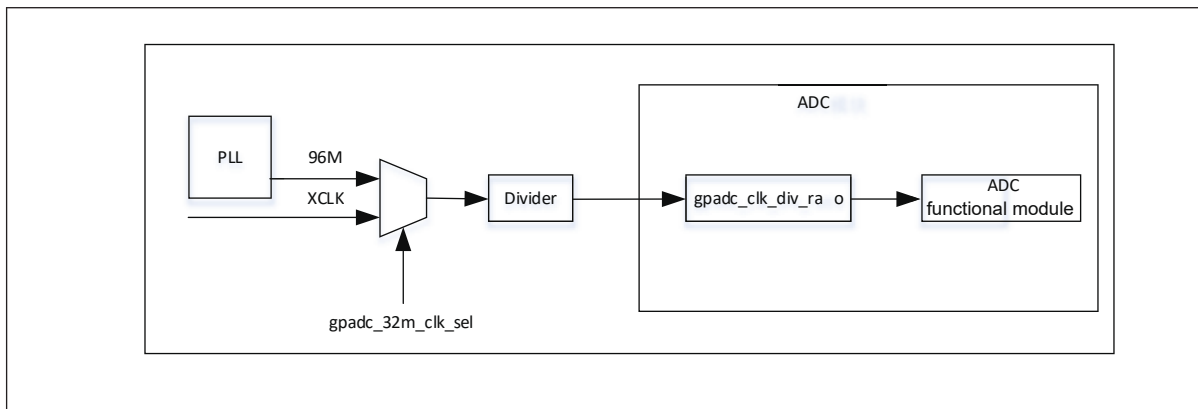
图 5.2: ADC 时钟
