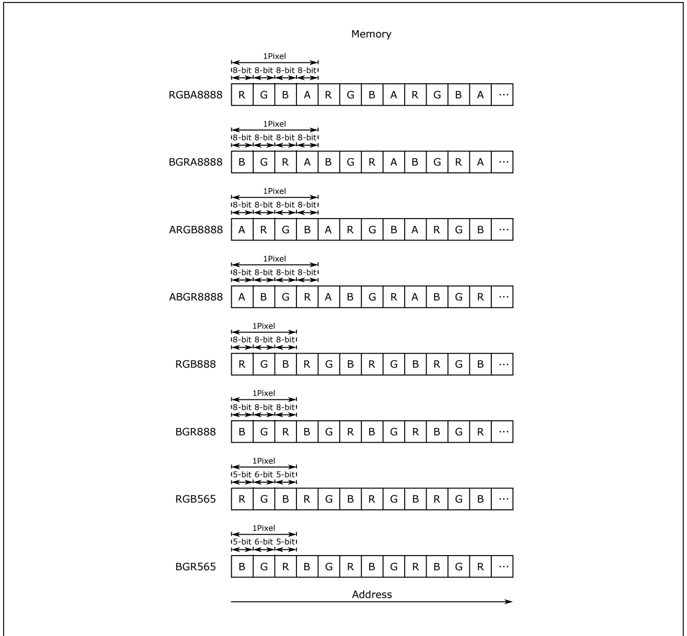
图 10.17: 输入像素格式
