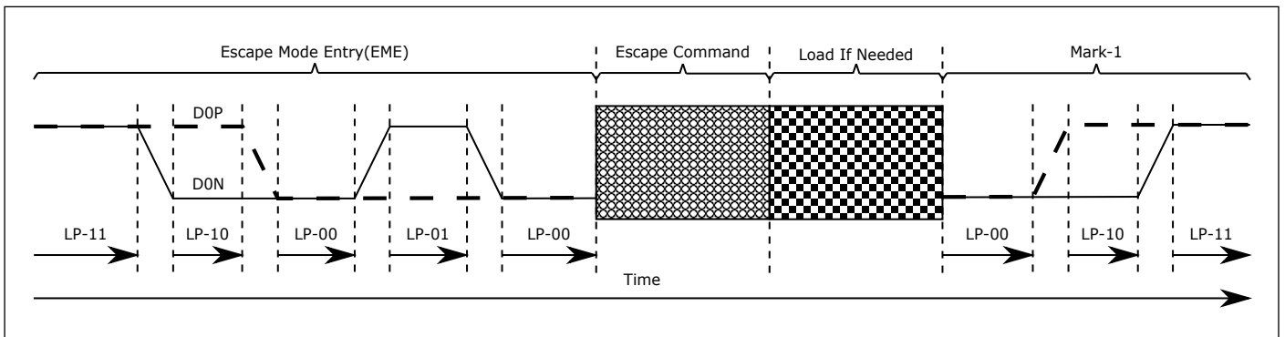
图 12.15: Escape 模式序列
