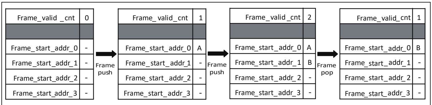
图 13.3: FIFO 框架
