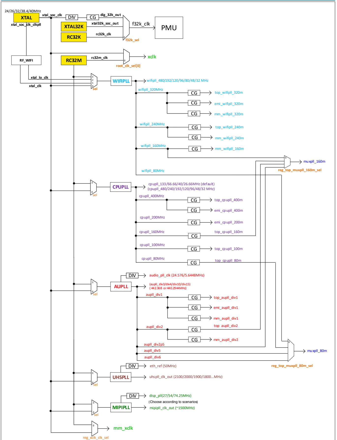
图 2.1: 系统时钟架构
