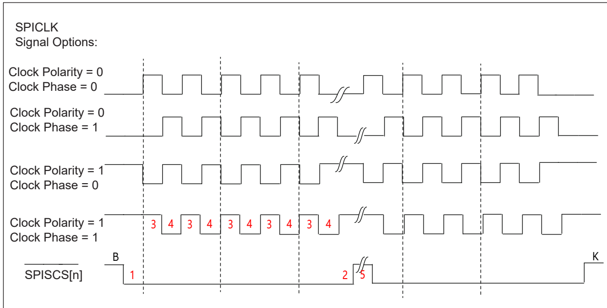
图 15.1: SPI 时序图
