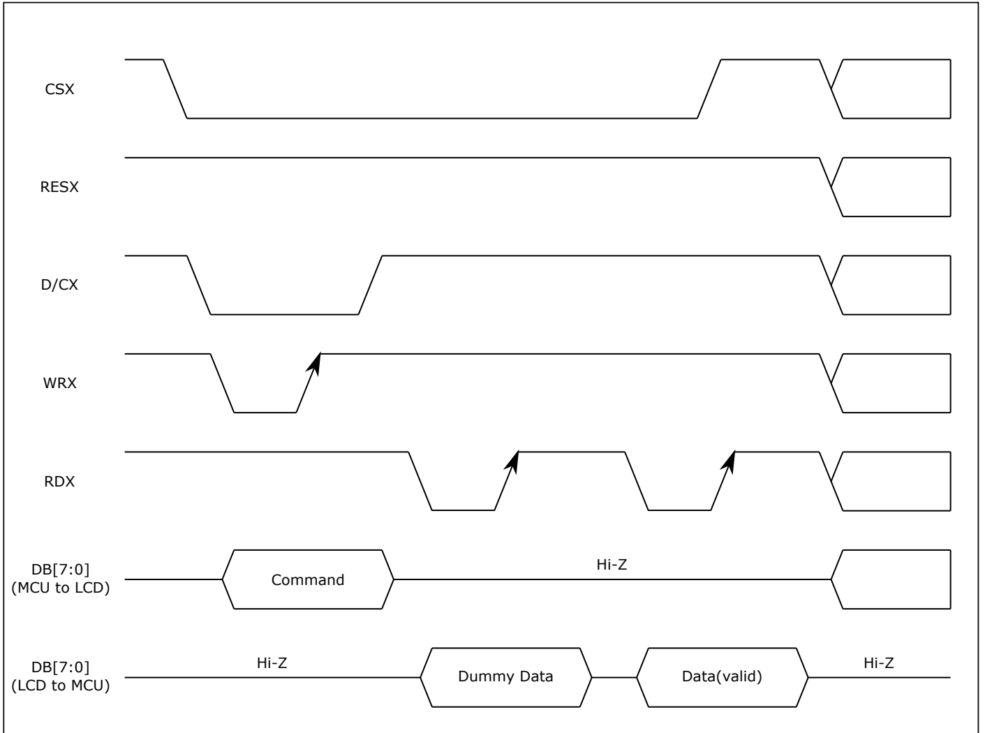
图 10.3: 读时序
