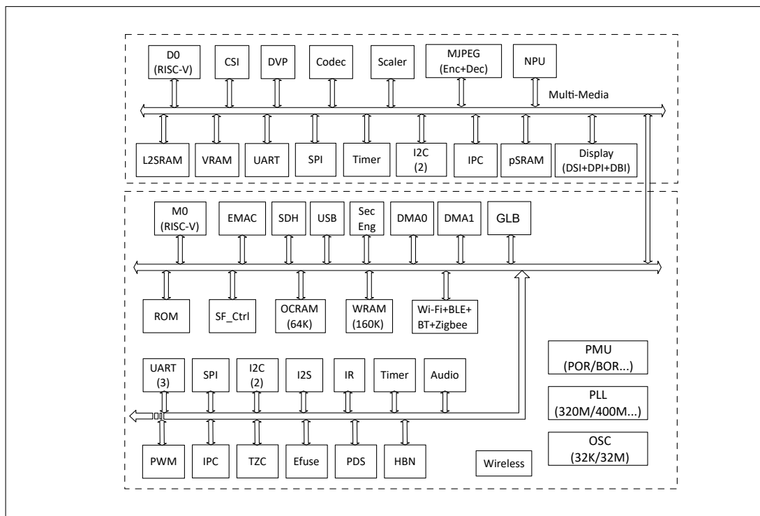
图 1.1: 系统框图
