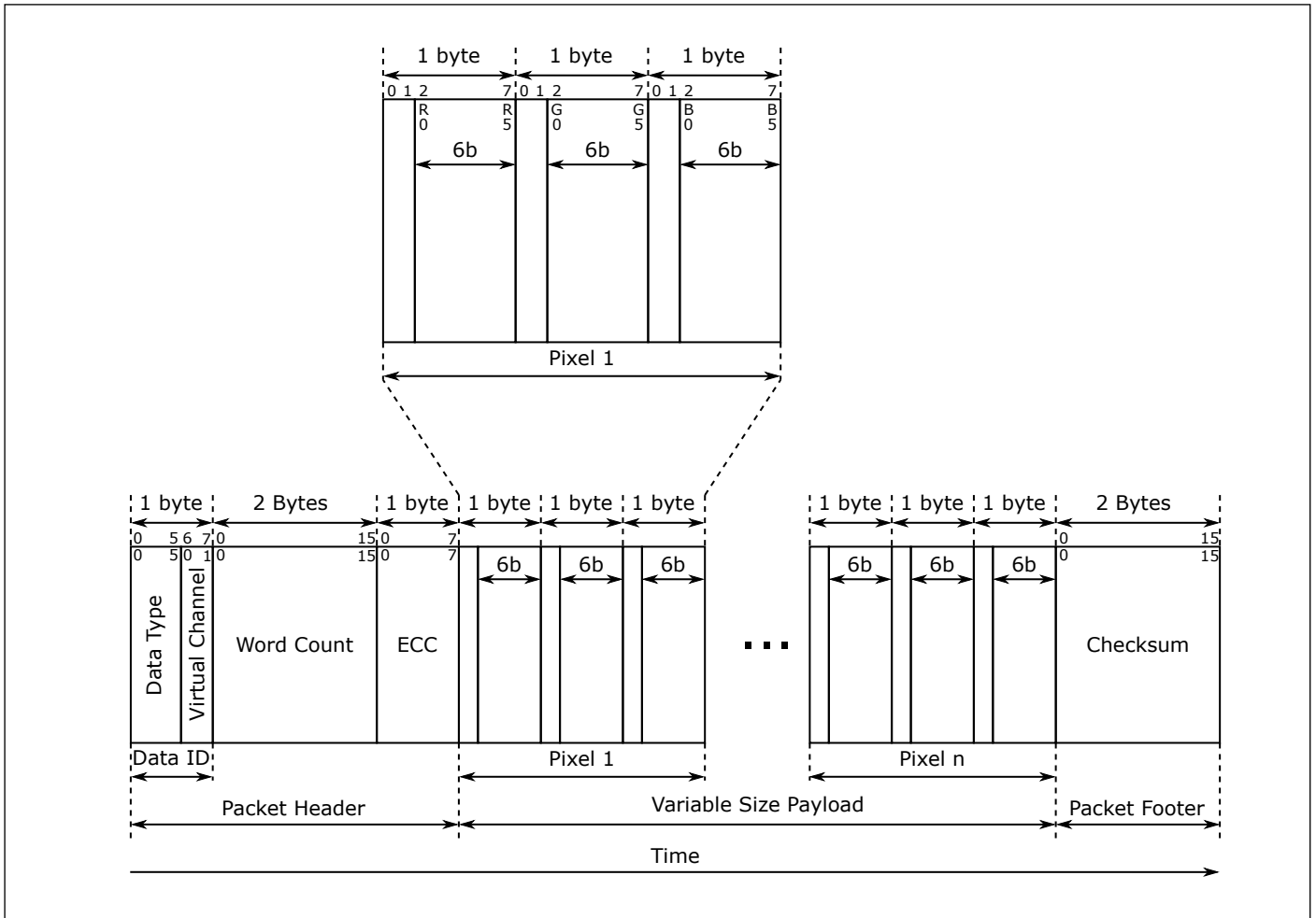
图 12.39: RGB666 像素格式
