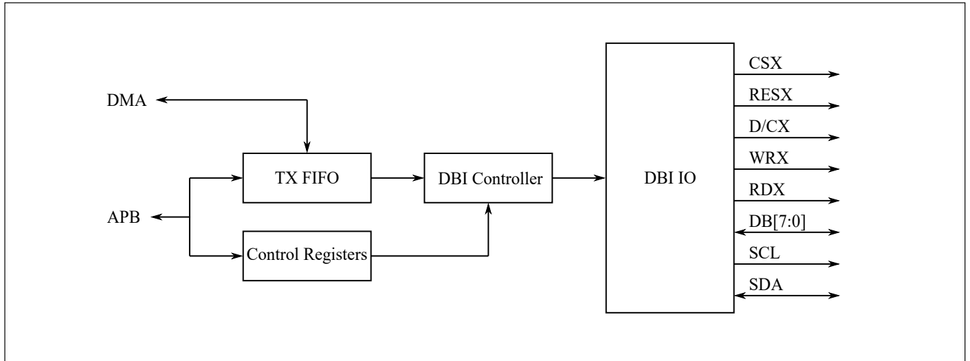
图 10.1: DBI 基本框图
