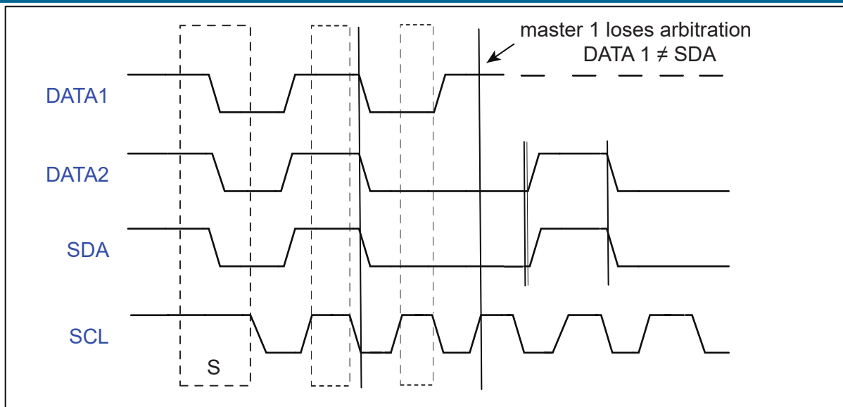
图 17.5: 同时传输数据波形示意图
