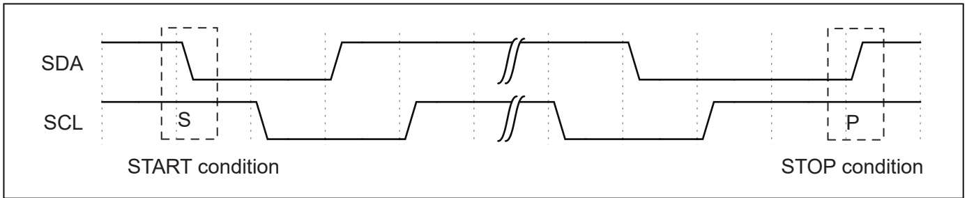
图 17.1: I2C 起始和停止条件
