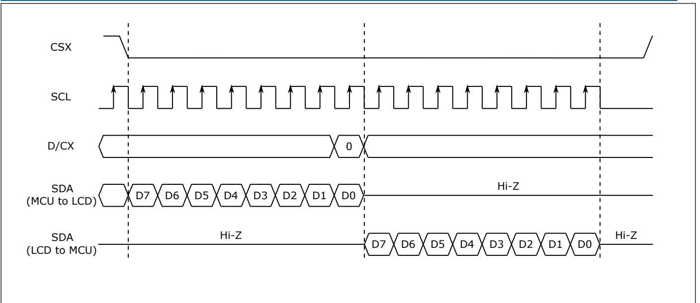
图 10.13: 读时序
