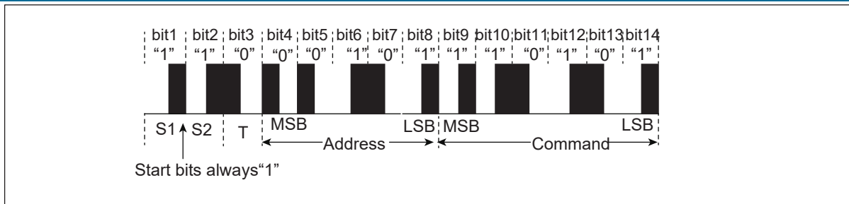
图 14.4: RC5 协议波形
