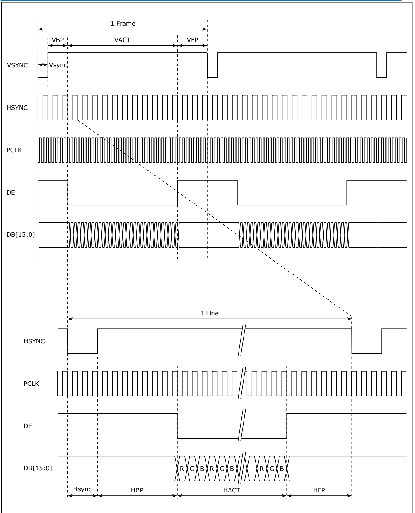
图 11.2: DPI 时序图
