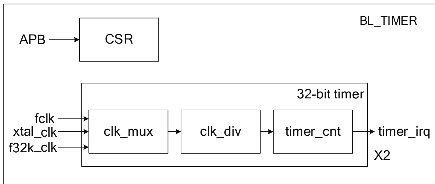
图 19.1: 定时器框图
