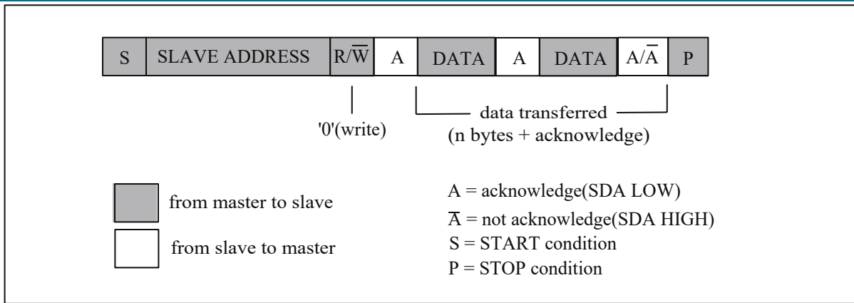
图 17.3: 主发送和从接收的时序
