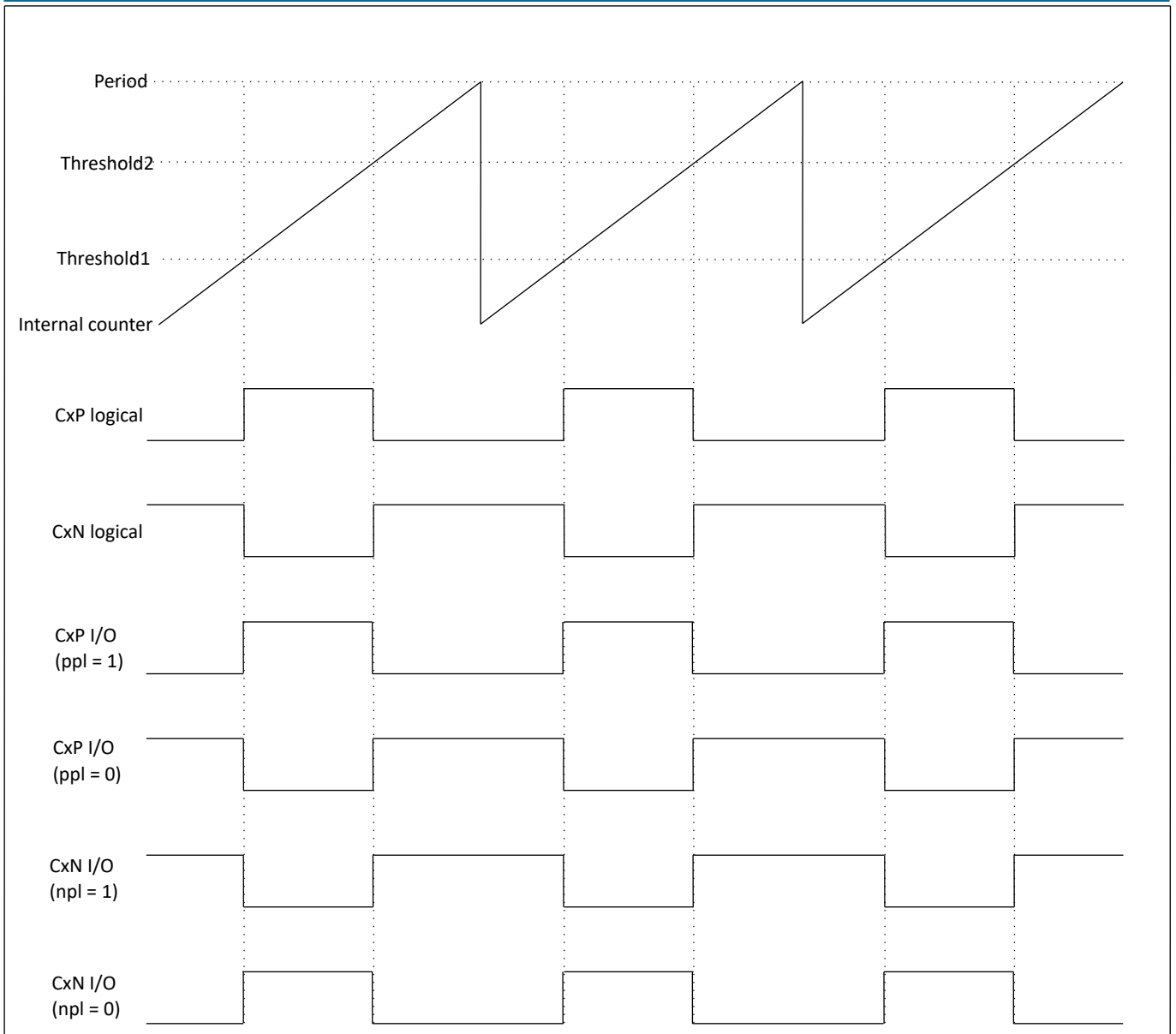
图 18.1: PWM 在不同配置下的波形图
