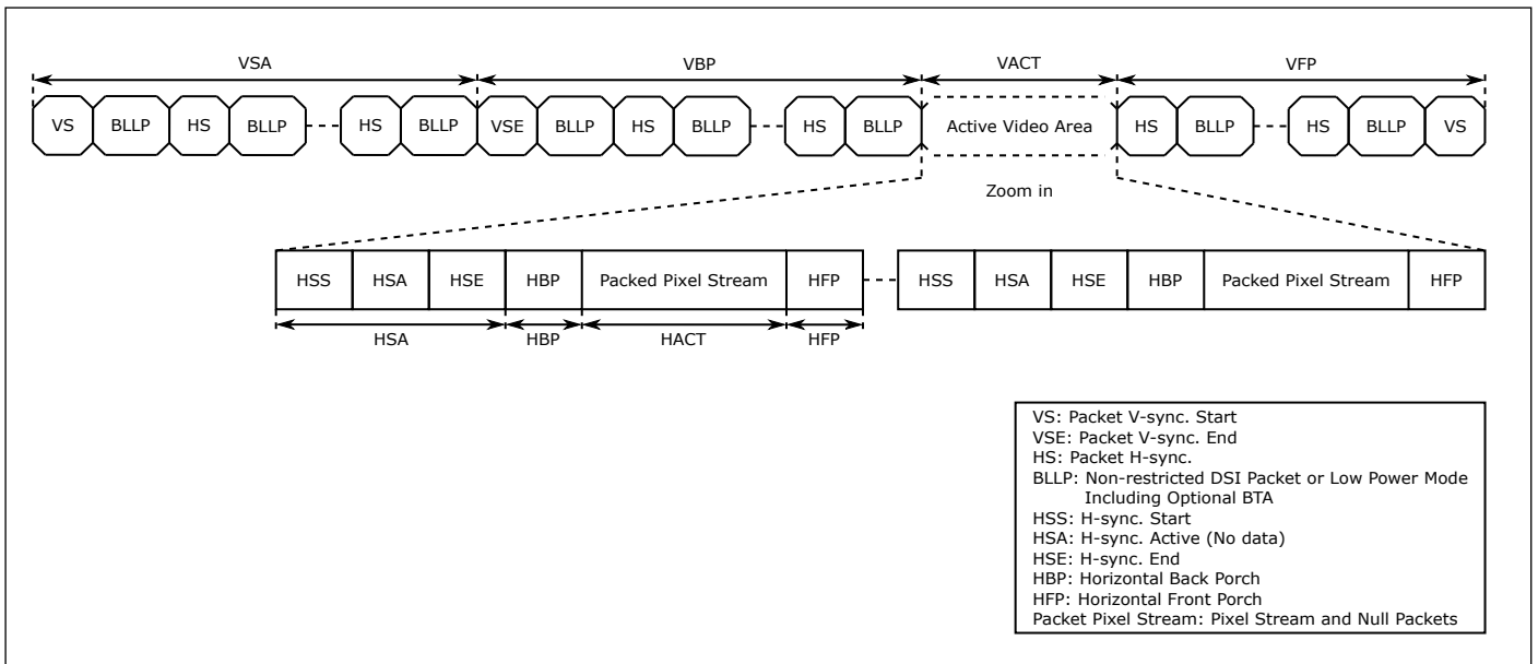
图 12.34: 具有同步脉冲的非突发模式时序图
