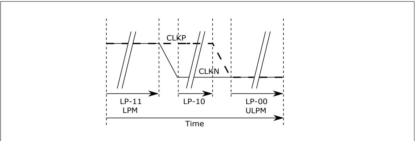
图 12.8: 由低功耗模式进入超低功耗模式
