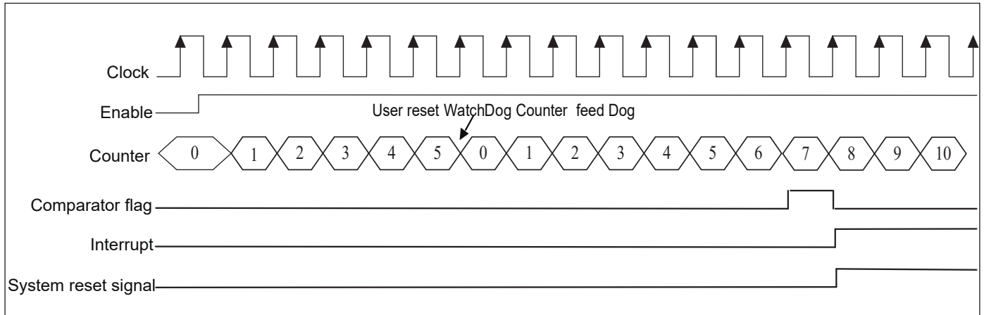
图 19.4: Watchdog 工作时序
