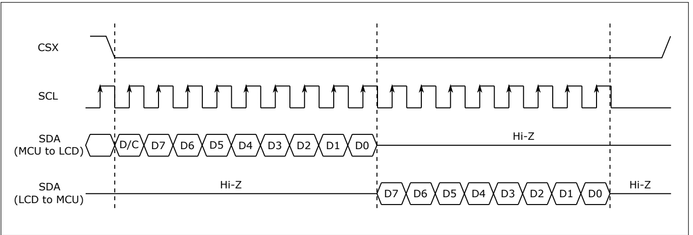
图 10.8: 读时序
