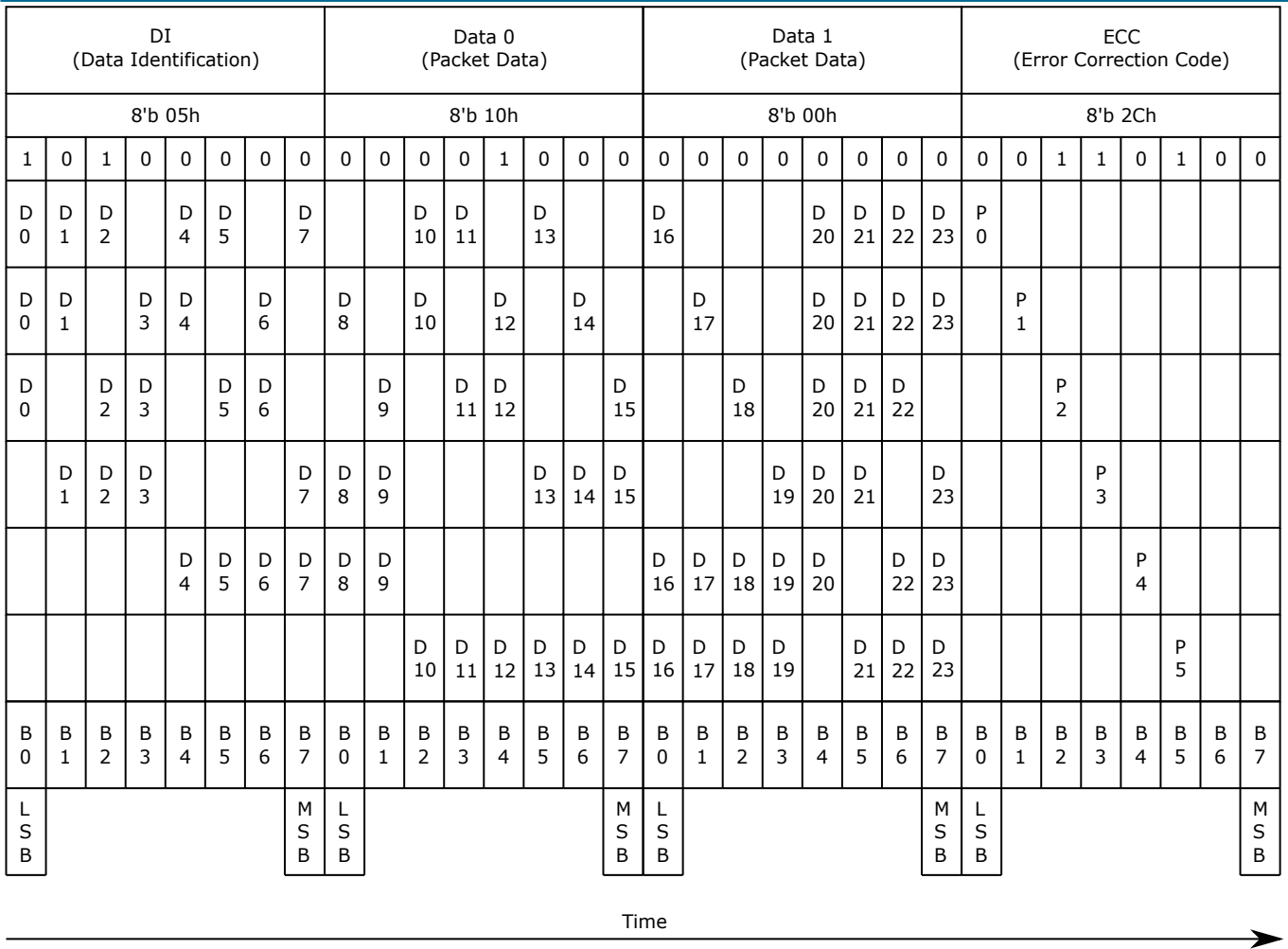
图 12.31: ECC 计算示例
