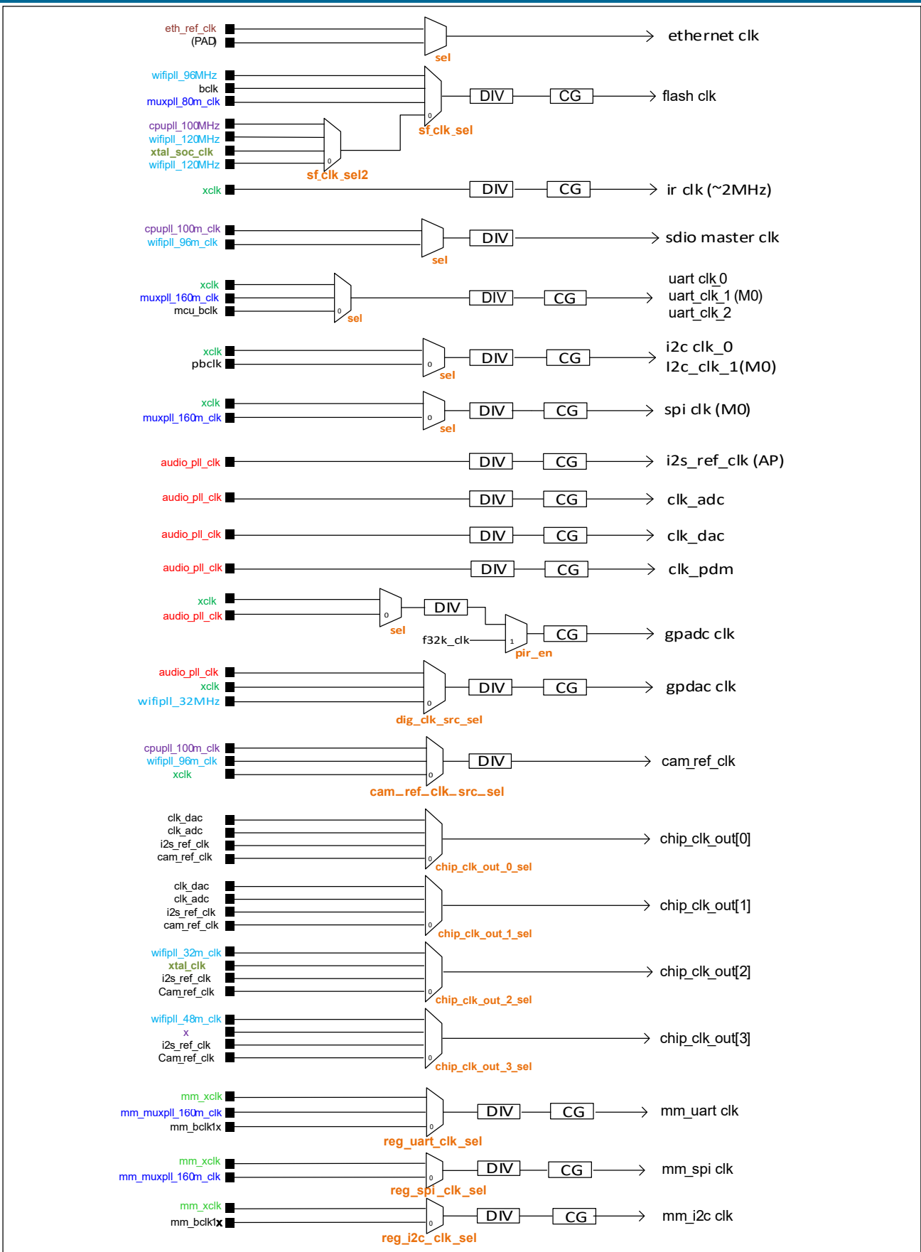
图 2.3: 外设时钟架构
