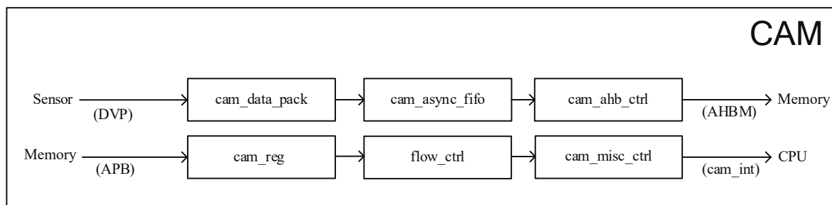
图 13.1: Cam 框图
