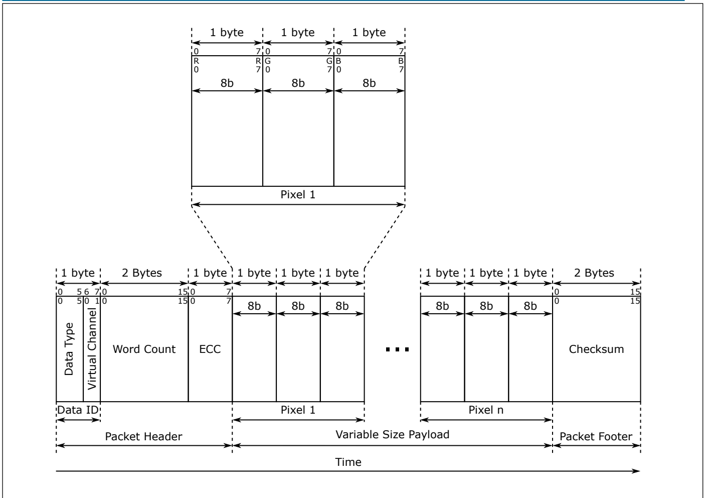
图 12.40: RGB888 像素格式
