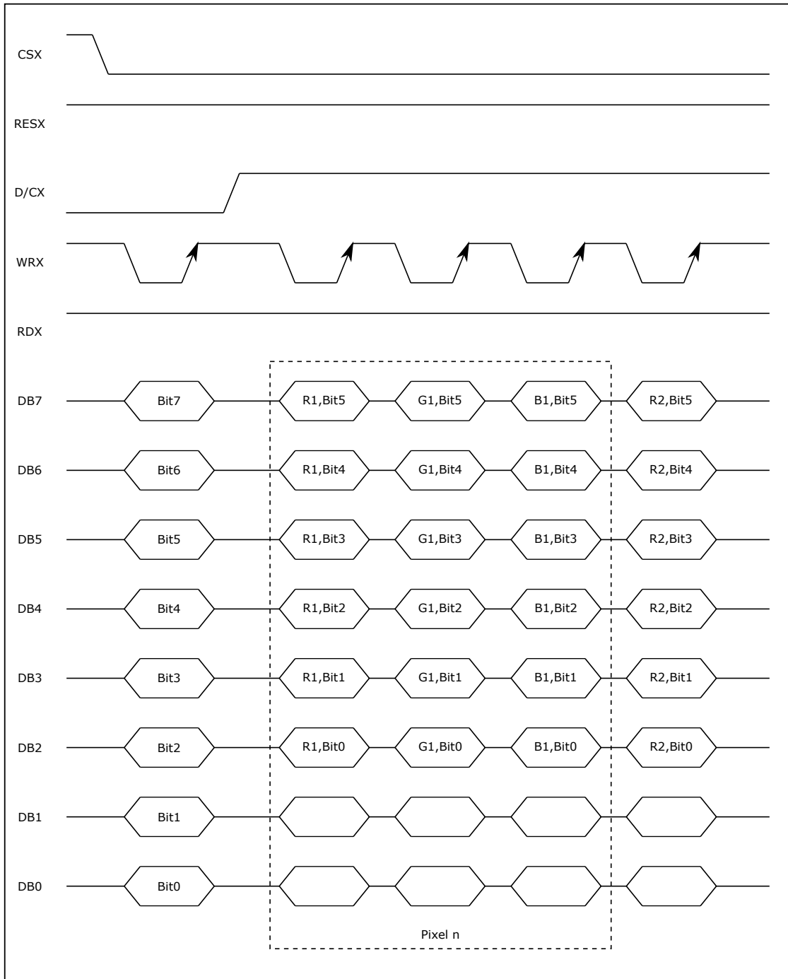
图 10.5: RGB666 输出
