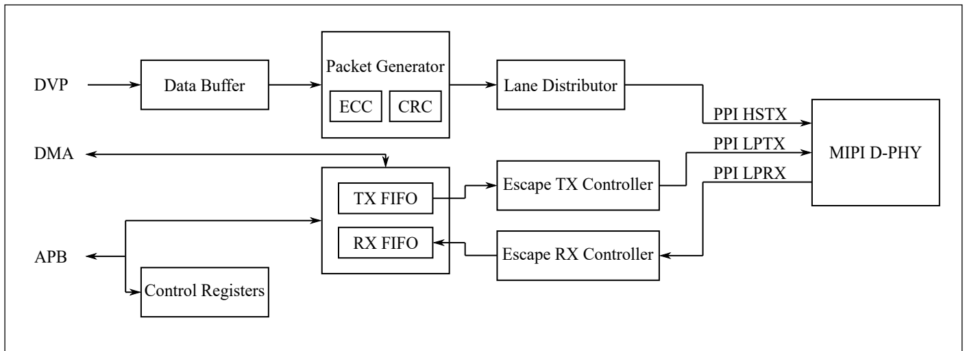
图 12.1: DSI 基本框图
