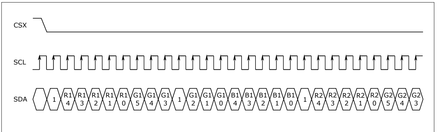
图 10.9: RGB565 输出
