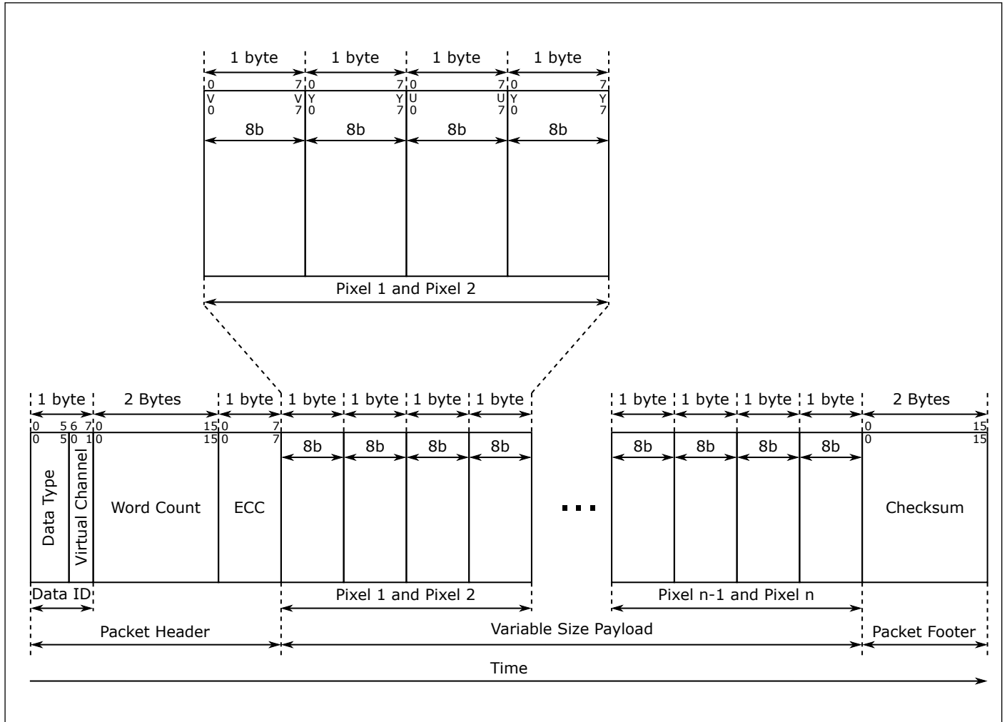
图 12.37: YUV422 像素格式
