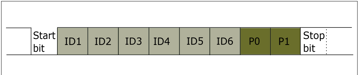
图 16.11: LIN 的 ID 域
