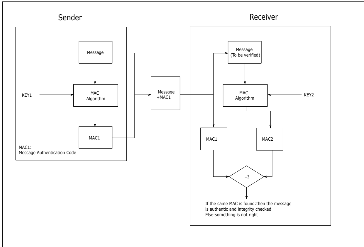
图 34.3: 消息认证码流程图
