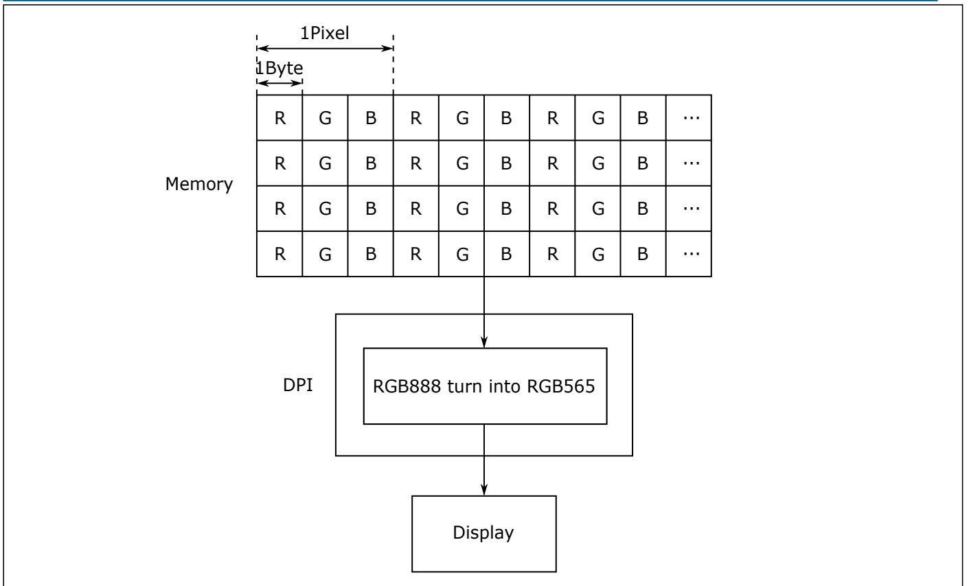
图 11.7: RGB888 处理过程
