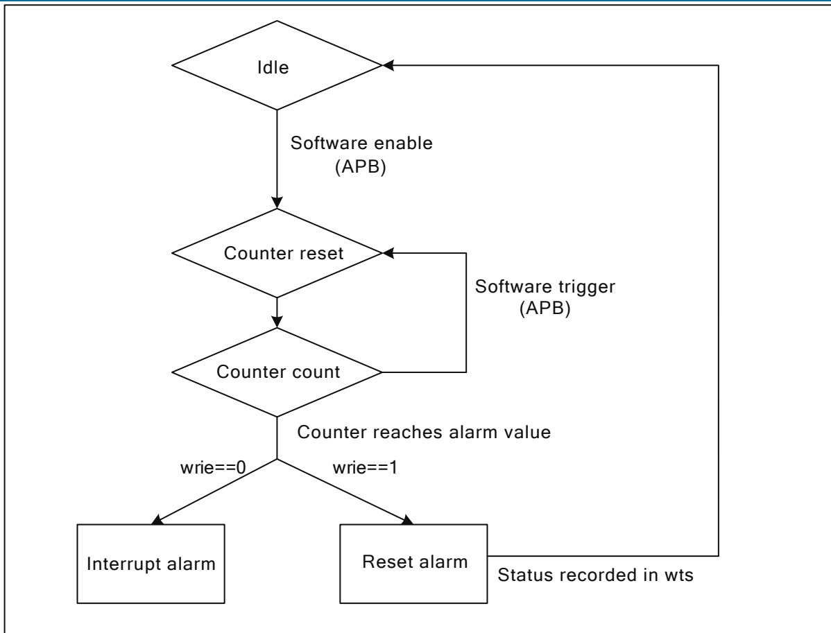
图 19.5: 看门狗报警机制
