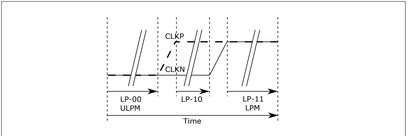
图 12.6: 由超低功耗模式进入低功耗模式
