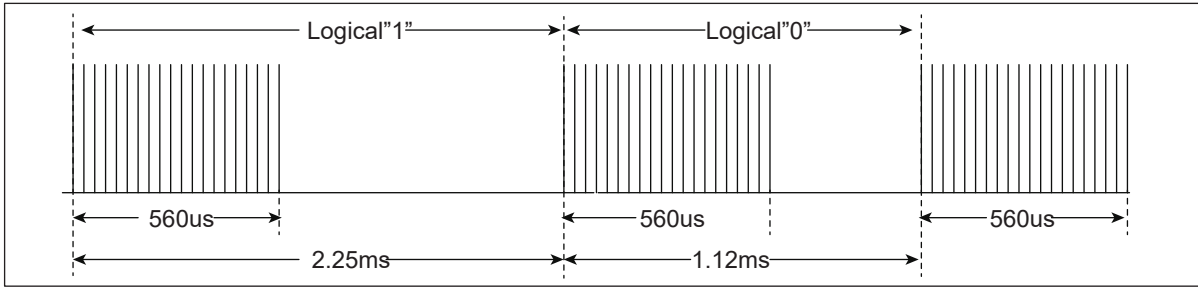
图 14.1: NEC 逻辑波形
