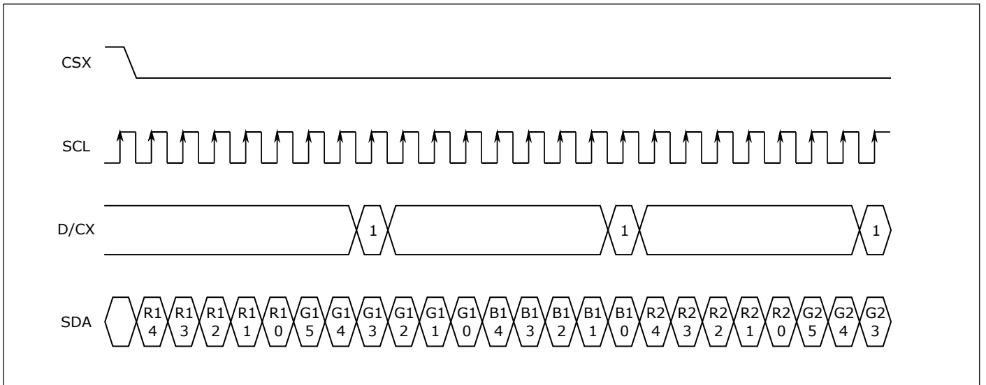
图 10.14: RGB565 输出
