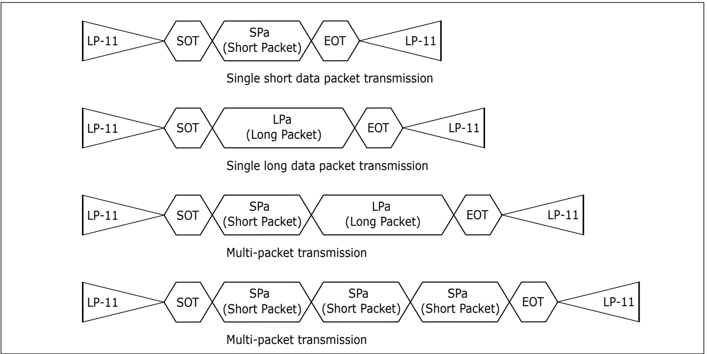
图 12.13: 高速数据传输突发序列
