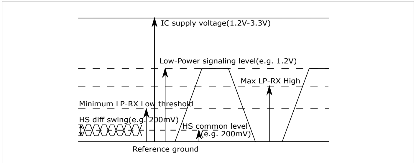
图 12.3: 高速和低功耗模式下的电平
