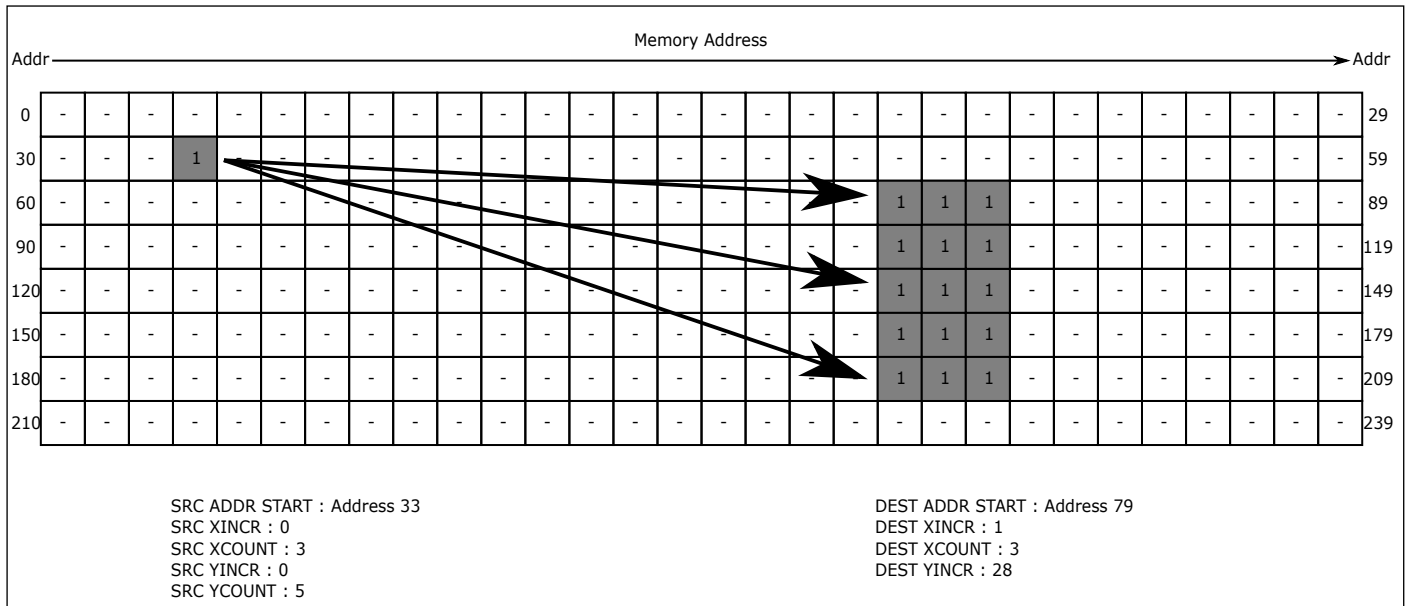
图 8.5: 图像填充
