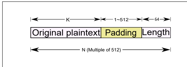
图 34.2: MD5 Padding
