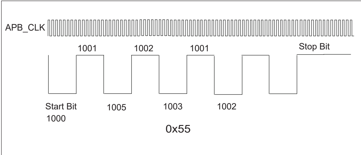
图 16.6: UART 固定字符模式波形图
