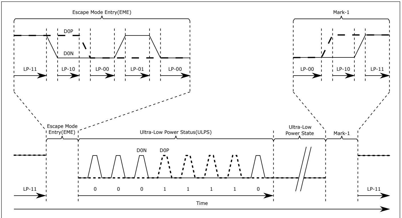
图 12.18: 超低功耗状态序列
