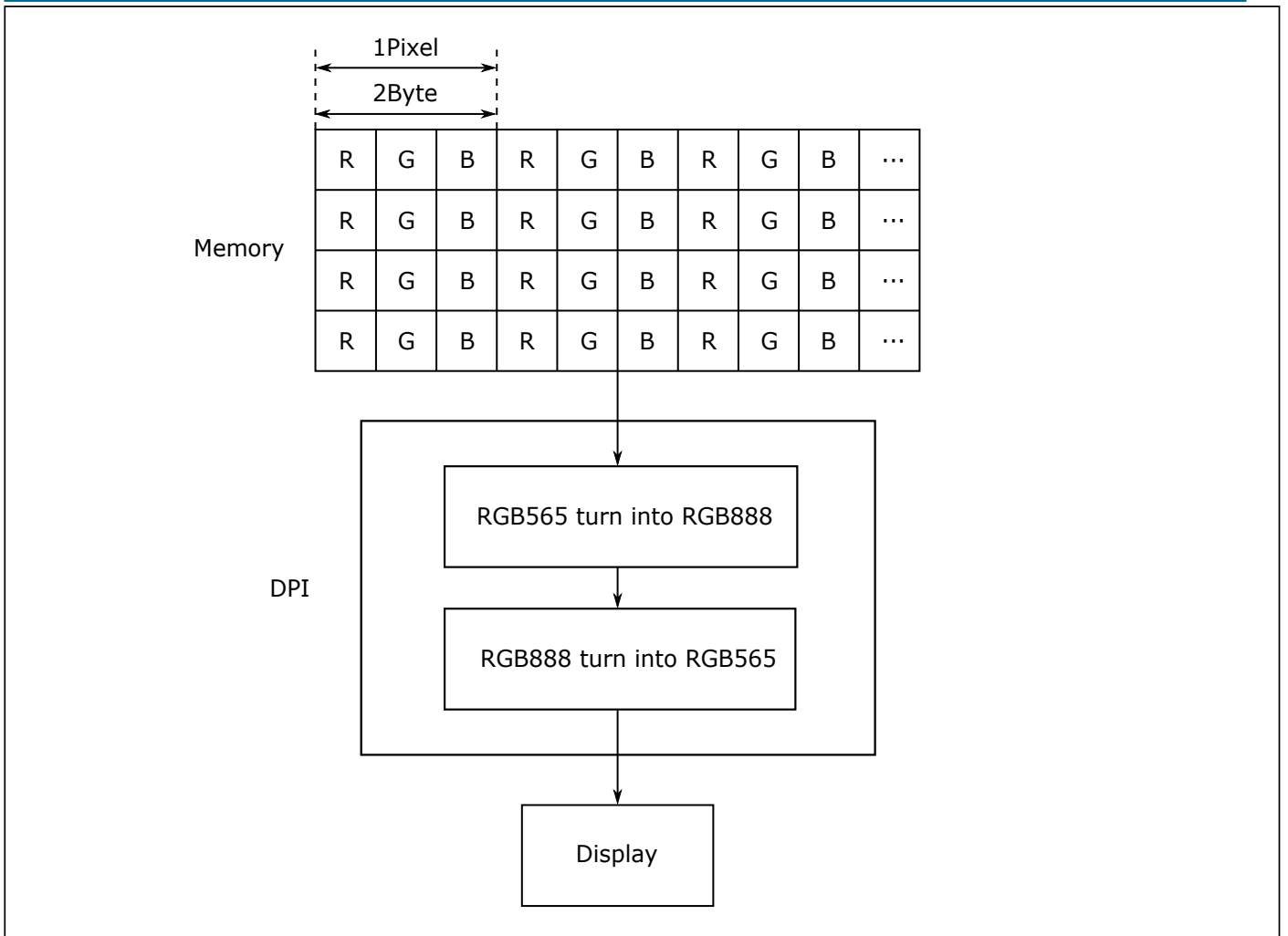
图 11.8: RGB565 处理过程
