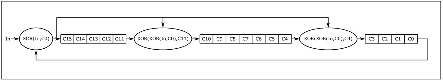
图 12.32: CRC 计算方法
