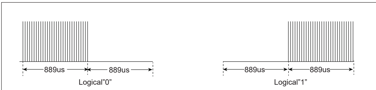
图 14.3: RC5 逻辑波形
