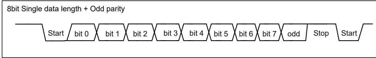
图 16.1: UART 数据格式
