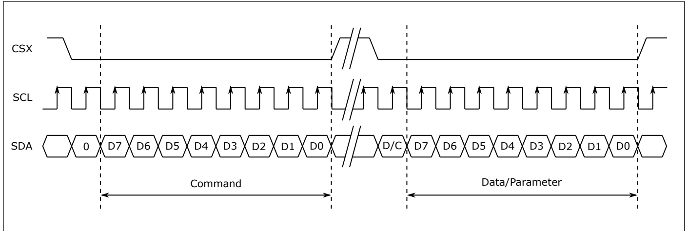
图 10.7: 写时序
