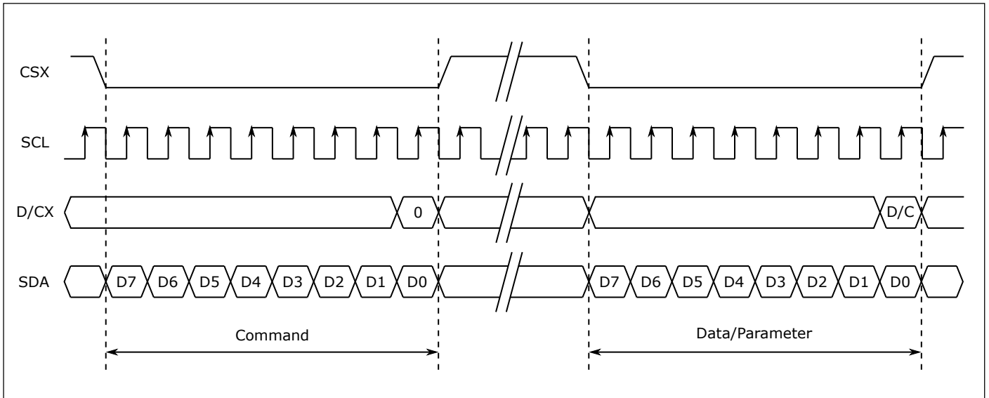
图 10.12: 写时序
