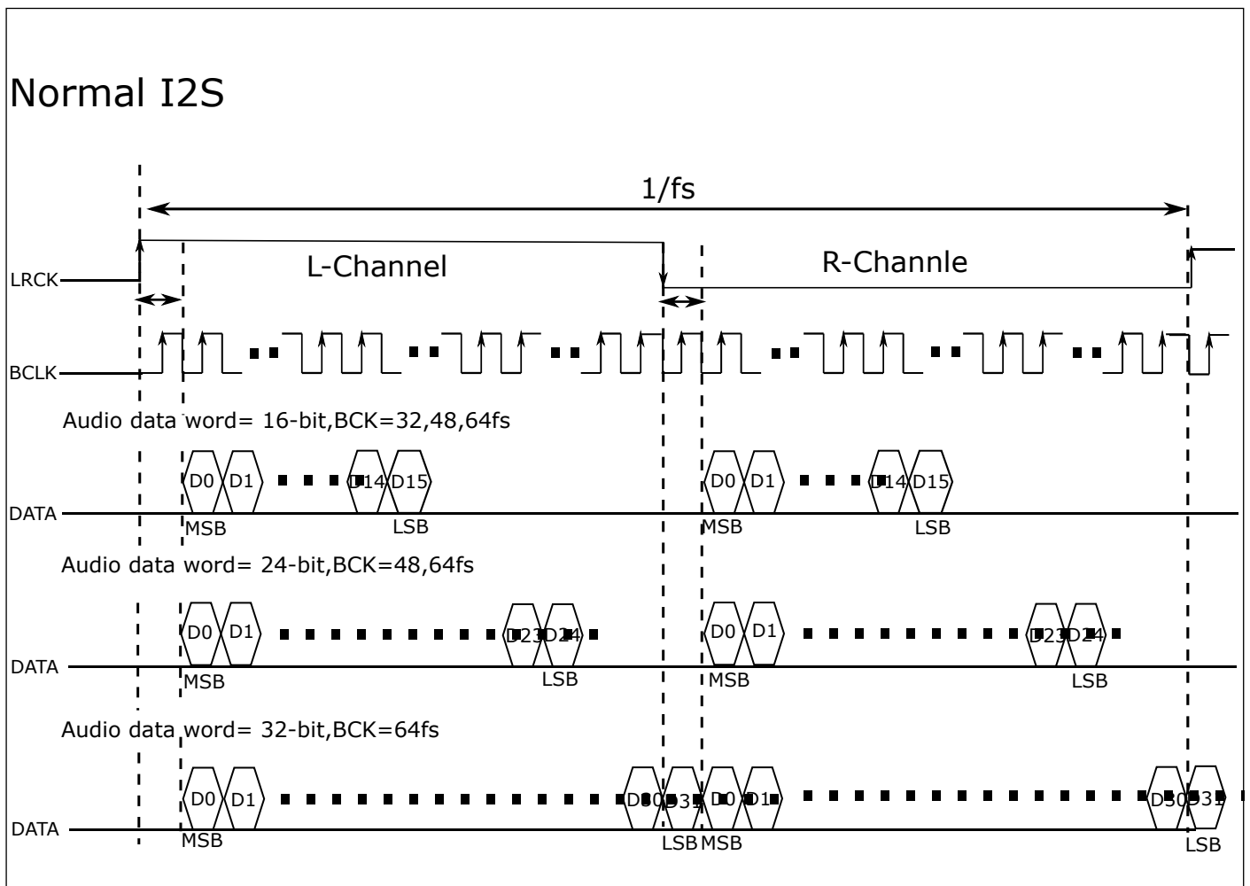
图 20.1: 标准 I2S 数据格式
