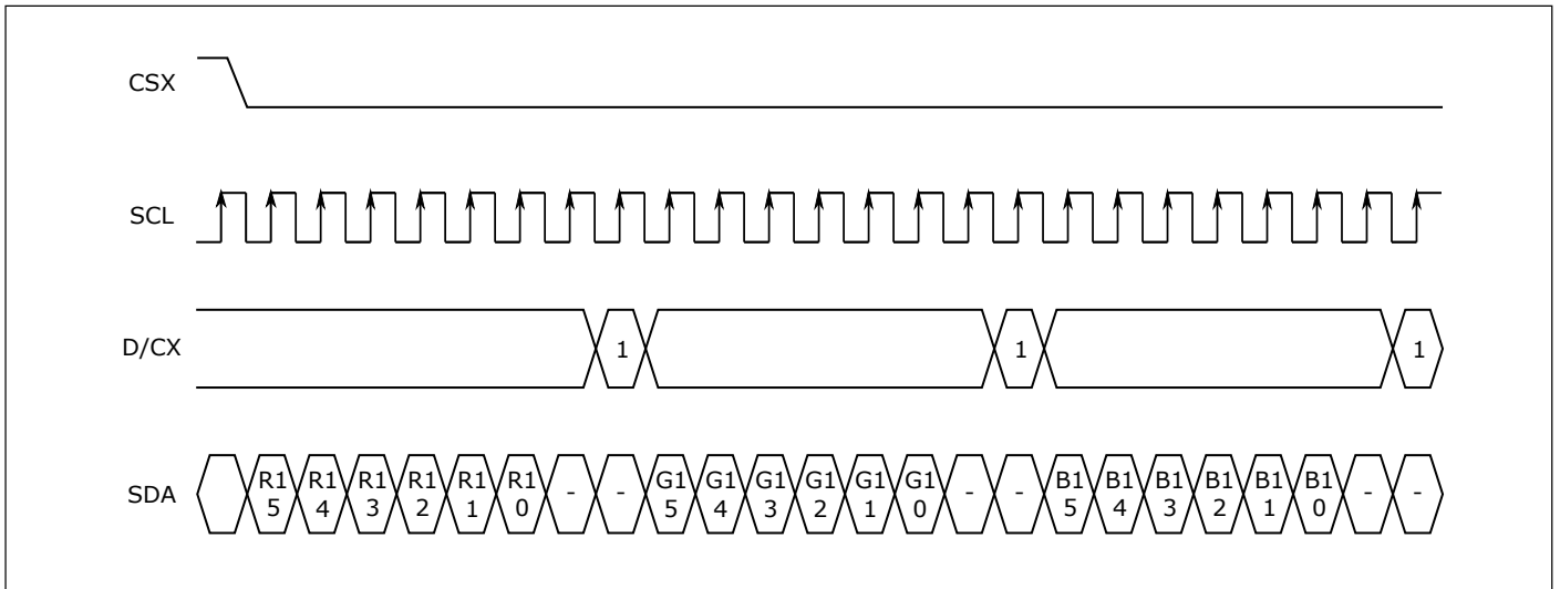
图 10.15: RGB666 输出
