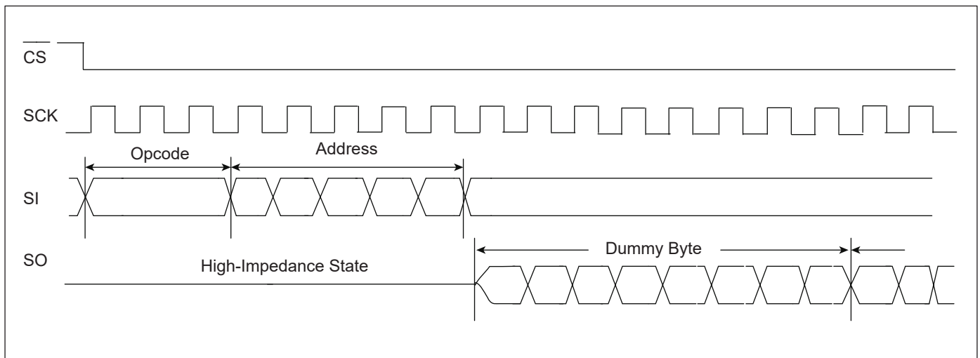
图 15.2: SPI Ignore 波形图
