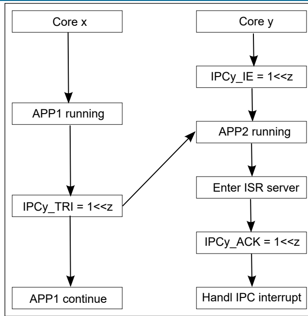
图 32.1: IPC 流程图
