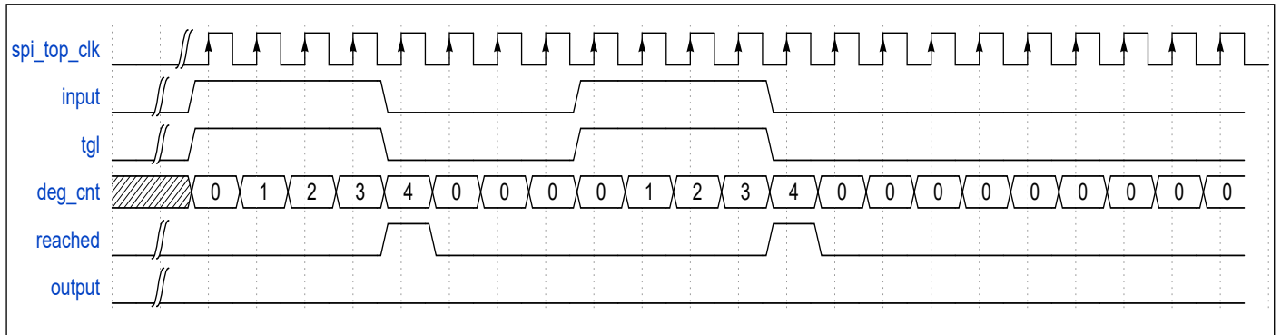
图 15.3: SPI 滤波波形图
