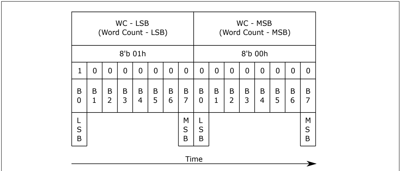
图 12.28: 数据包的字节顺序
