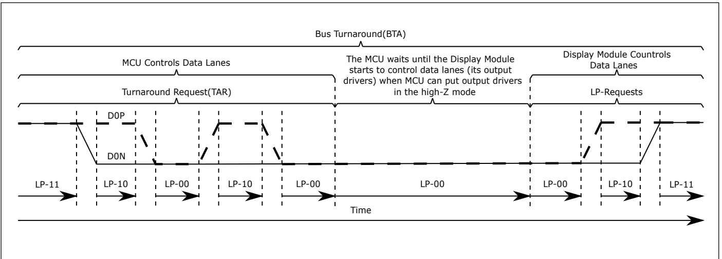
图 12.14: 总线反转序列
