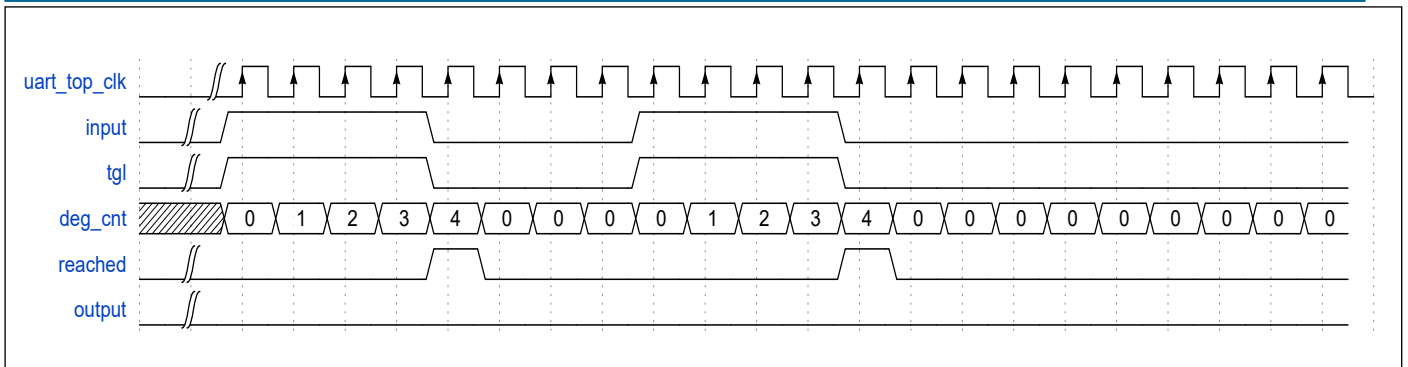
图 16.5: UART 滤波波形图
