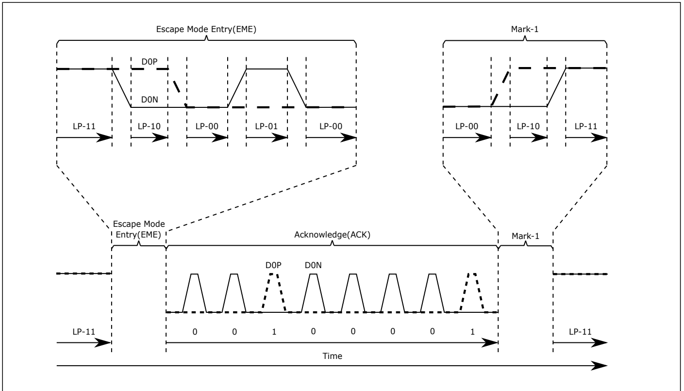
图 12.20: 应答序列
