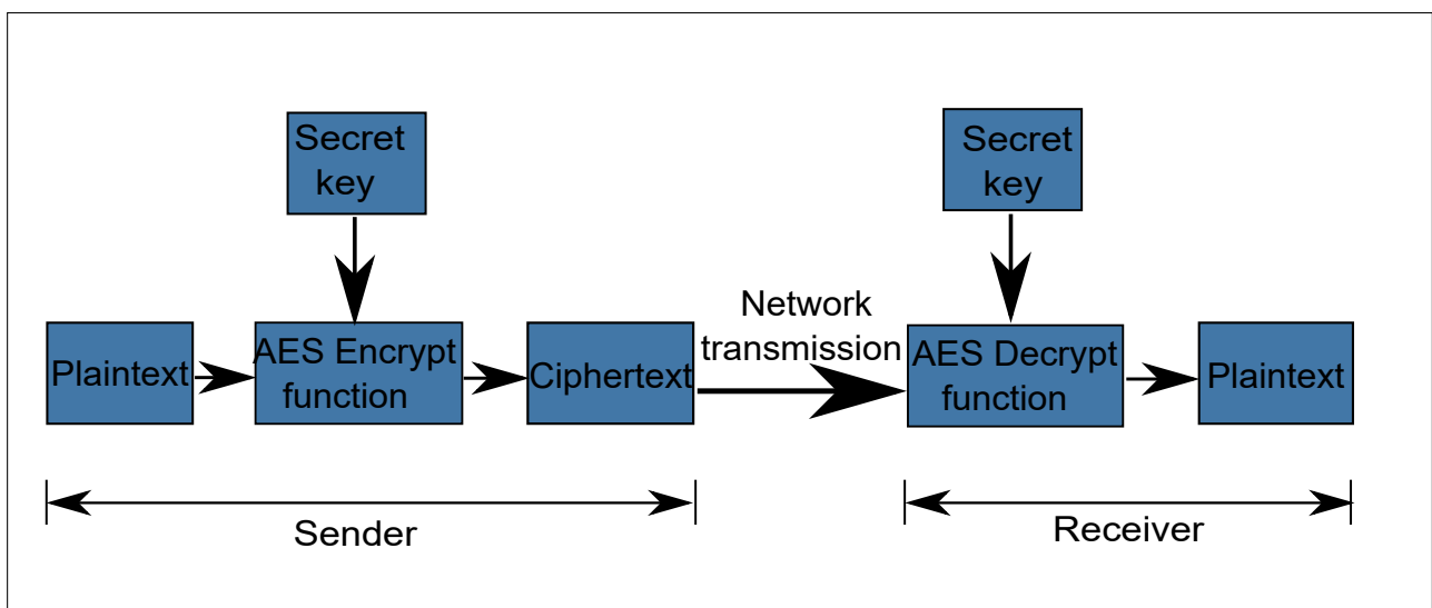
图 34.1: AES 加密流程图
