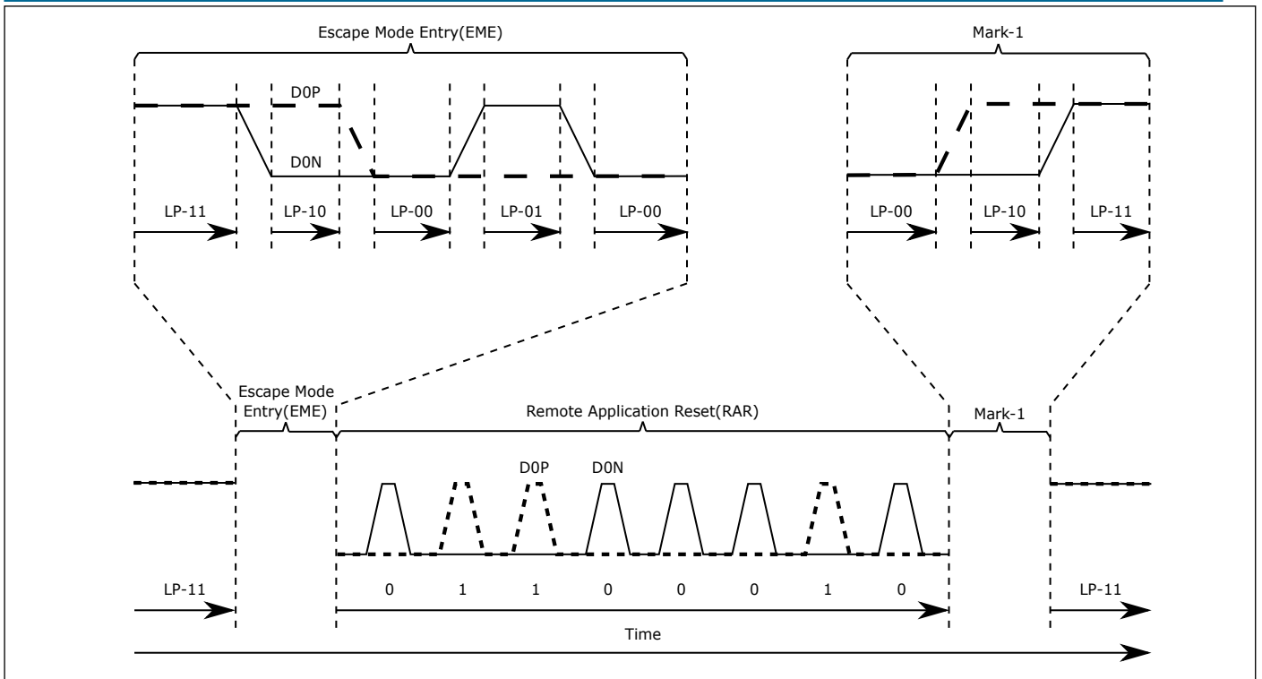
图 12.19: 远程复位序列
