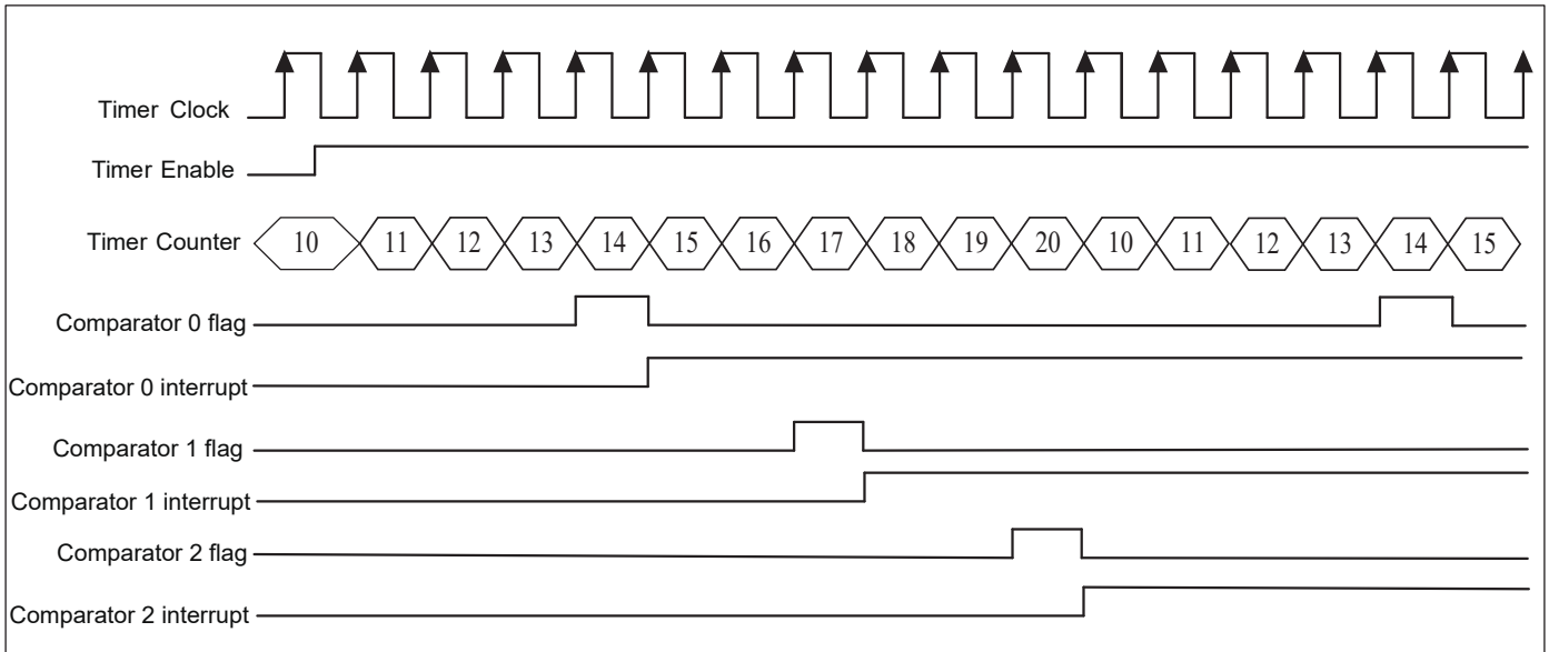
图 19.3: 定时器在 PreLoad 模式下工作时序
