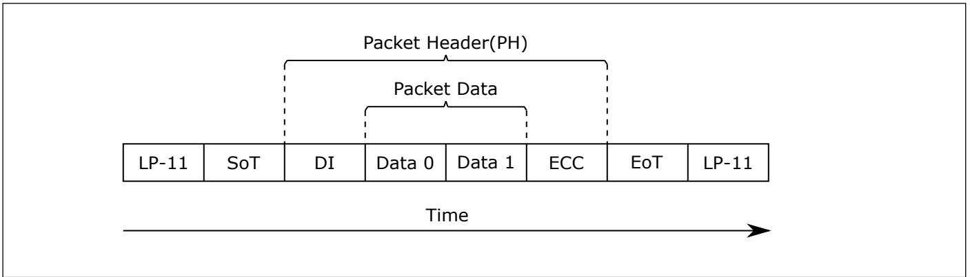
图 12.24: 短数据包结构图
