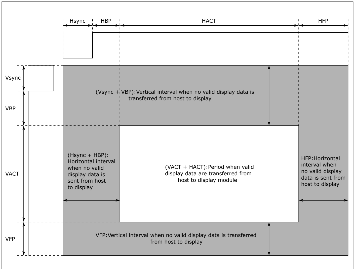
图 11.3: 定时参数图
