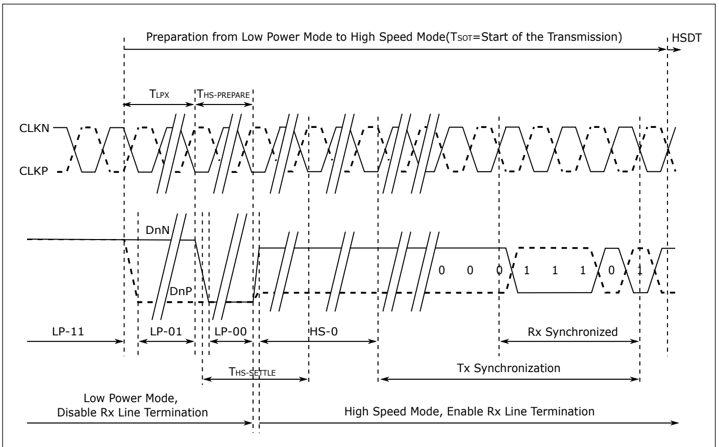
图 12.11: 高速数据传输进入序列
