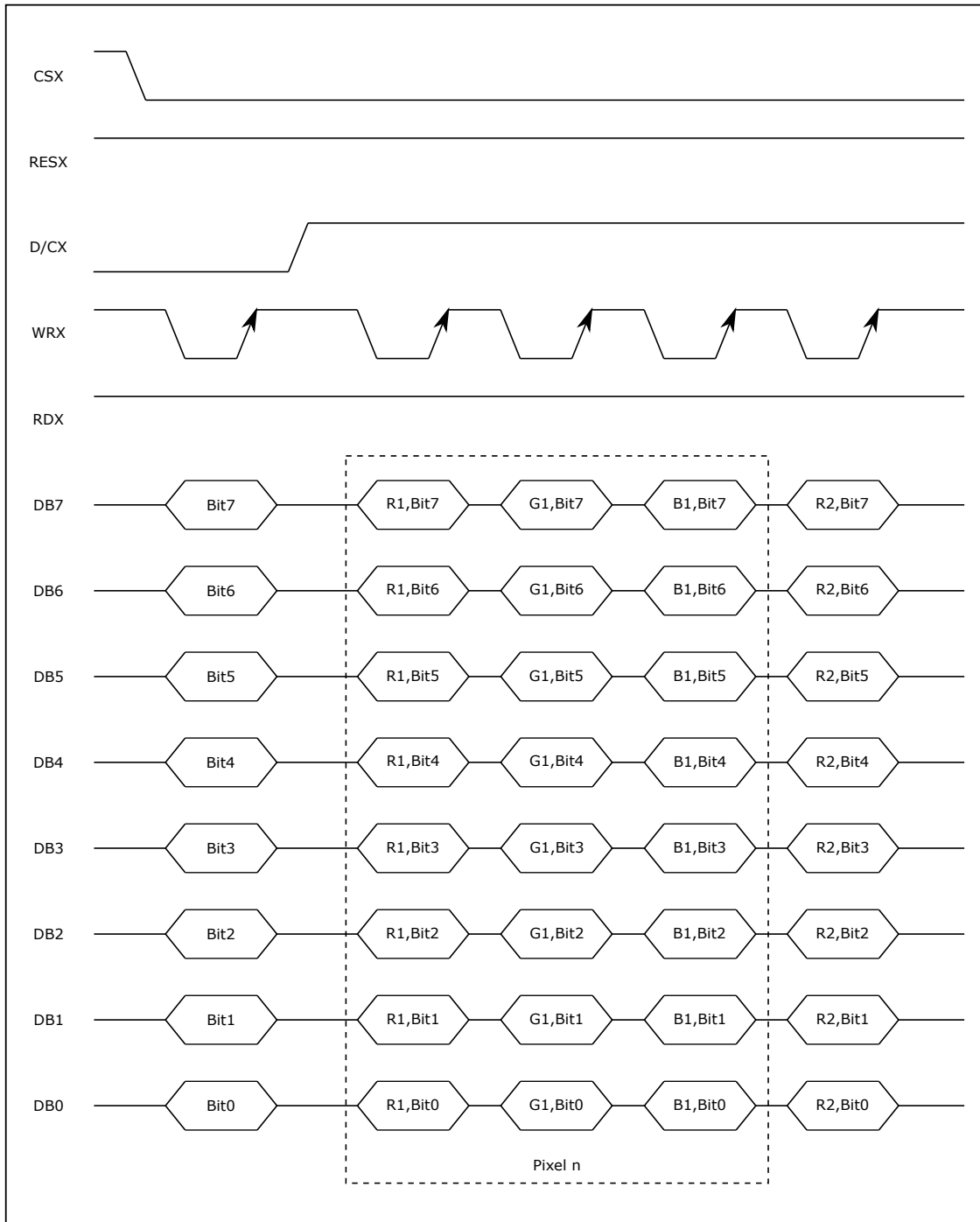
图 10.6: RGB888 输出
