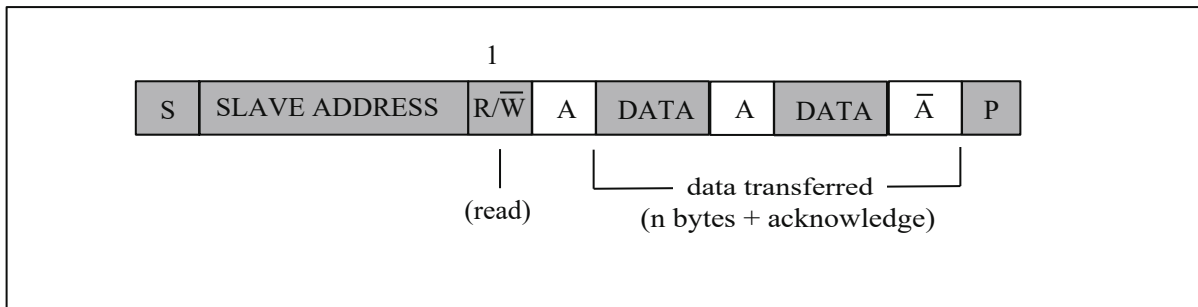
图 17.4: 主接收和从发送的时序
