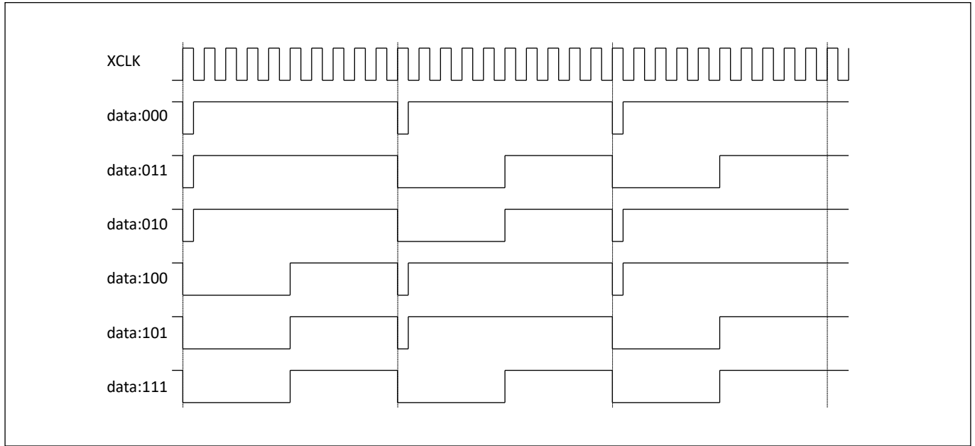
图 4.4: 默认电平为高电平, 逻辑 0 电平翻转, 逻辑 1 电平翻转输出波形
