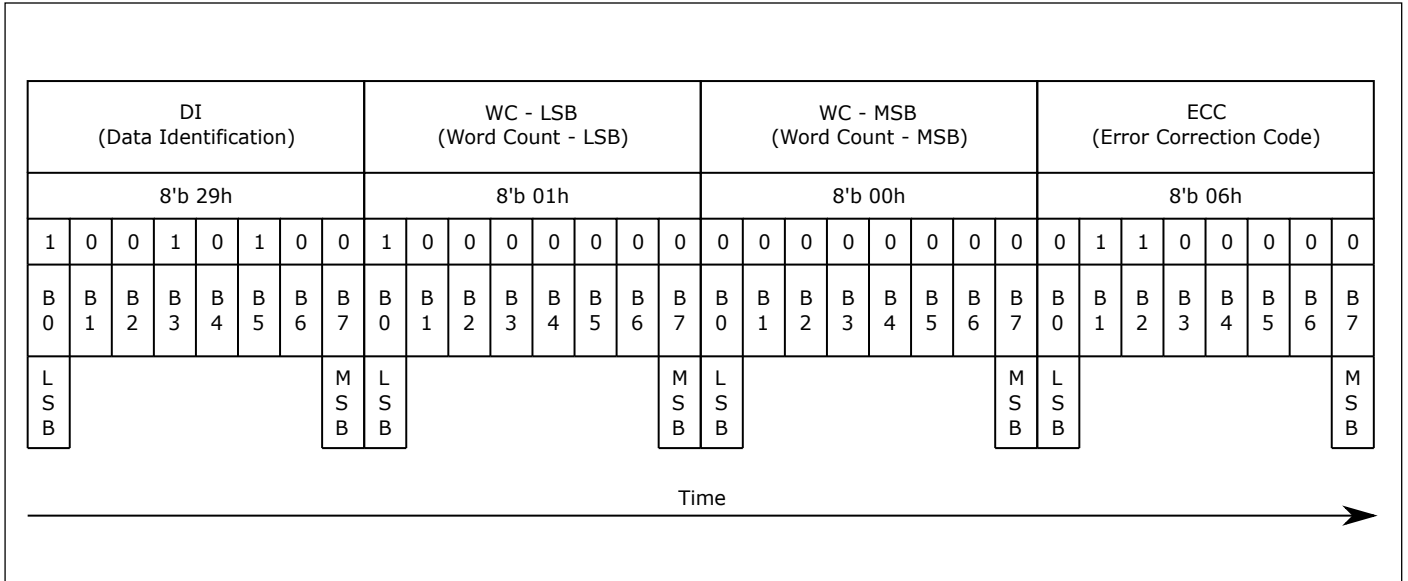
图 12.27: 数据包字节的位顺序
