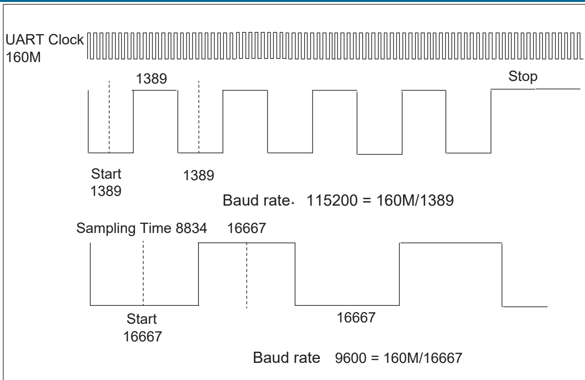
图 16.4: UART 采样波形图
