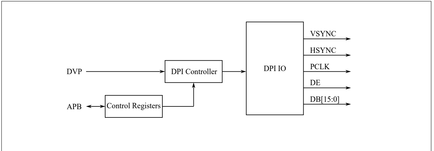
图 11.1: DPI 基本框图
