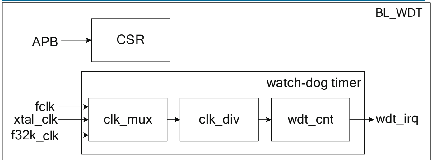
图 19.2: 看门狗定时器框图
