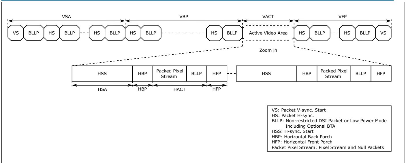
图 12.36: 突发模式时序图
