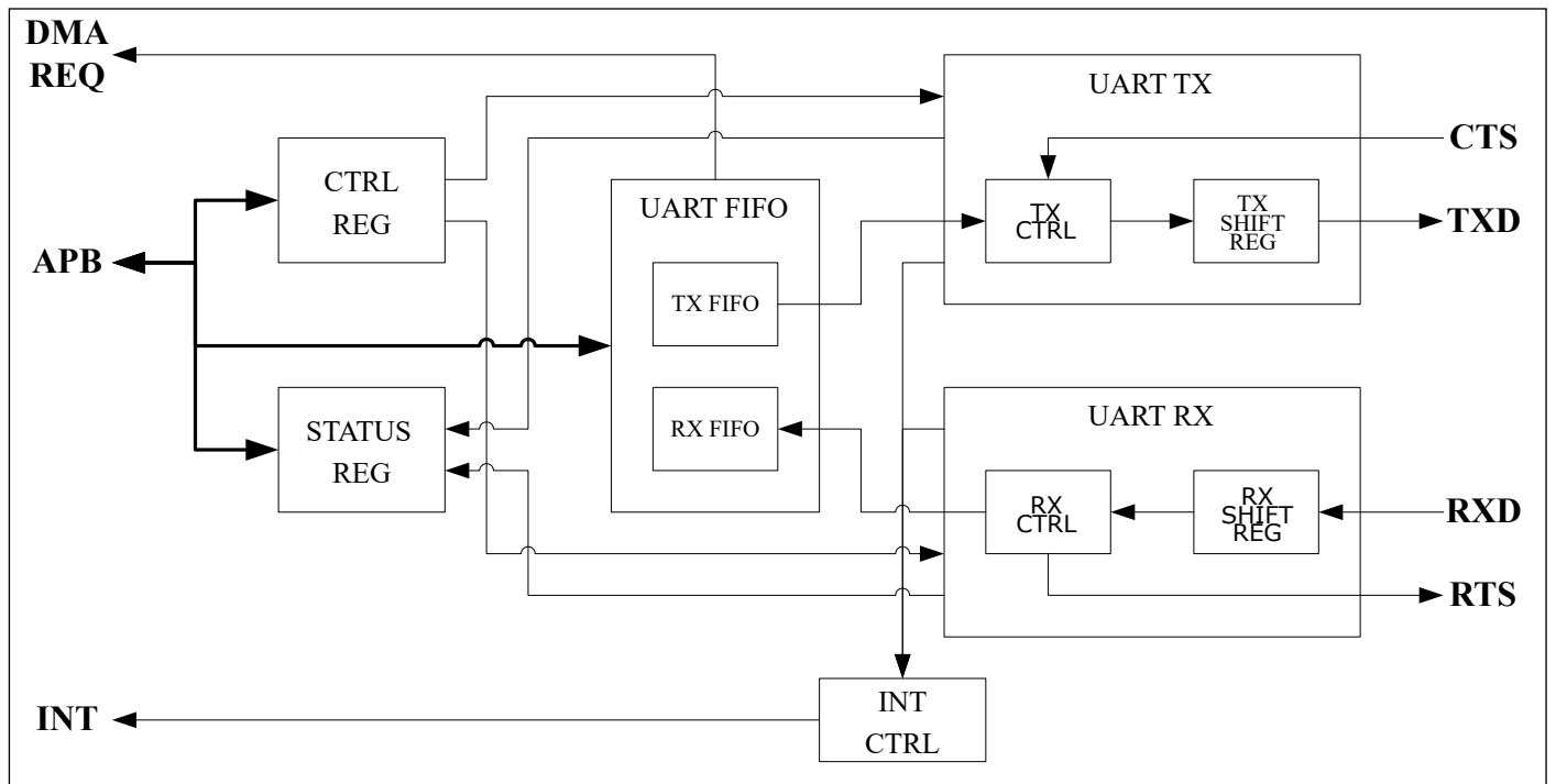
图 16.2: UART 架构图
