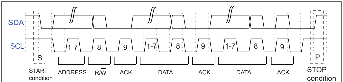
图 17.2: I2C 数据传输格式
