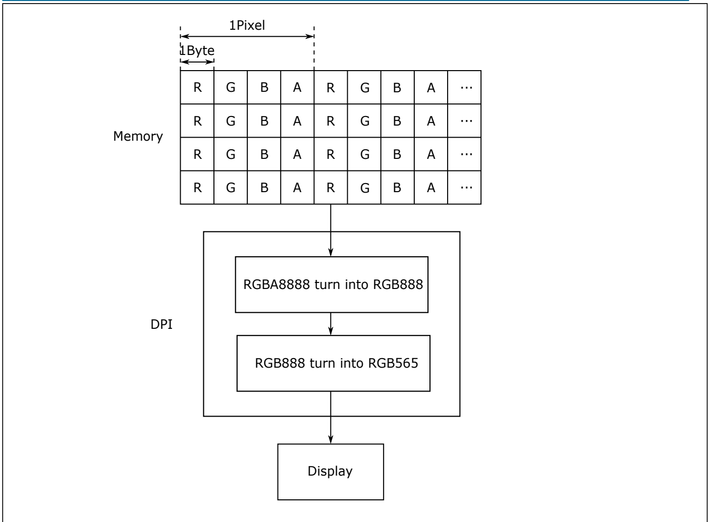
图 11.9: RGBA8888 处理过程
