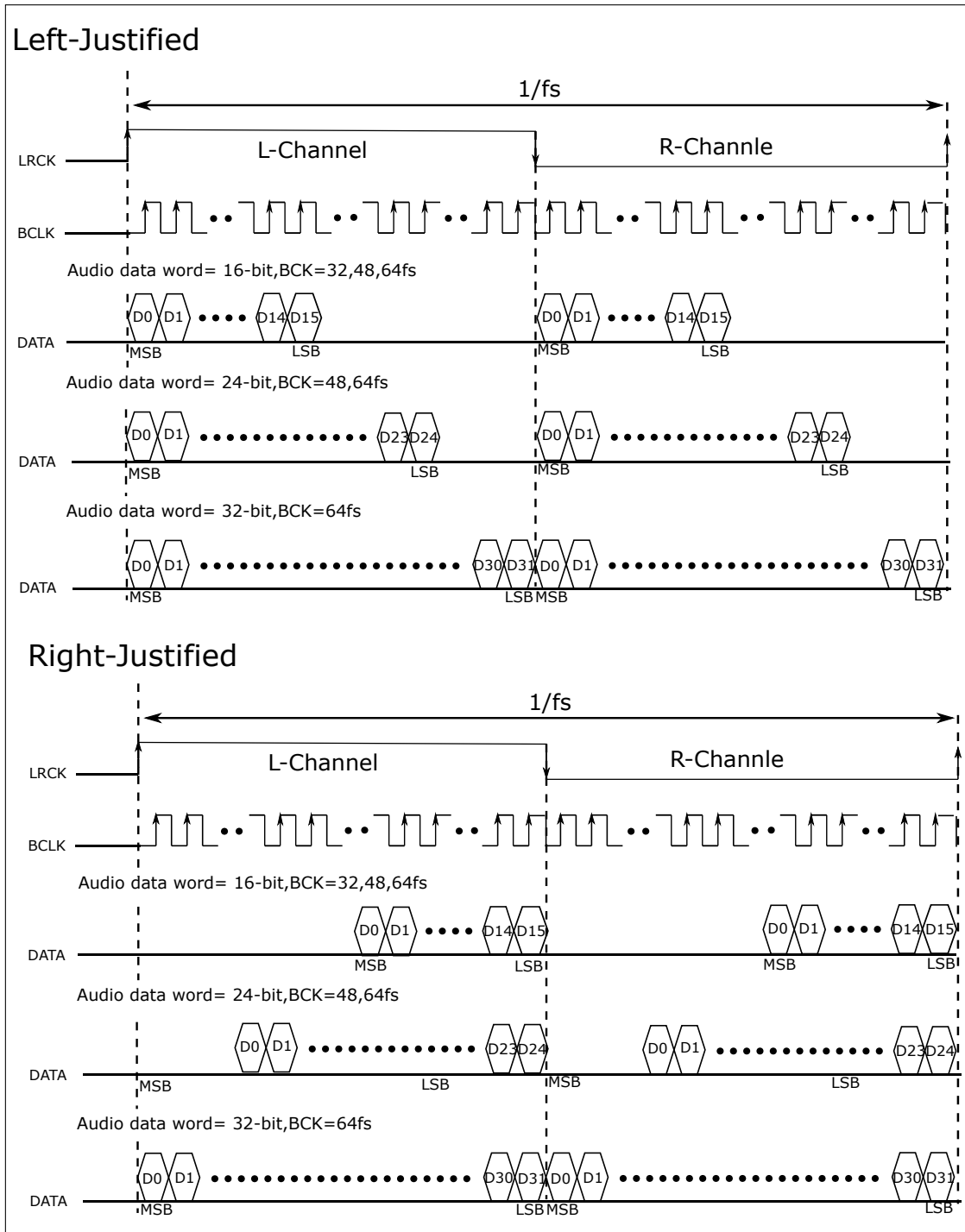
图 20.2: I2S 左对齐/右对齐数据格式
