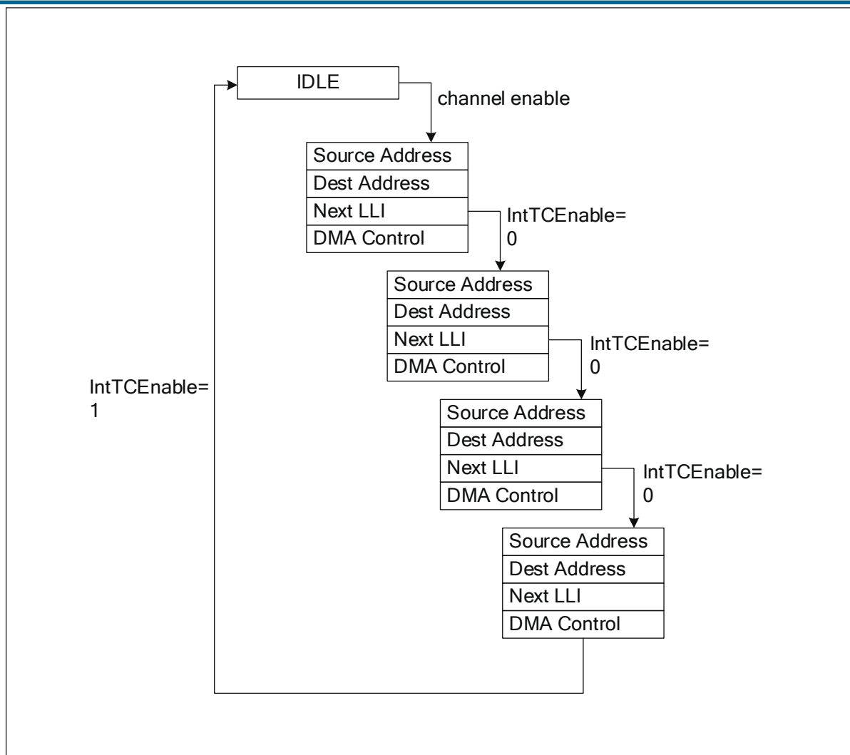
图 7.3: LLI 框架
