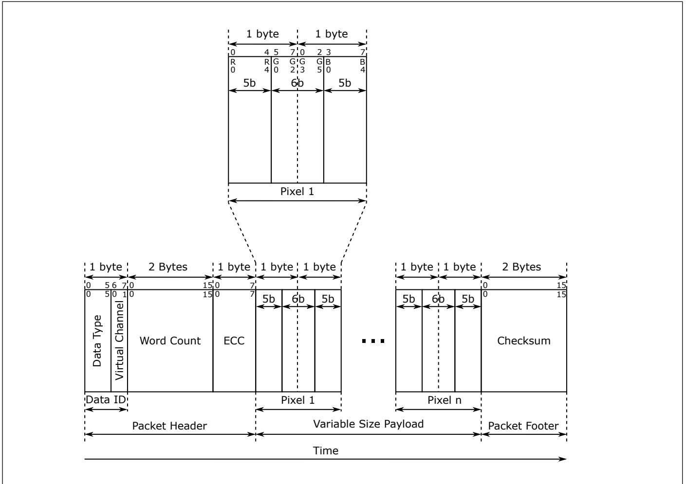
图 12.38: RGB565 像素格式
