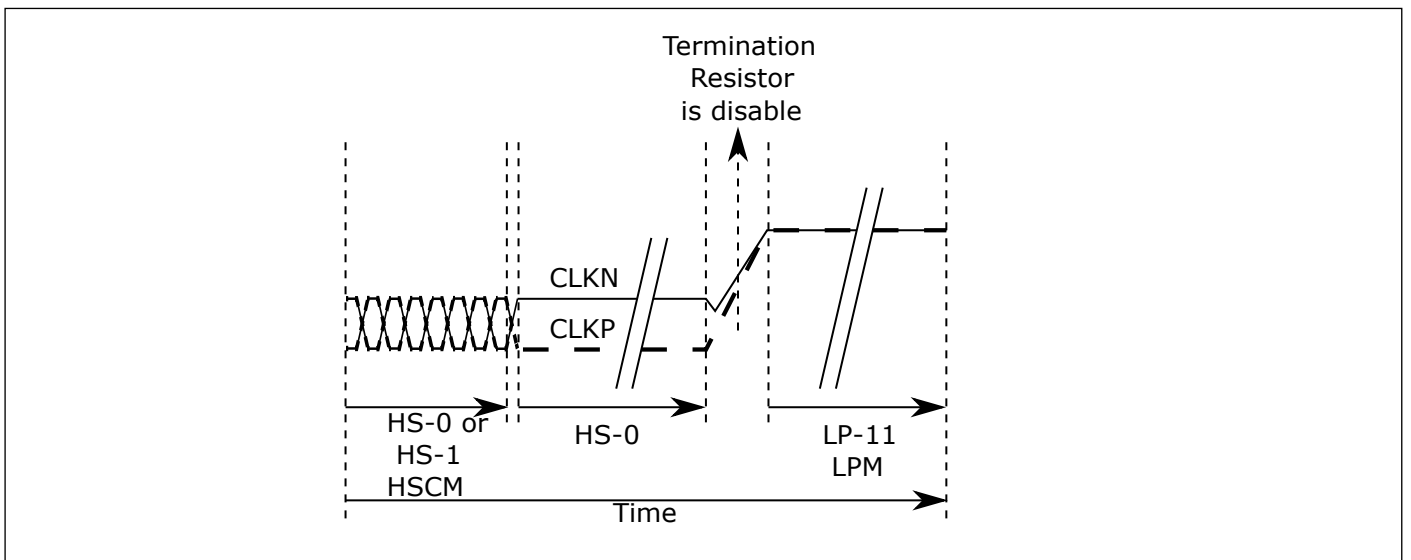
图 12.7: 由高速时钟模式进入低功耗模式
