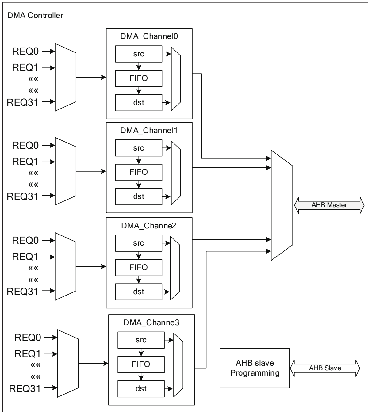
图 7.1: DMA 框图
