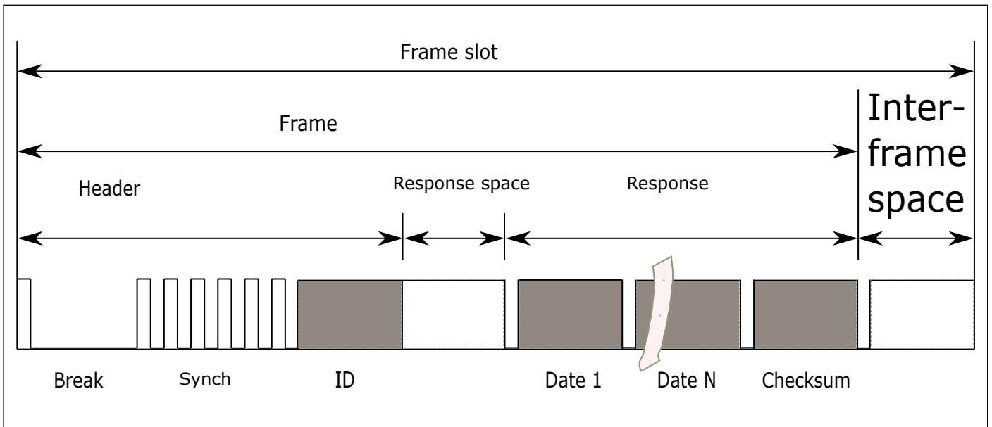
图 16.8: 一个典型的 LIN 帧
