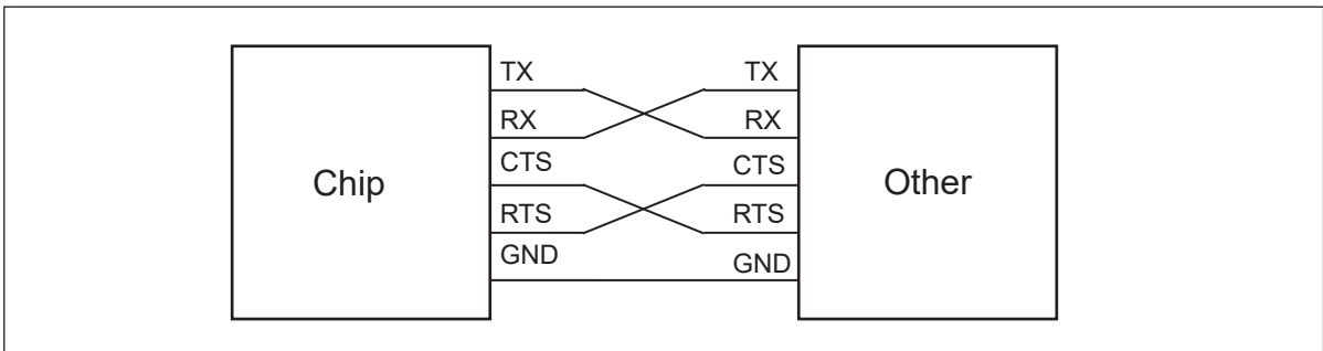
图 16.7: UART 硬件流控图
