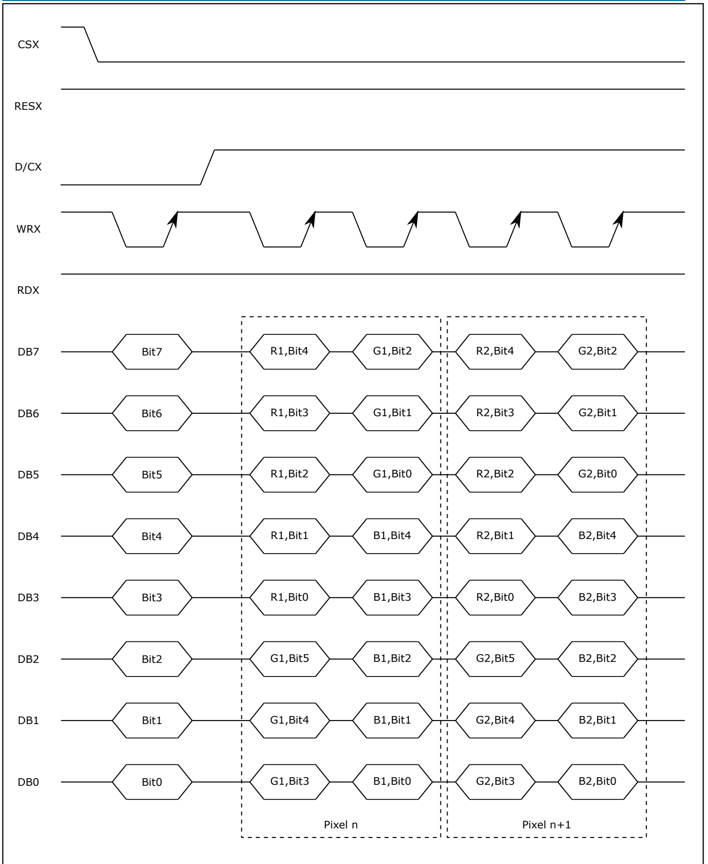
图 10.4: RGB565 输出
