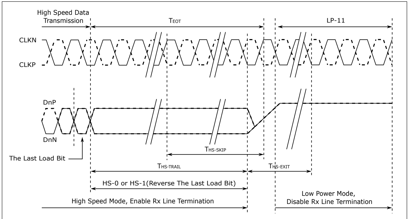
图 12.12: 高速数据传输退出序列
