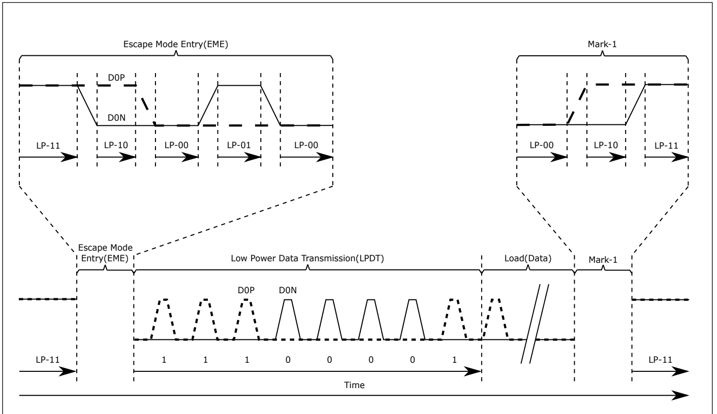
图 12.17: 低功耗数据传输序列
