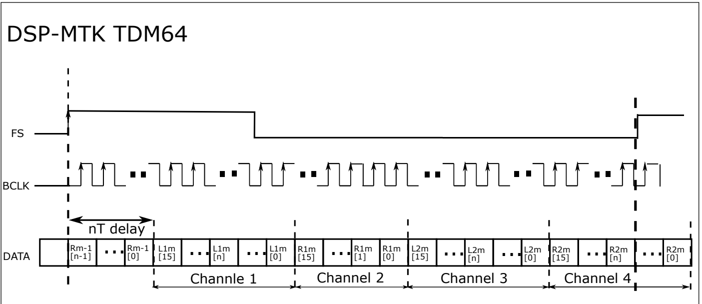
图 20.3: I2S TDM64 模式六通道录音
