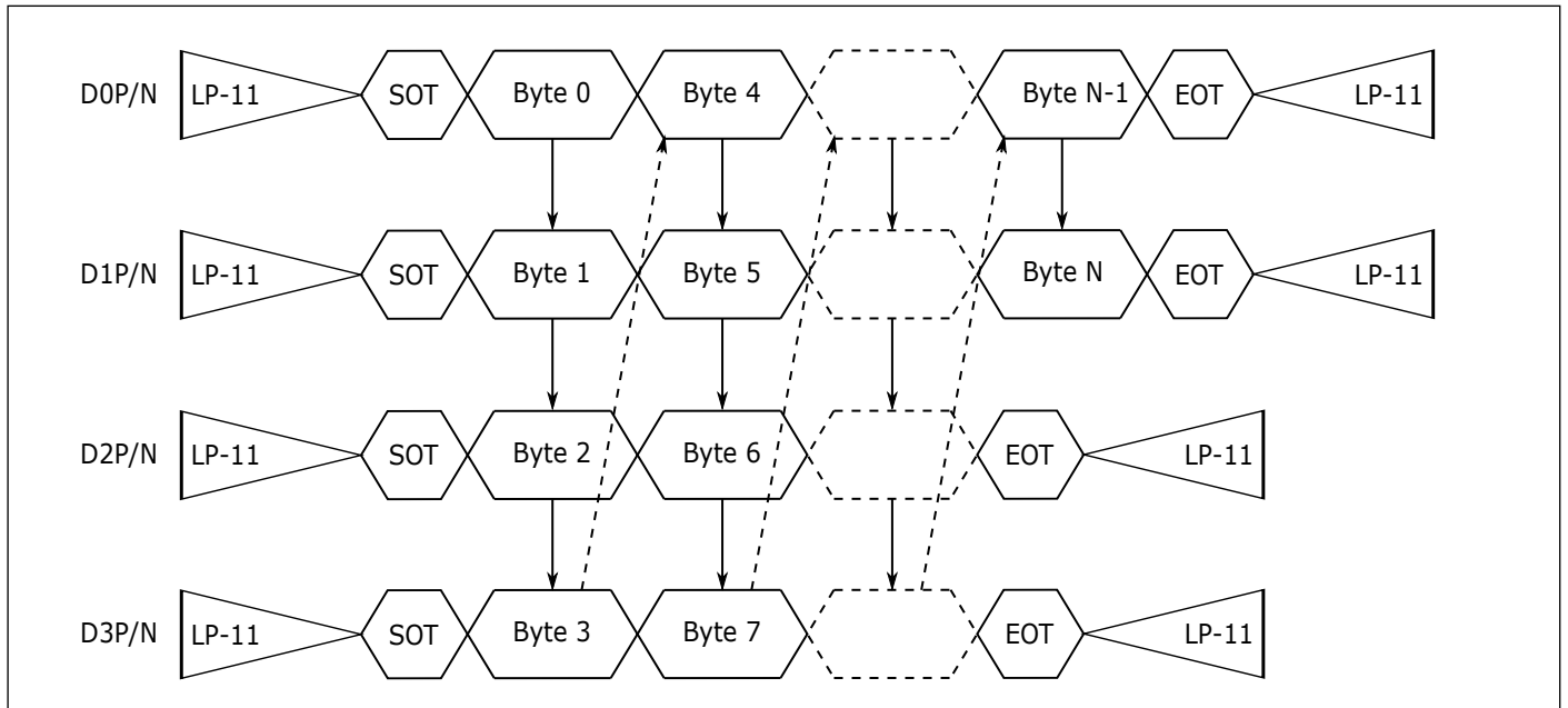
图 12.23: 非通道整数倍传输
