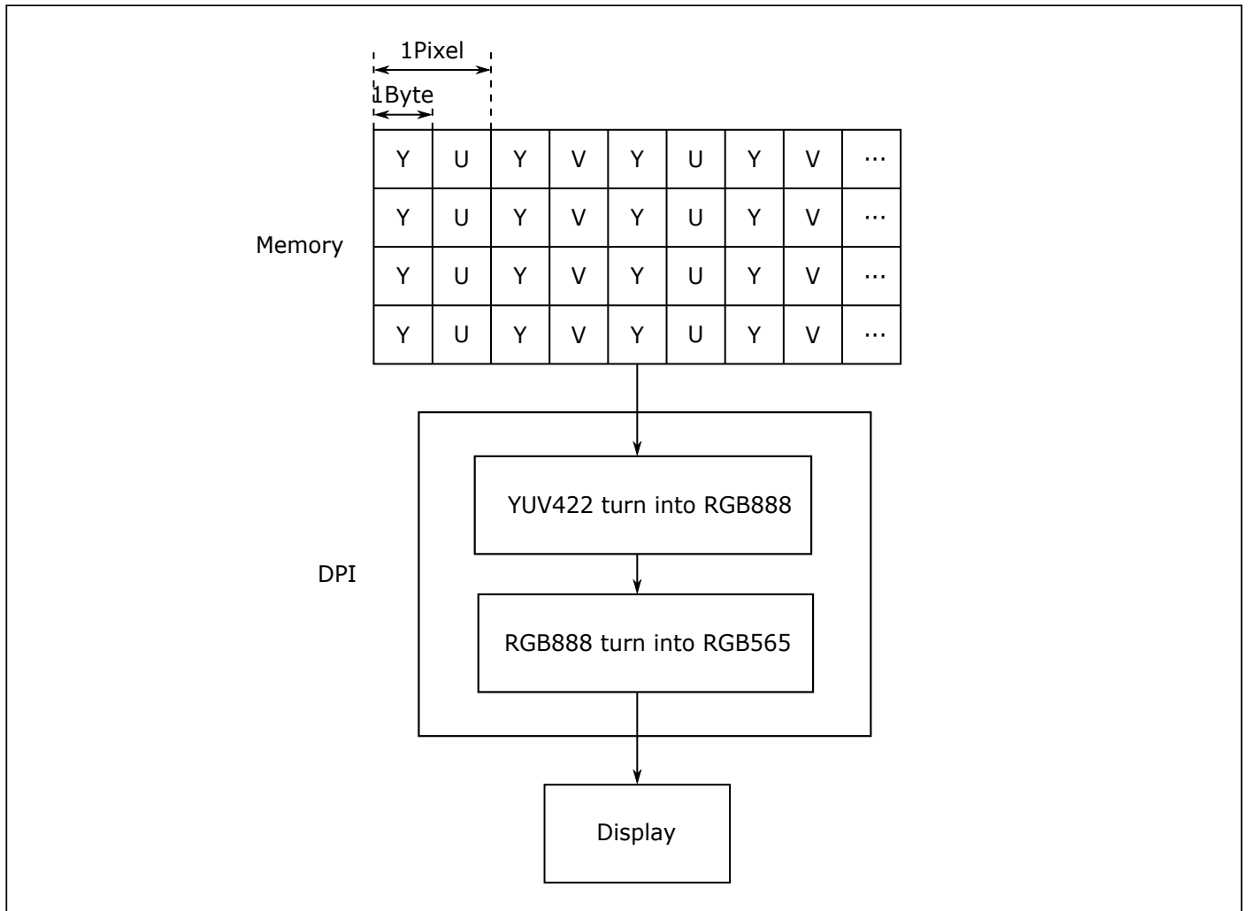
图 11.6: YUV422 处理过程
