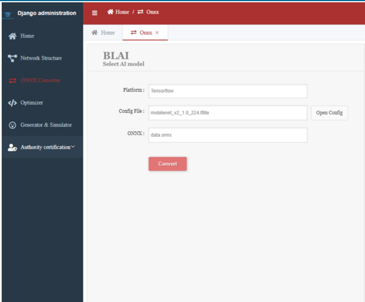
图 30.3: 转换界面
