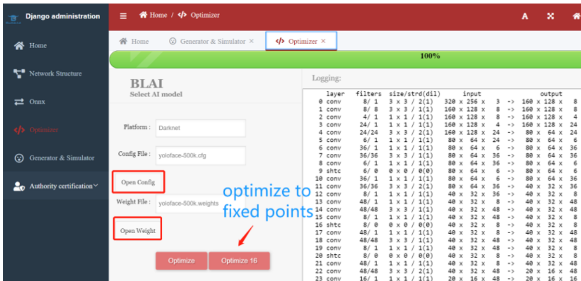
图 30.5: 优化器界面
