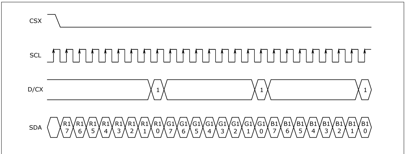
图 10.16: RGB888 输出
