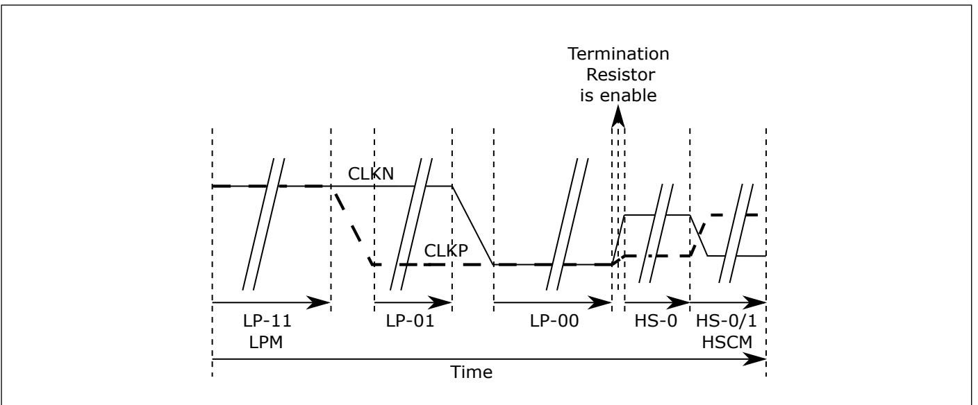
图 12.9: 由低功耗模式进入高速时钟模式
