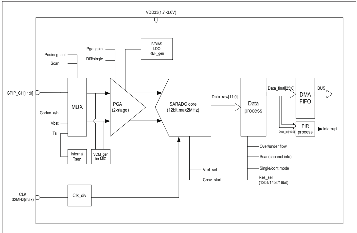
图 5.1: ADC 基本框图
