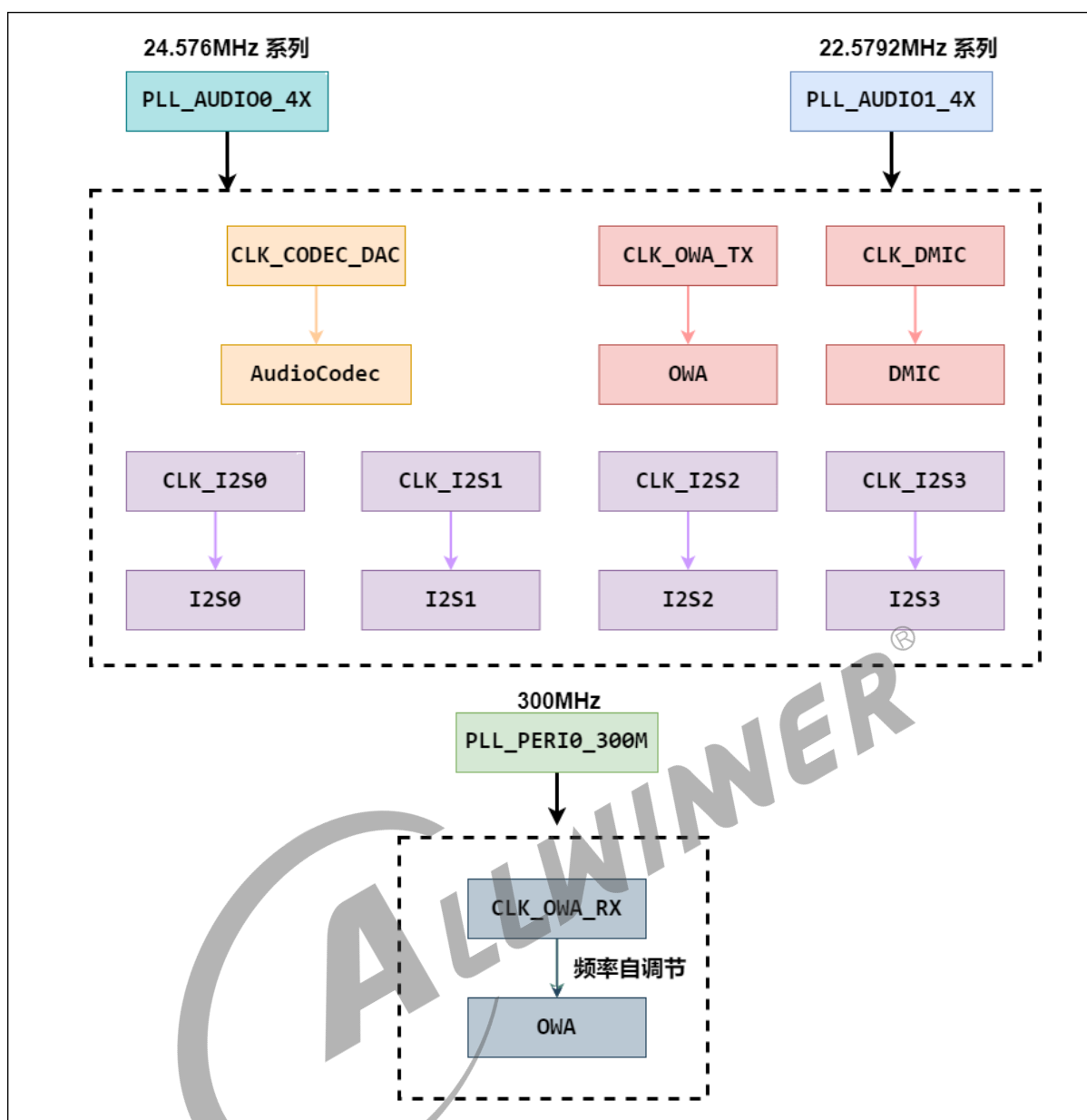
图 6-11: 时钟树 sun55iw6
