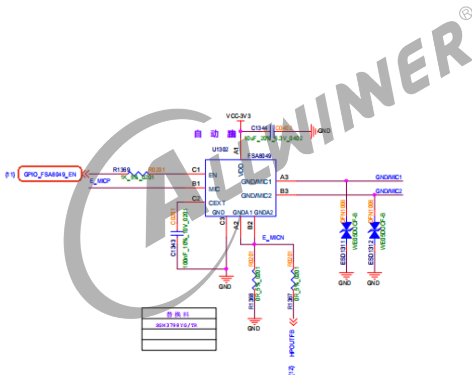
图 6-2: AI985 SCANP TYPE-C 耳机检测电路
