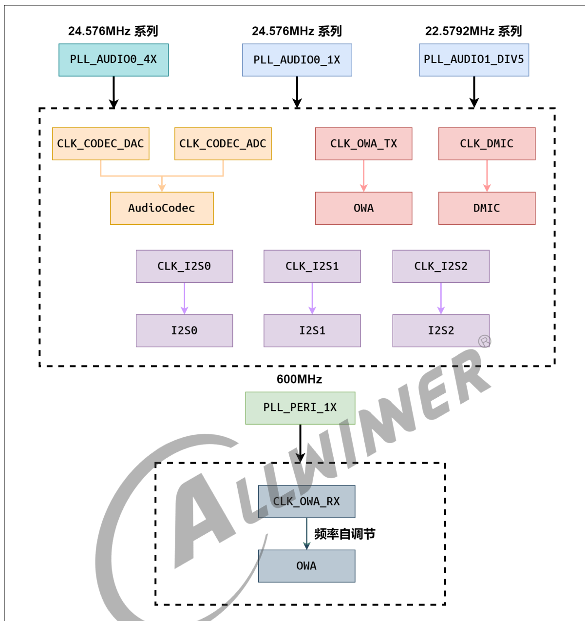
图 6-13: 时钟树 sun251iw1
