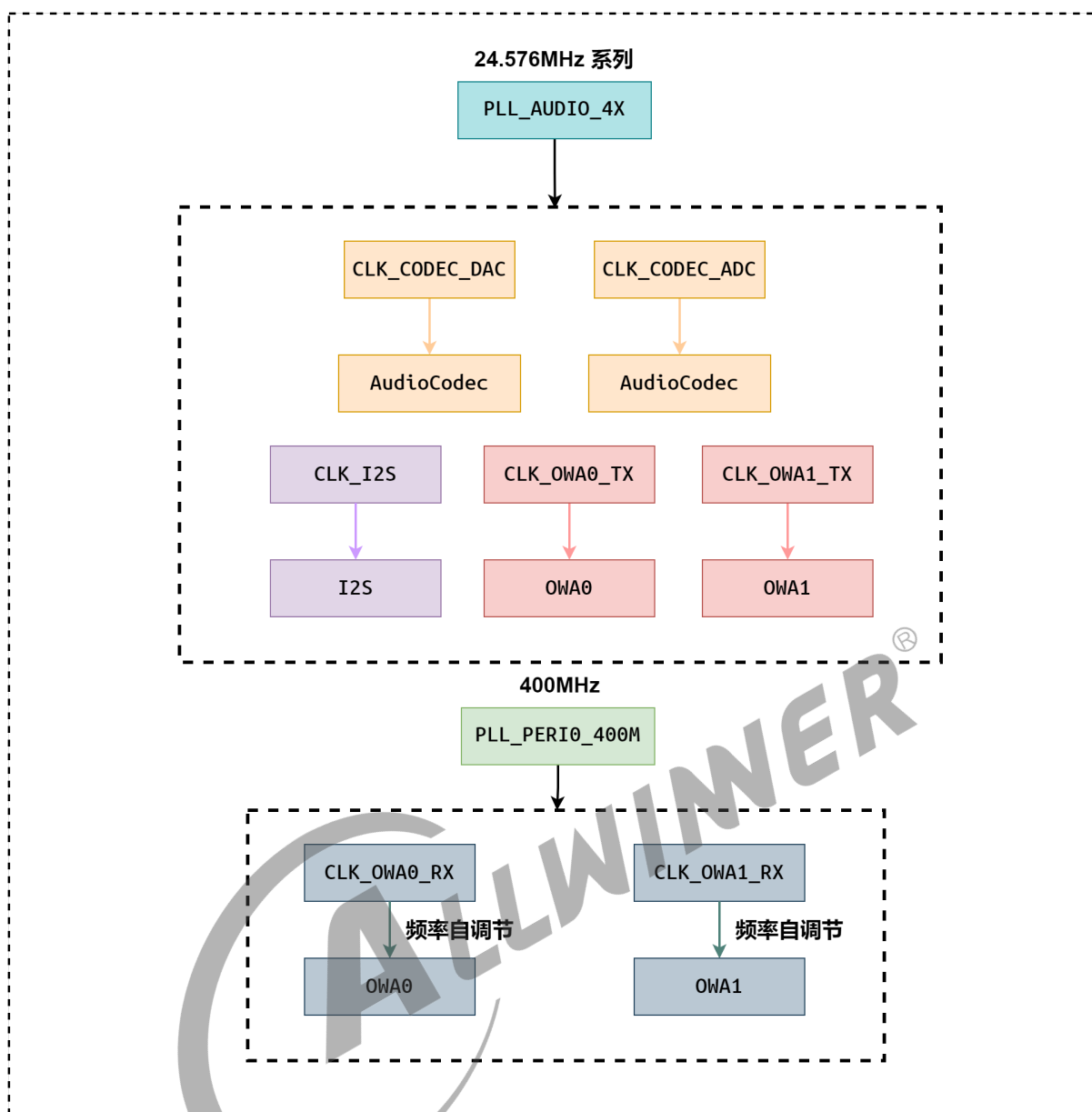
图 6-15: 时钟树 sun50iw15
