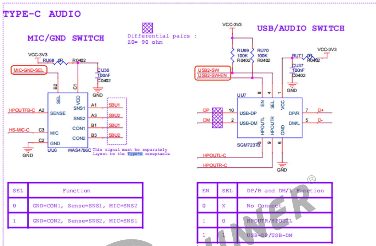
图 6-1: A523 EVB TYPE-C 耳机检测电路
