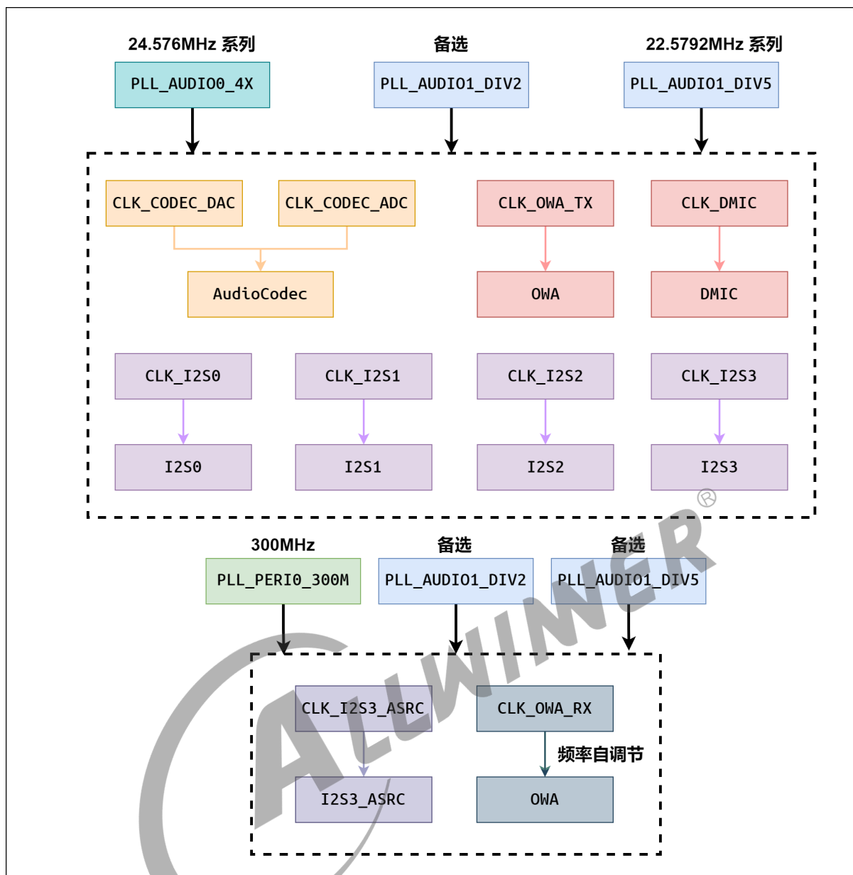
图 6-10: 时钟树 sun55iw3
