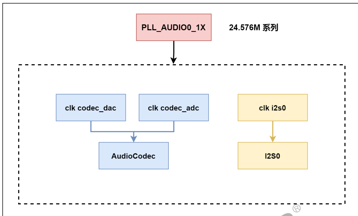
图 6-12: 时钟树 sun300iw1
