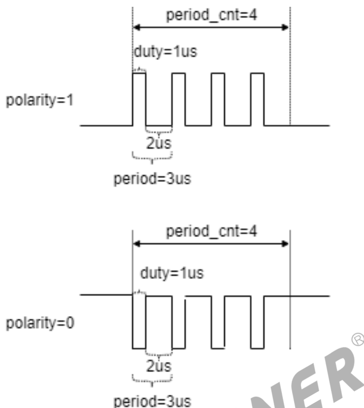
图 6-3: 脉冲使能方式示例
