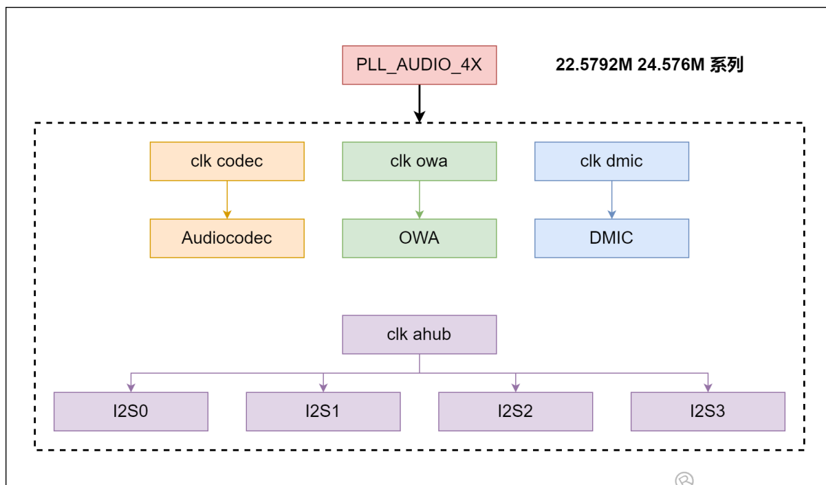
图 6-8: 时钟树 sun50iw9
