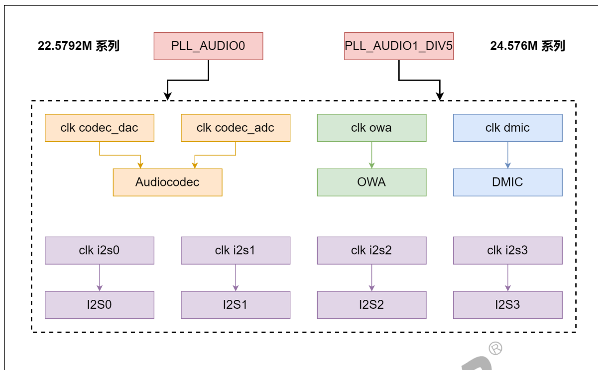
图 6-4: 时钟树 sun8iw20
