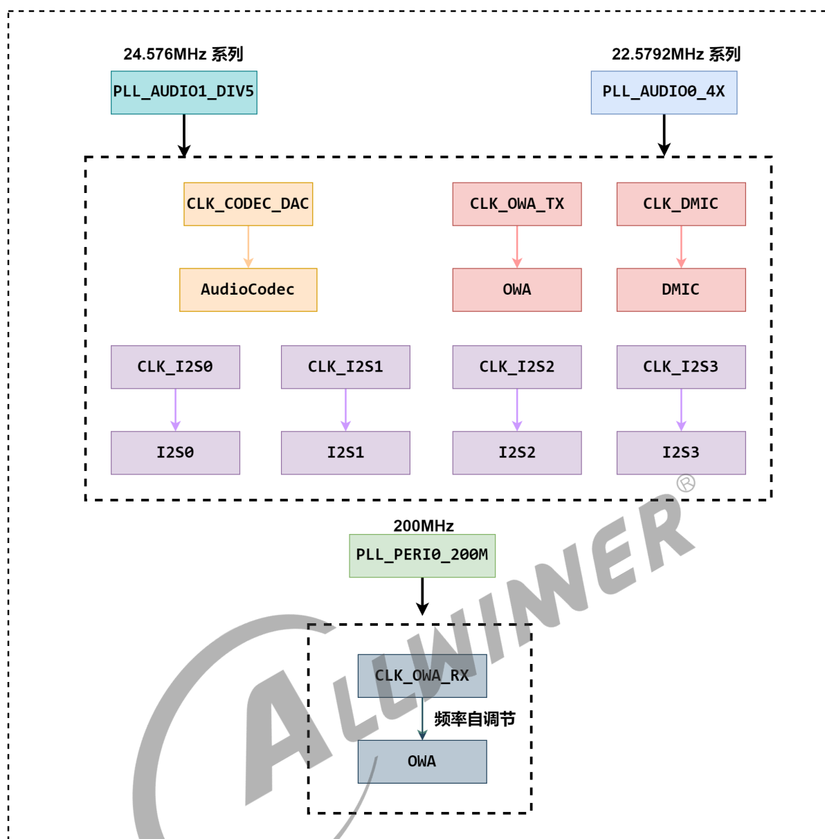
图 6-14: 时钟树 sun60iw2
