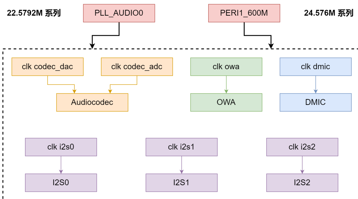
图 6-7: 时钟树 sun8iw22
