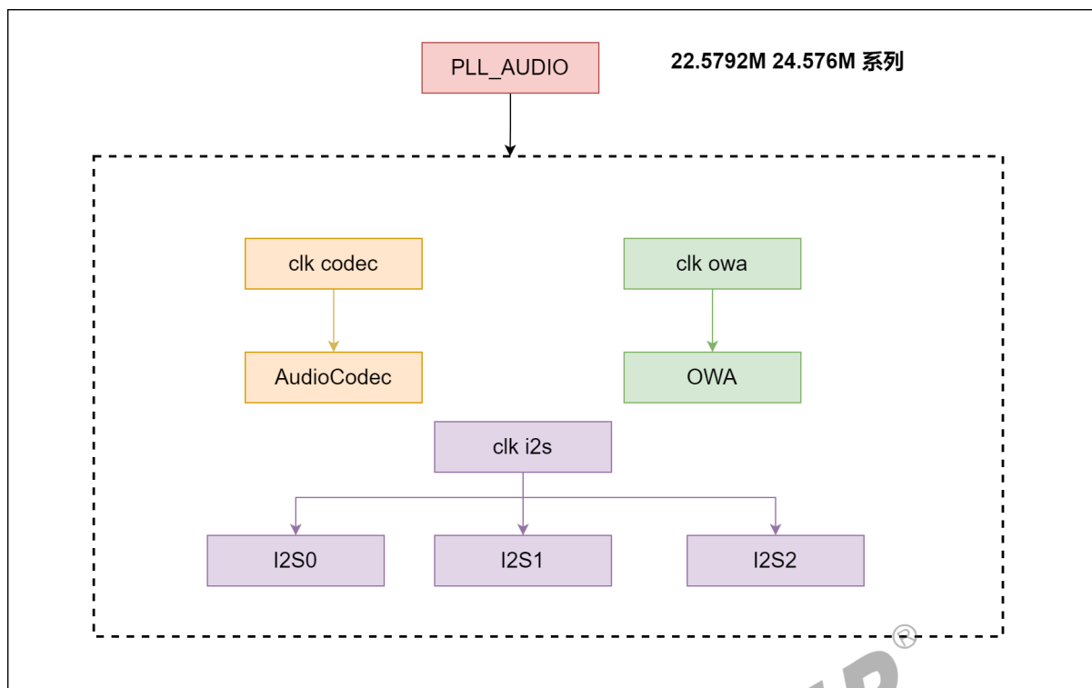
图 6-6: 时钟树 sun8iw11
