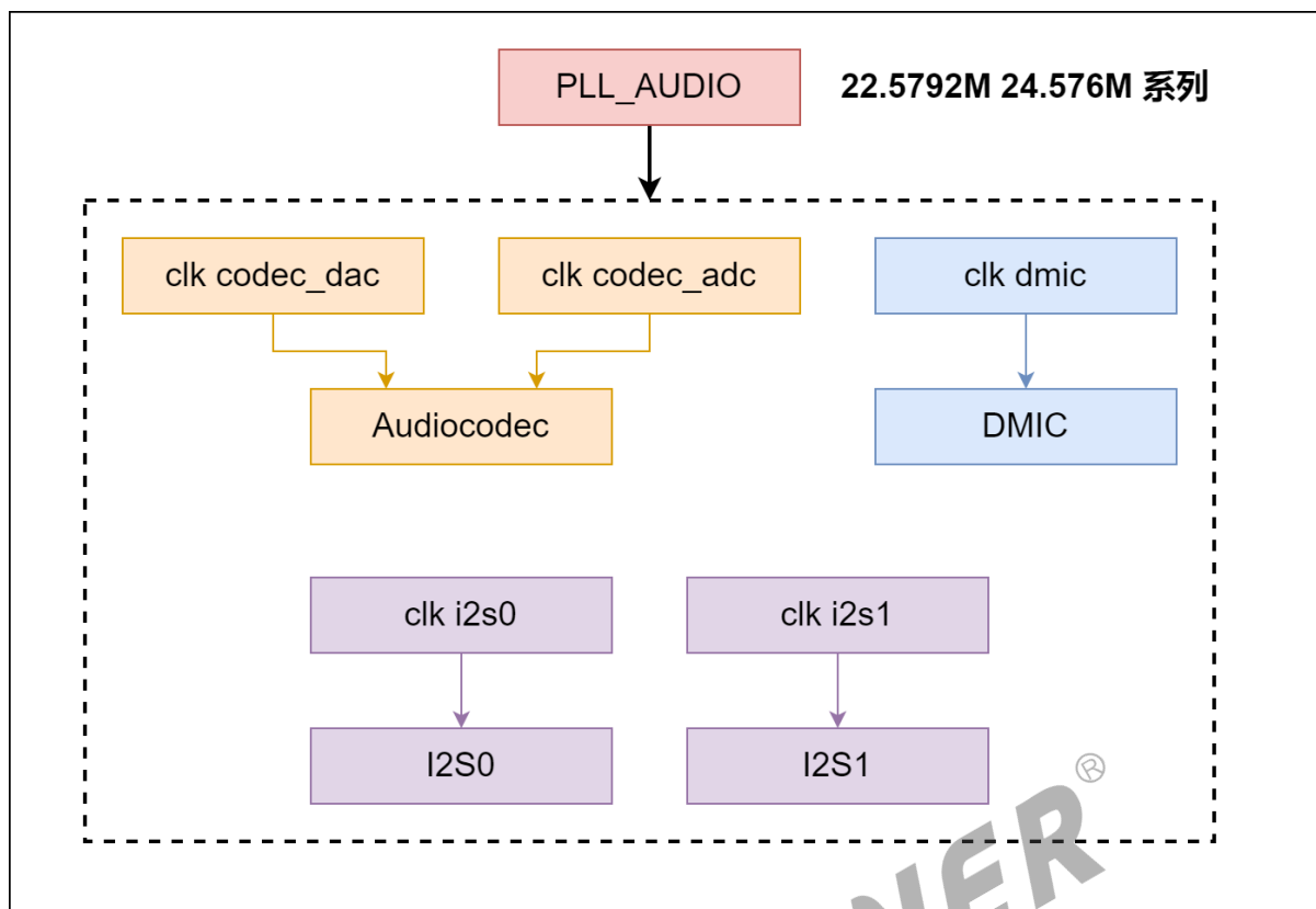
图 6-5: 时钟树 sun8iw21
