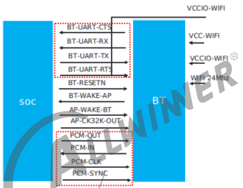
图 3-1: 主控与 BT 硬件连接简图
