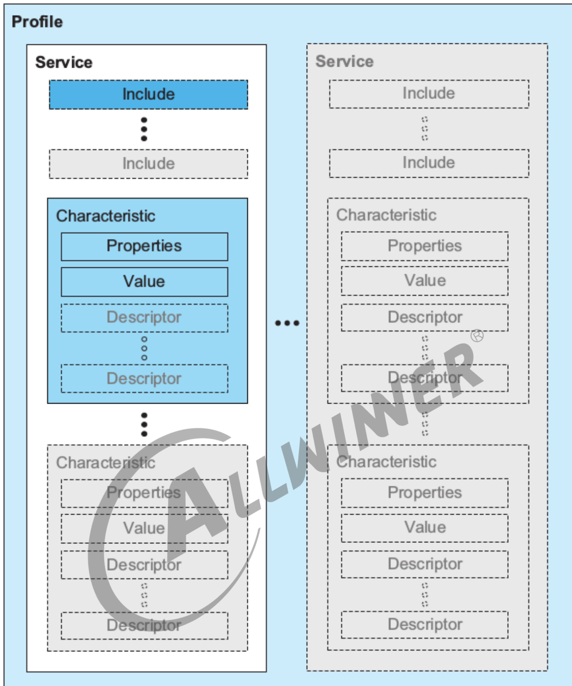
图 2-20: GATT Server 模型
