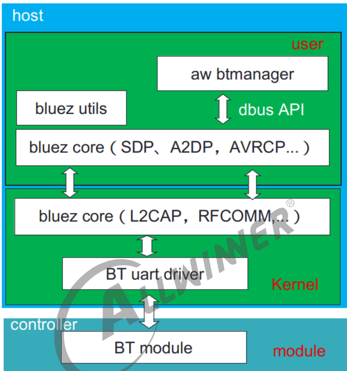
图 2-22: Tina 蓝牙协议栈结构图
