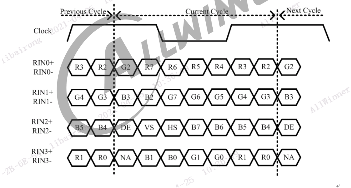
图 5-2: lvds mode ns
