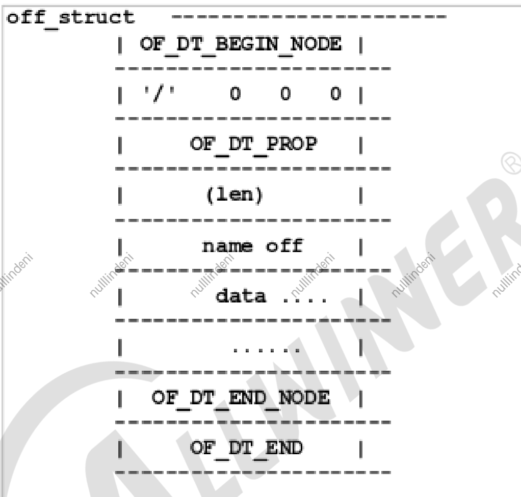
图 7: device-tree 的 structure 结构
