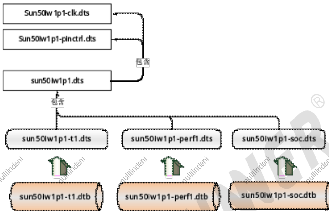
图 9: 不存在 sysconfig 的配置结构
