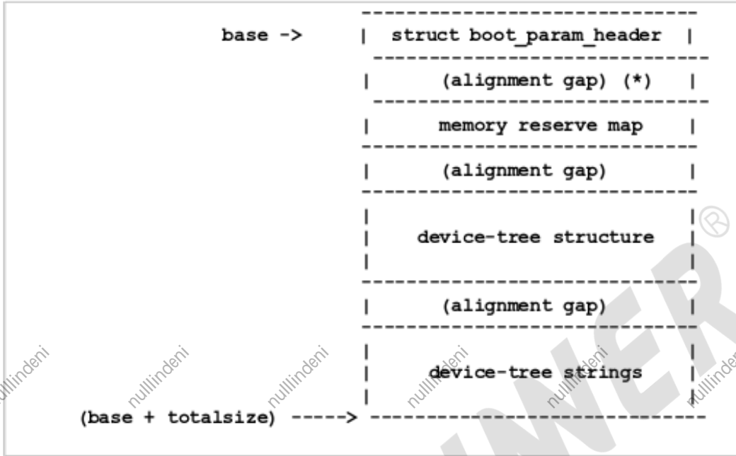
图 6: dtb 内存布局
