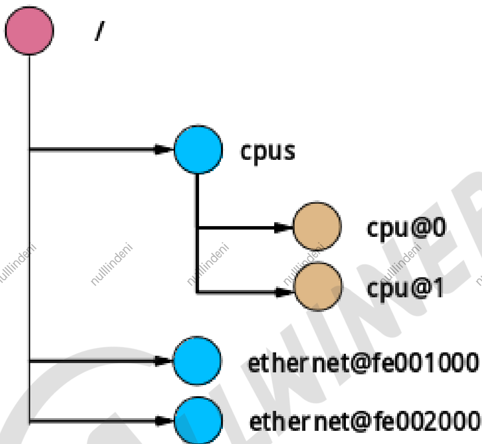
图 3: 节点名称规范示例
