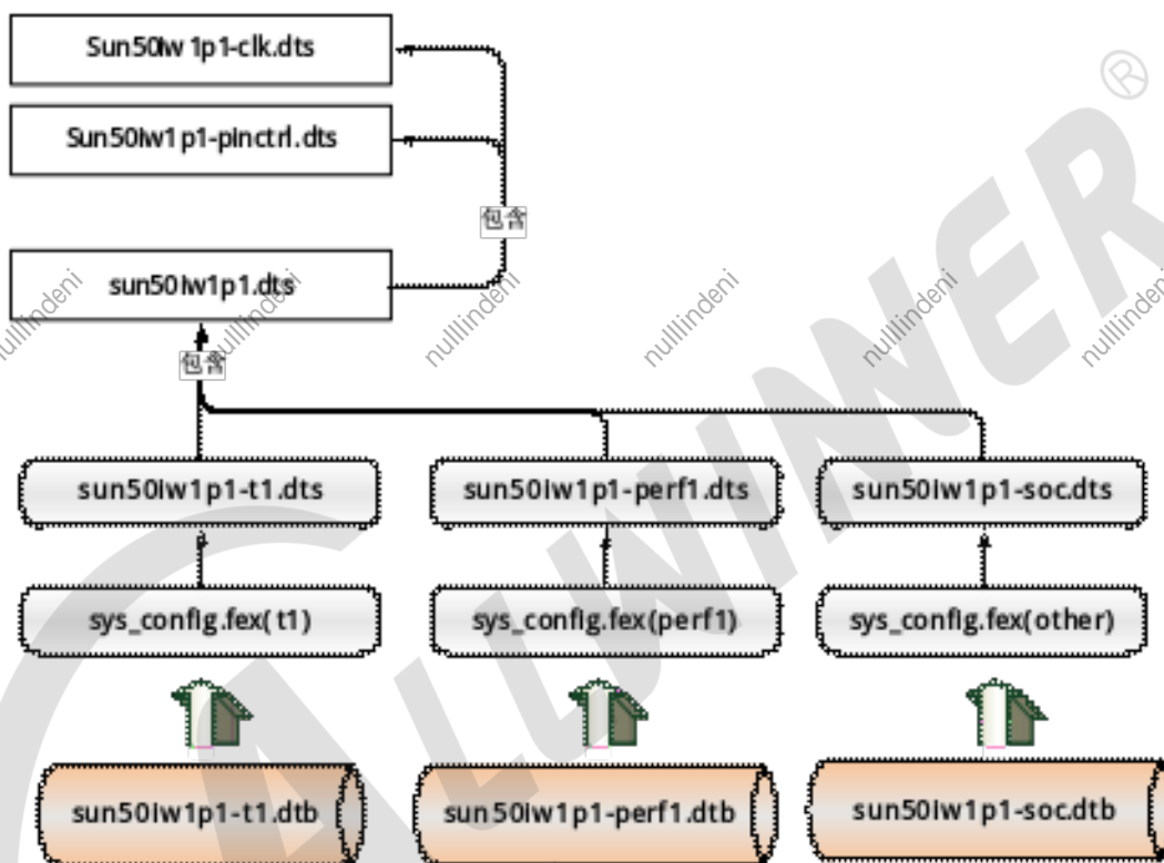
图 10: 存在 sysconfig 的配置结构
