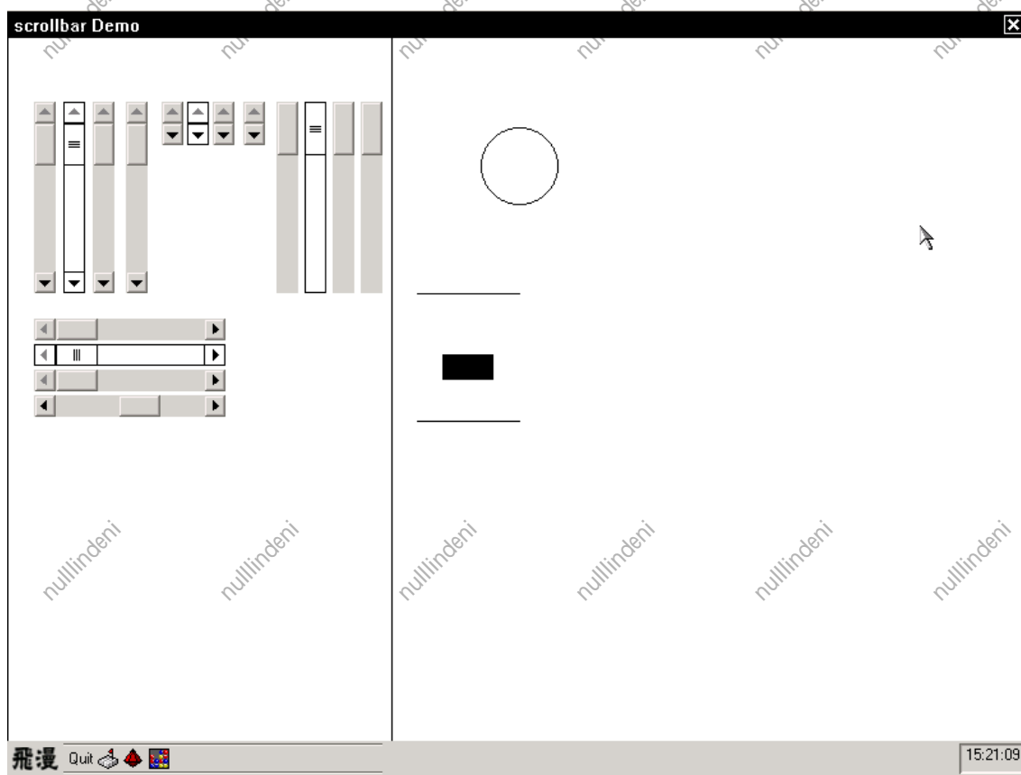
图 39.3 滚动条控件
