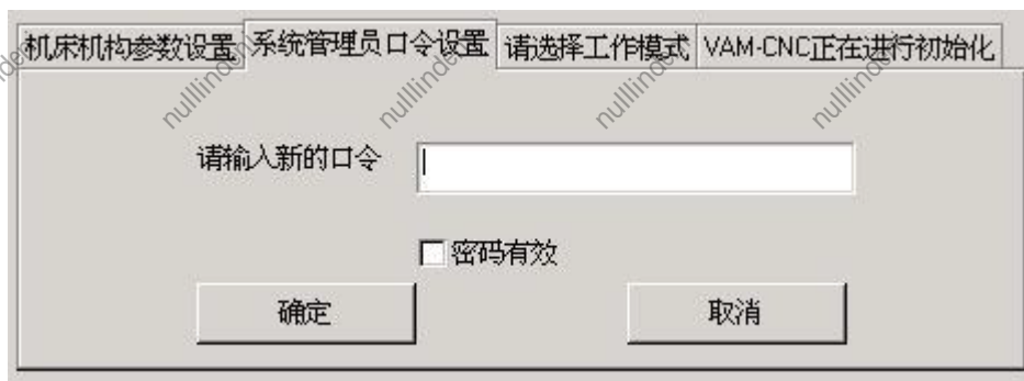
图 28.1 属性页控件
