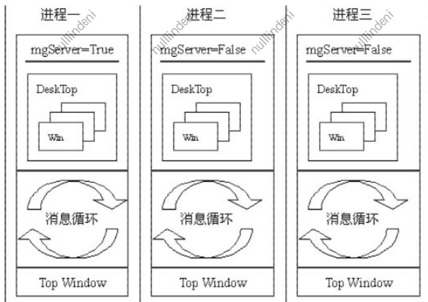
图 16.1 多进程模型
