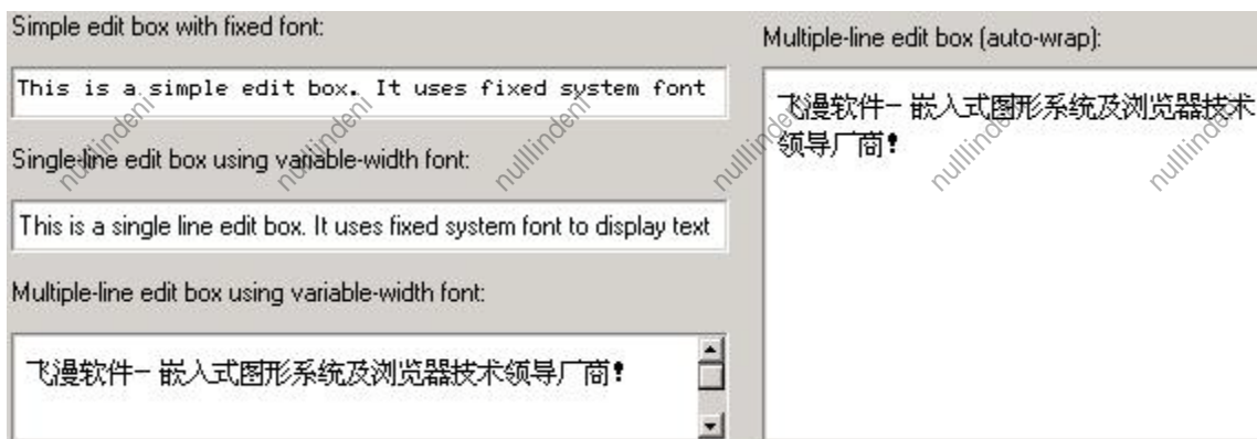
图 22.1 MiniGUI 编辑框
