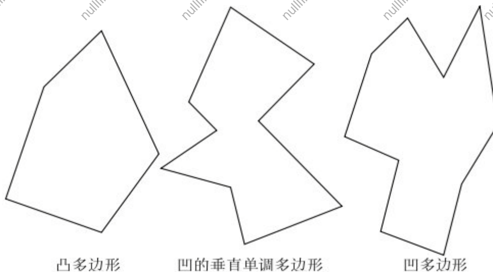
图 15.1 各种多边形
