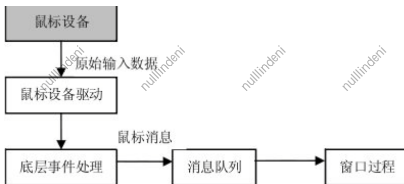
图 9.2 MiniGUI 中的鼠标输入
