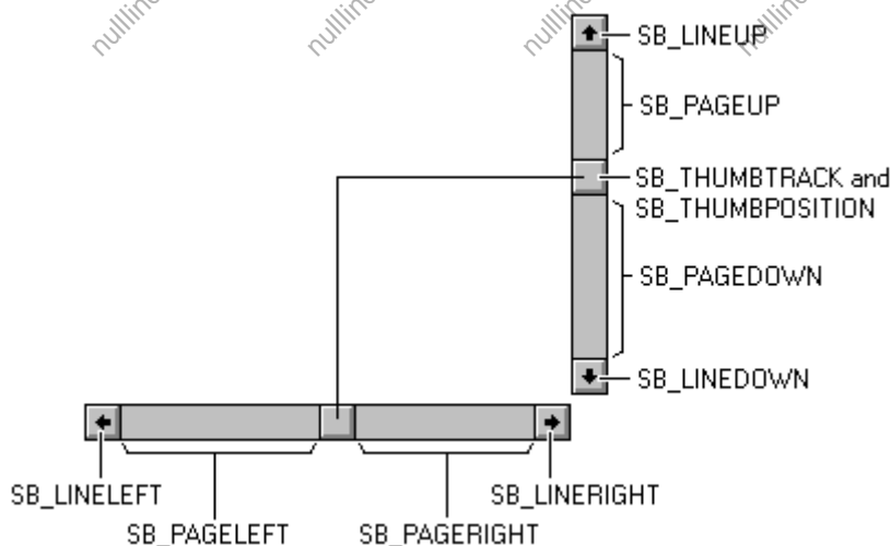
图 39.2 鼠标触发的通知消息
