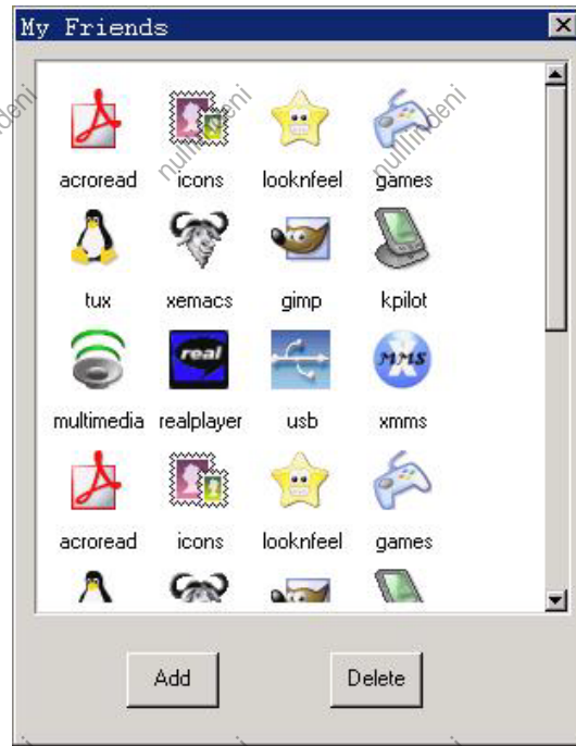
图 38.1 图标型控件
