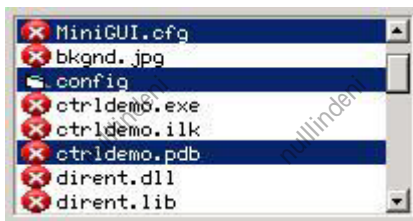
图 21.2 多选列表框
