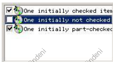
图 21.3 高级列表框
