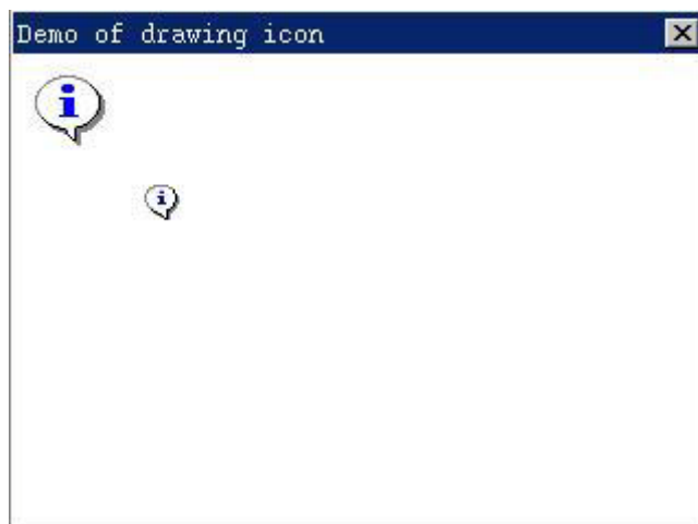
图 10.1 图标的绘制
