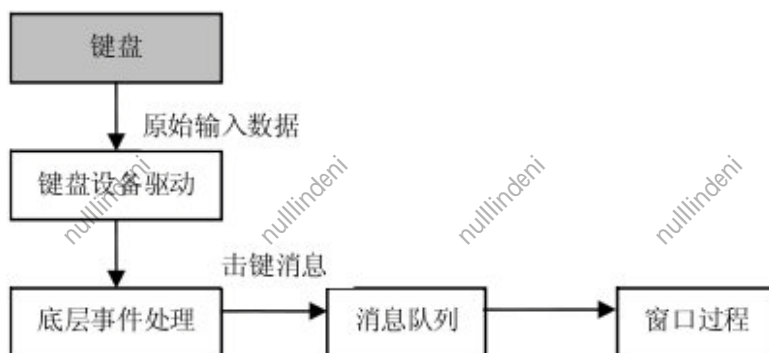
图 9.1 MiniGUI 中的键盘输入
